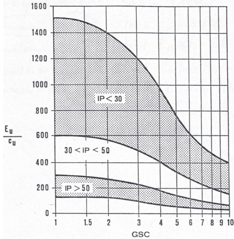
Figura 6.3 - Modulo di Young operativo in condizioni non drenate (Duncan e Buchignami, 1976)
