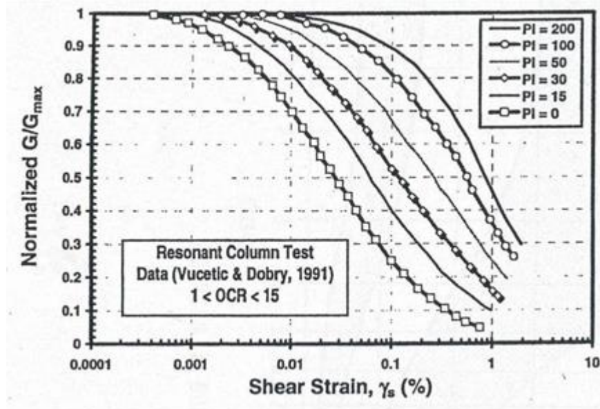
Figura 6.2 - Curve sperimentali del rapporto G/G_{max} da prove di colonna risonante ciclica (Vucetic & Dobry, 1991)
