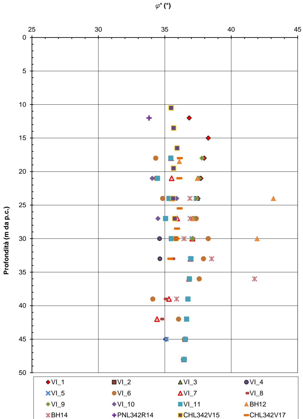
Figura 8-43 - Unità 4 - Stima angolo di attrito da prove SPT
