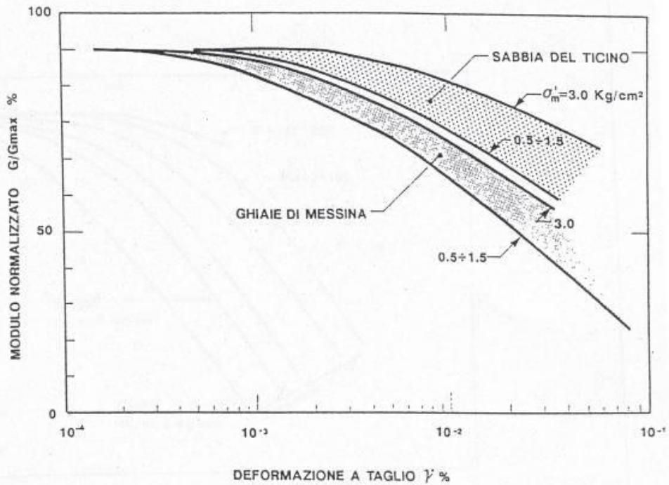
Figura 6.4 - Degrado del modulo G per terreni incoerenti
