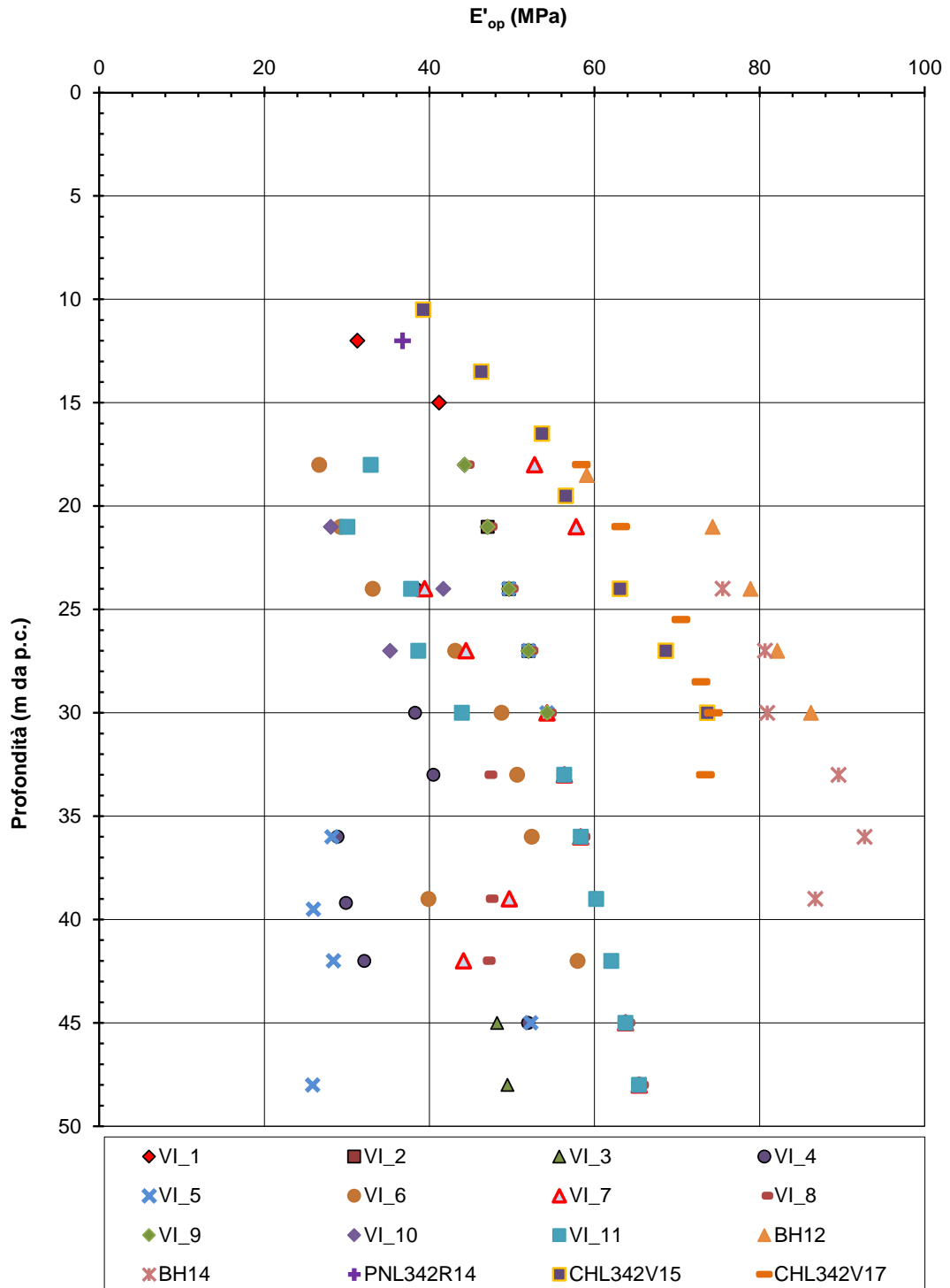
Figura 8-46 - Unità 4 - Stima modulo di Young operativo da prove SPT
