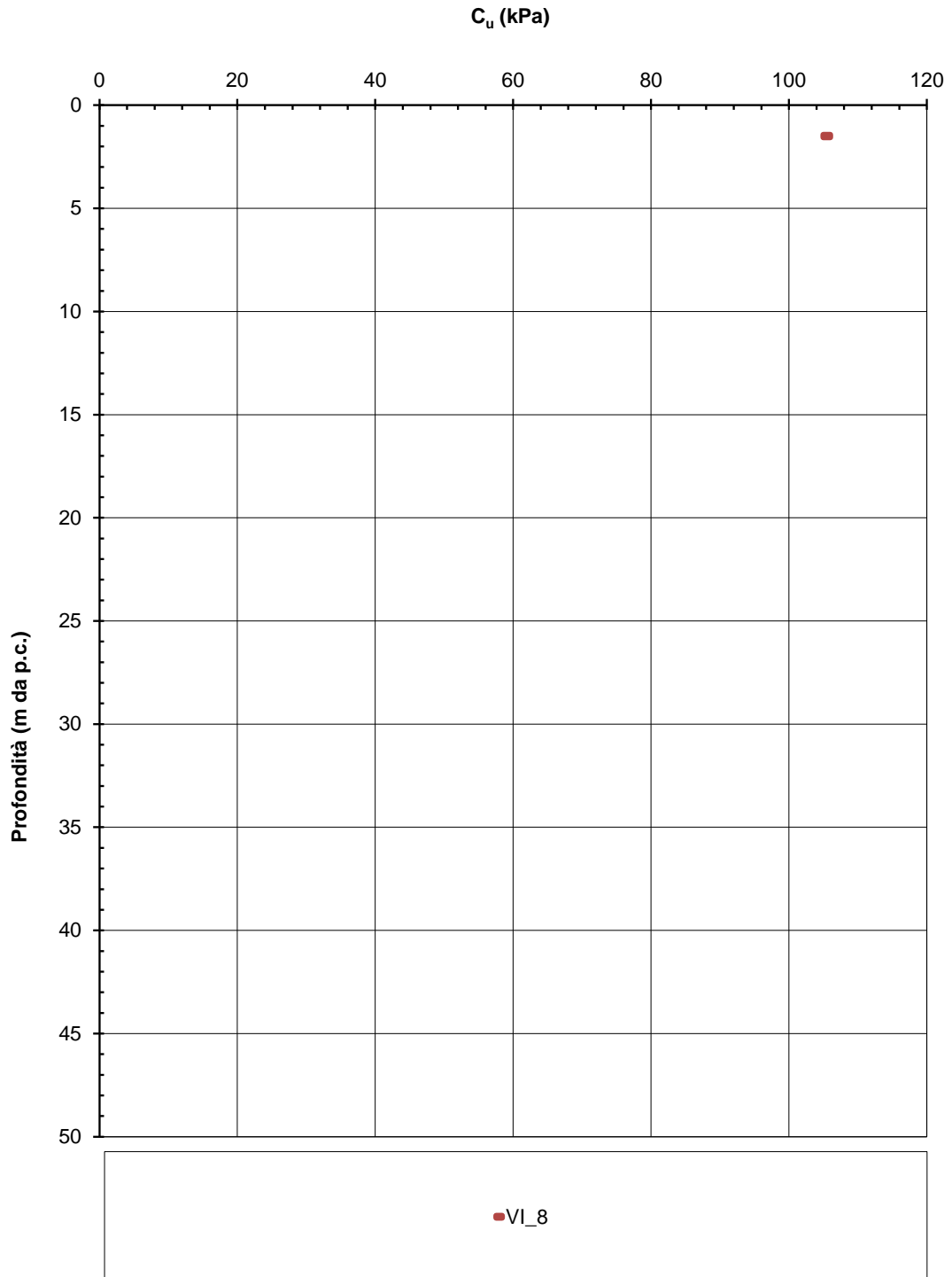
Figura 8-9 - Unità 1 - Stima coesione non drenata c_u da prove SPT
