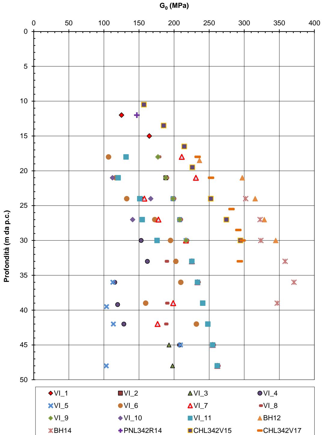
Figura 8-44 - Unità 4 - Stima modulo di taglio a piccole deformazioni da prove SPT
