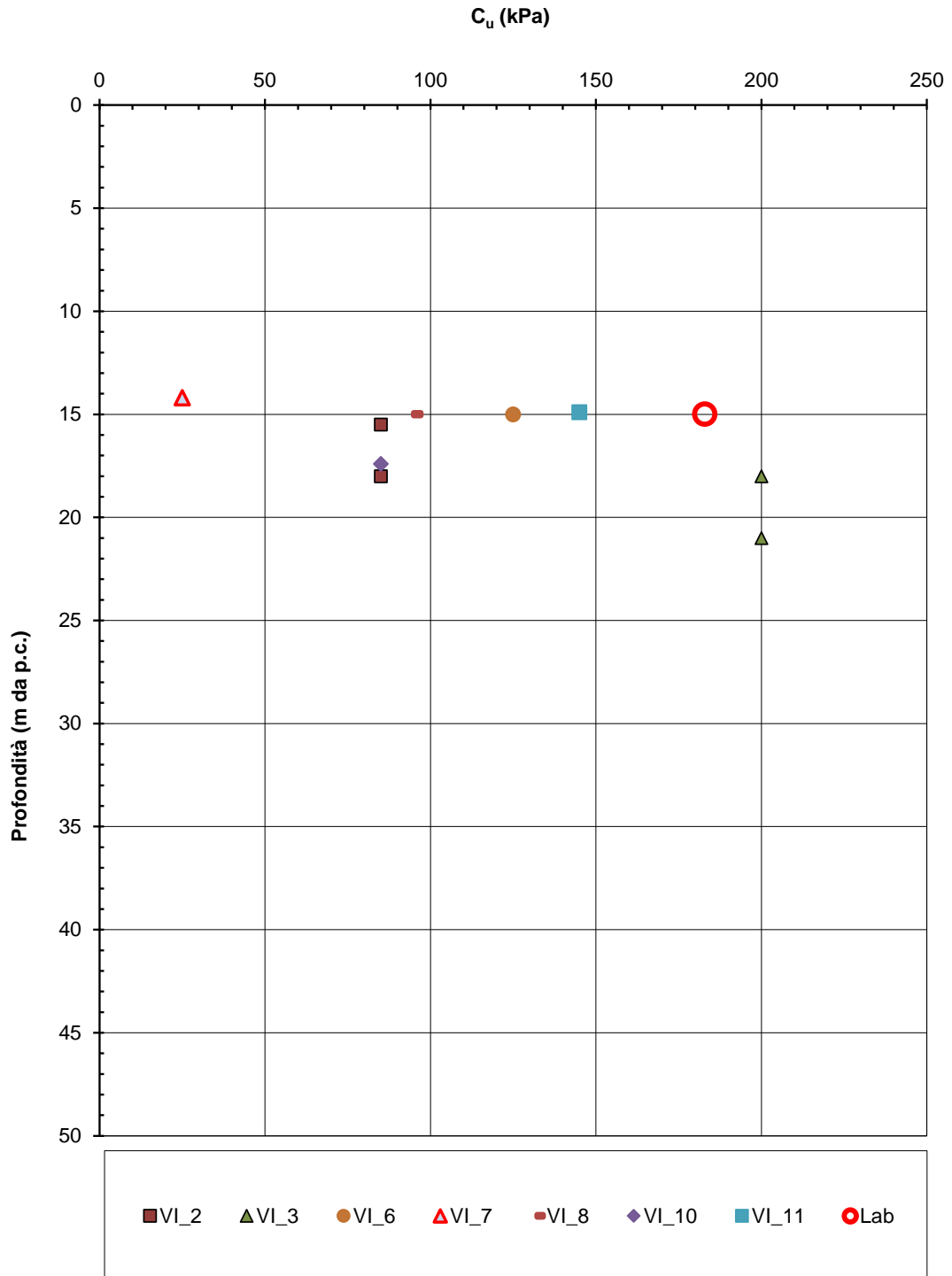
Figura 8-32 - Unità 3 - Stima coesione non drenata c_u da prove SPT e di laboratorio
