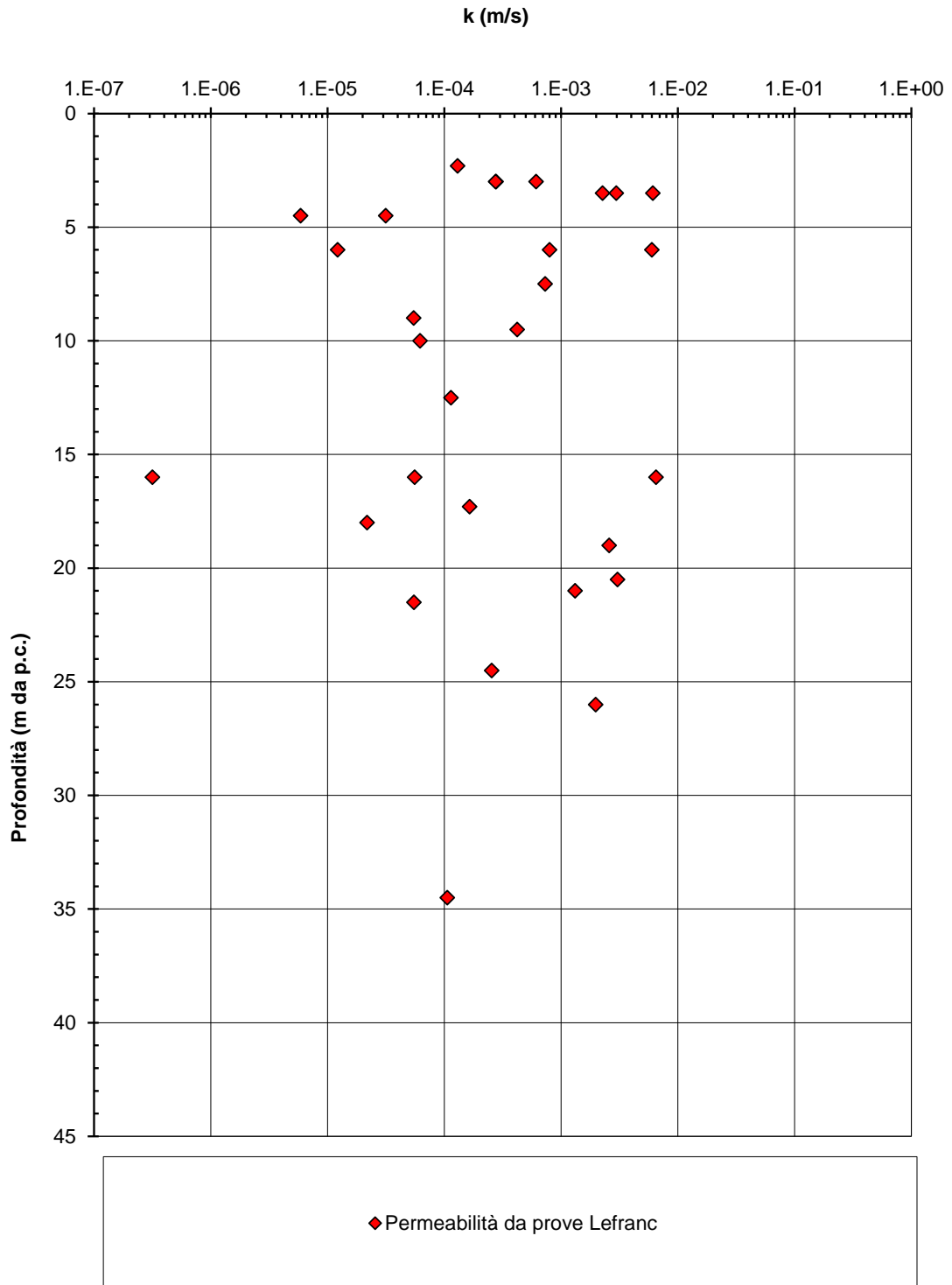
Figura 8.47 – Permeabilità k_h da prove Lefranc
