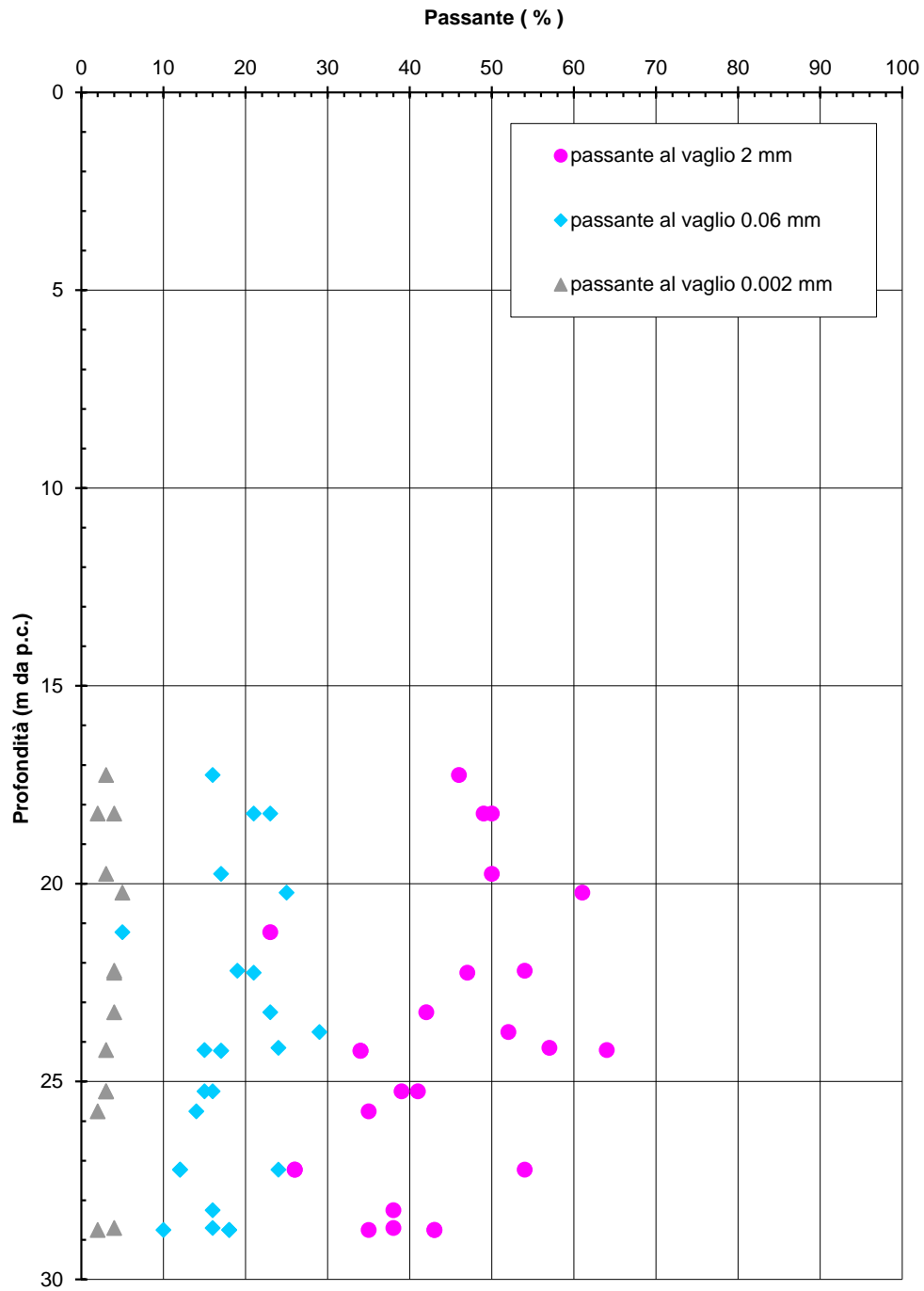
Figura 8-40 - Unità 4 - Granulometria sintetica da prove di laboratorio.
