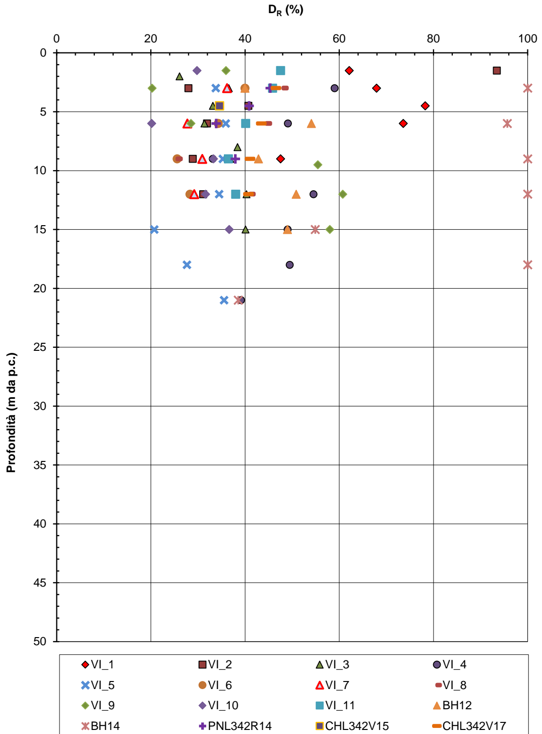
Figura 8-19 - Unità 2 - Stima densità relativa da prove SPT
