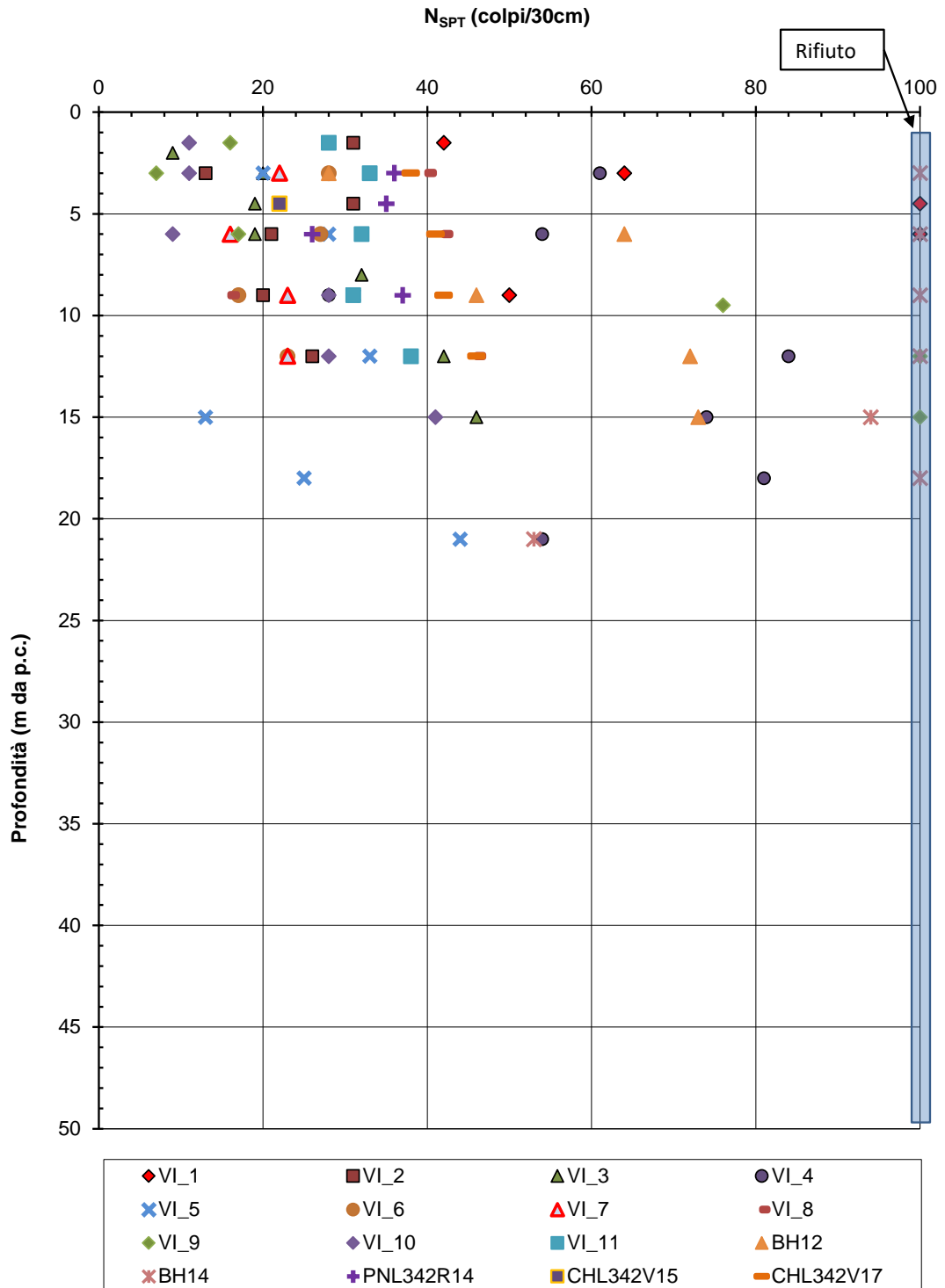
Figura 8-18 - Unità 2 - Prove SPT
