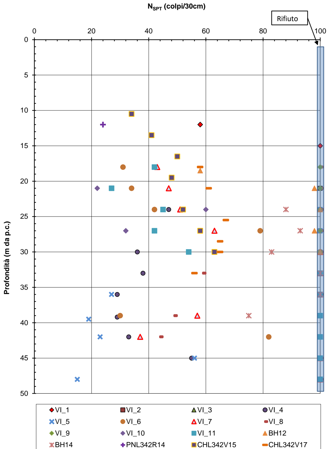
Figura 8-41 - Unità 4 - Prove SPT
