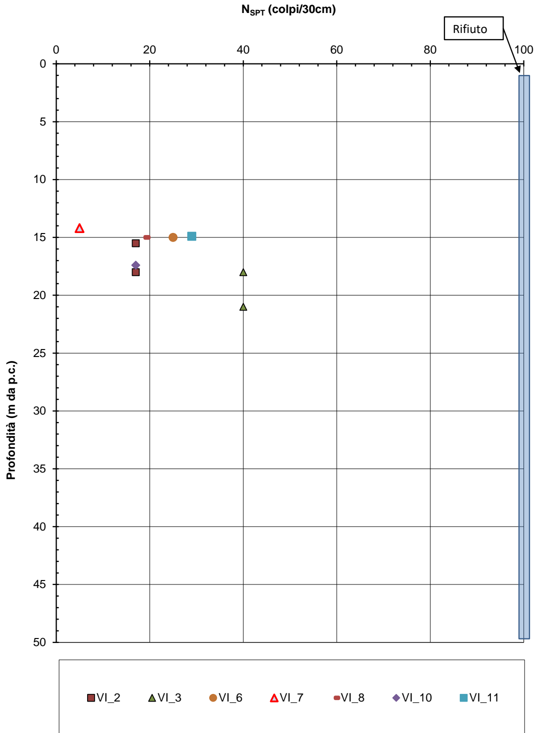
Figura 8-31 - Unità 3 - Prove SPT
