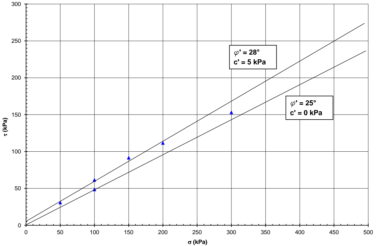
Figura 8-10 - Unità 1 - Stima coesione efficace e angolo di attrito da prove di laboratorio
