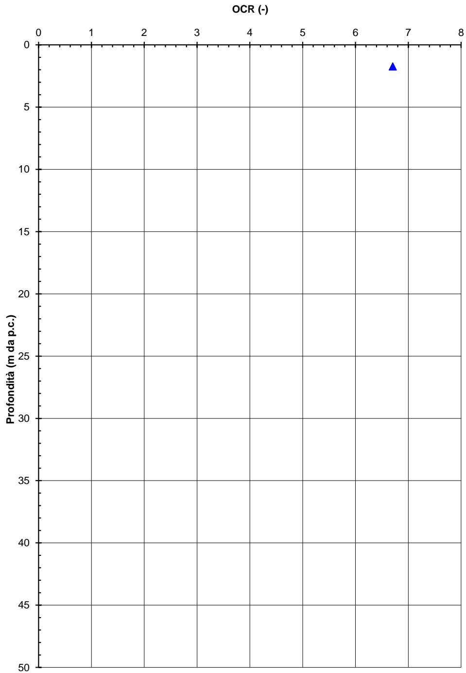
Figura 8-16 – Unità 1 - Grado di sovraconsolidazione da prove edometriche
