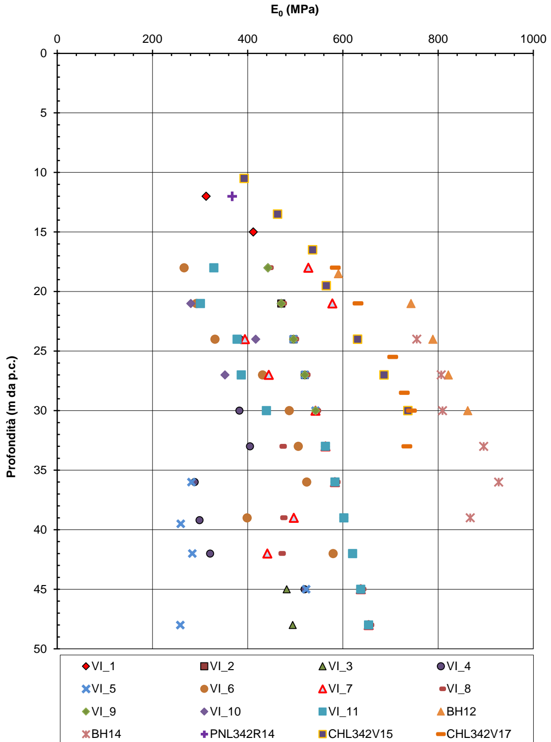
Figura 8-45 - Unità 4 - Stima modulo di Young a piccole deformazioni da prove SPT
