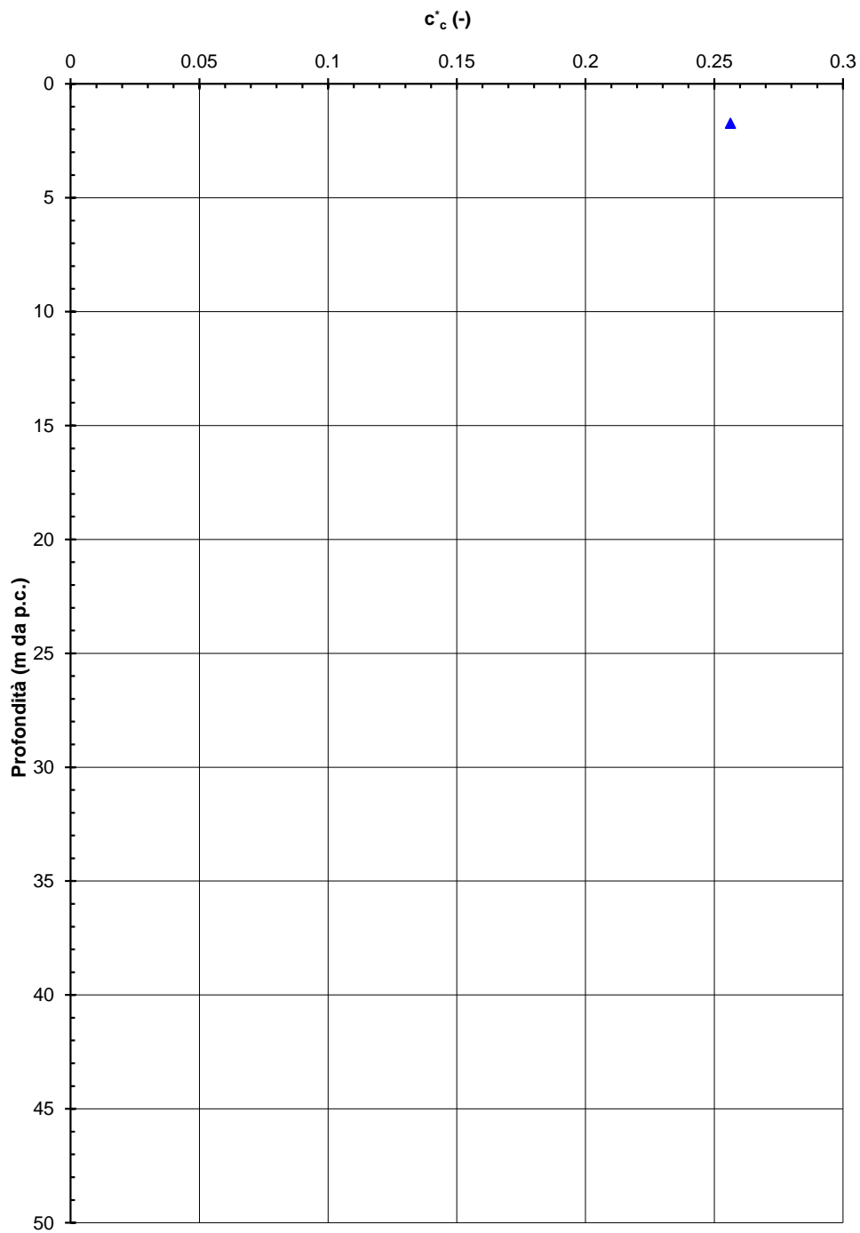
Figura 8-14 – Unità 1 - Coefficiente di compressione vergine ( Cc^* ) sul piano di Burland (1990)
