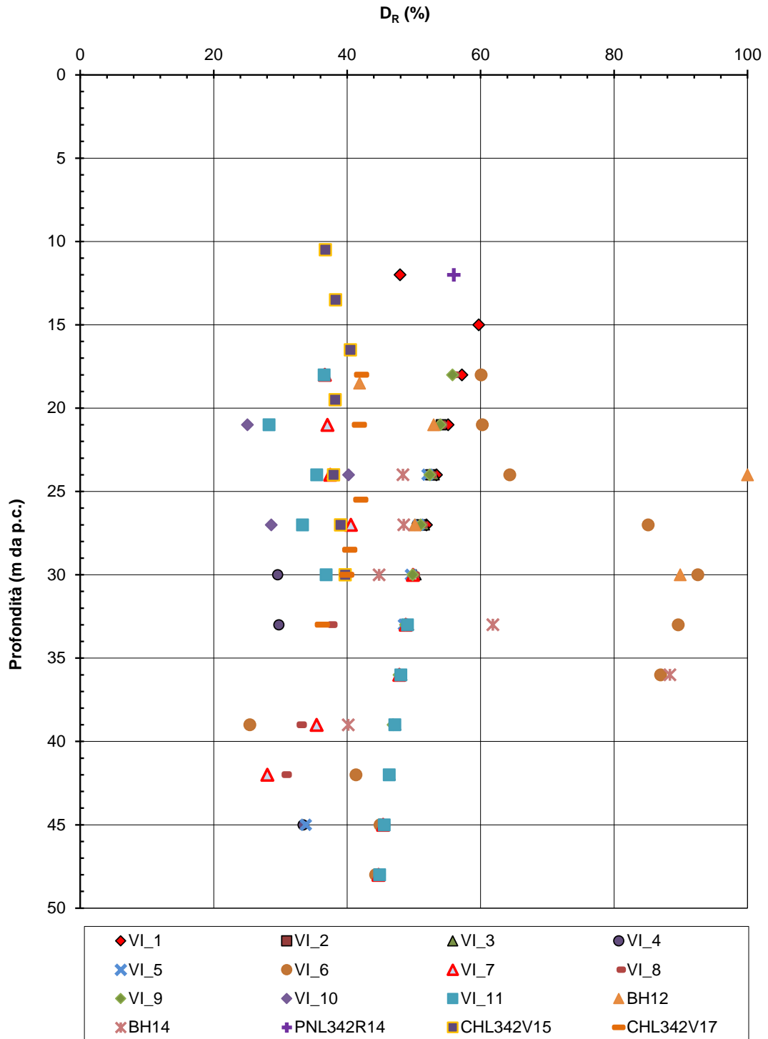
Figura 8-42 - Unità 4 - Stima densità relativa da prove SPT
