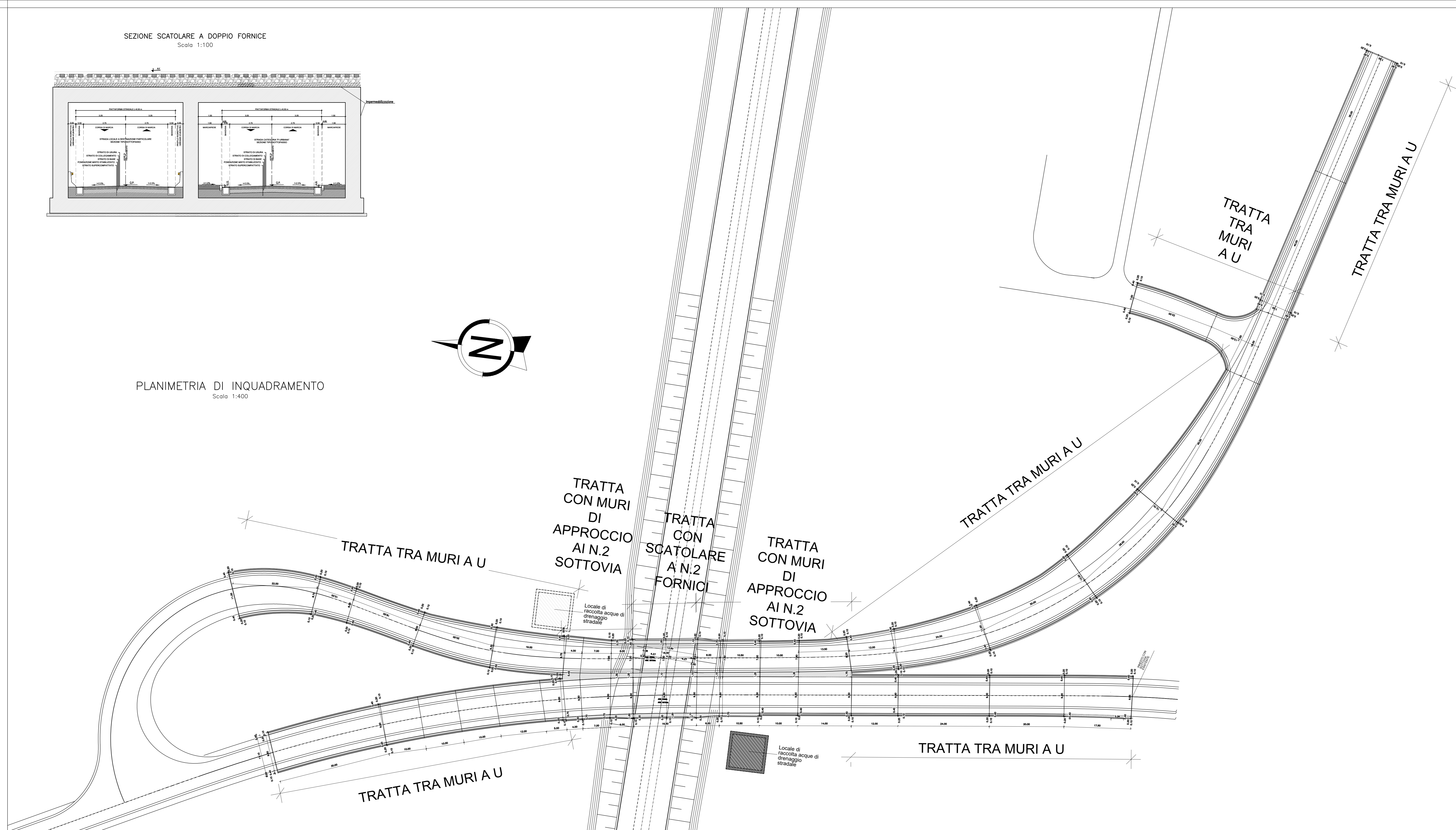
PIANTA CARPENTERIA quota testa muri Scala 1:200
