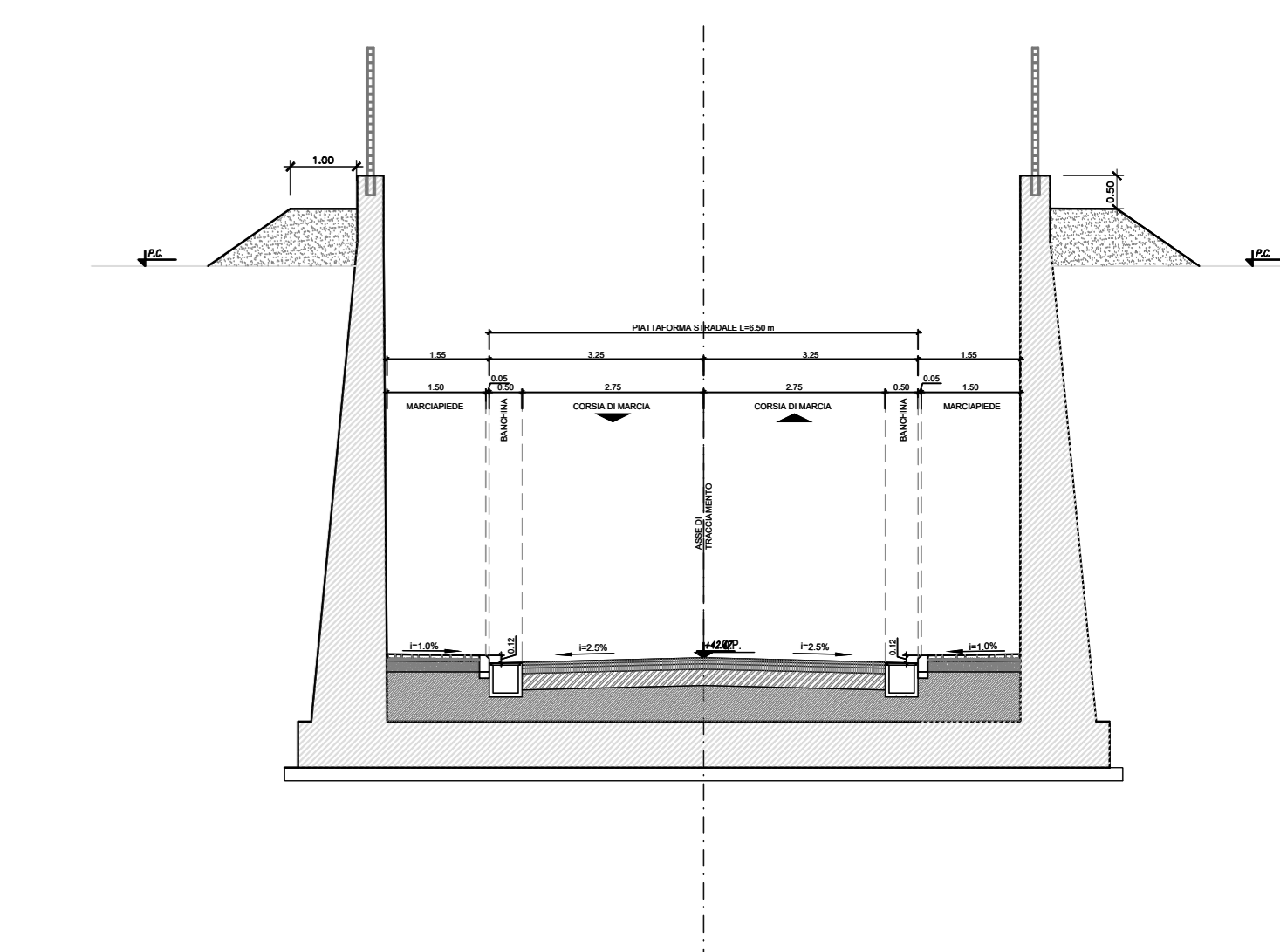
SEZIONE TRA MURI A U con strada da 9,50m Scala 1:100
