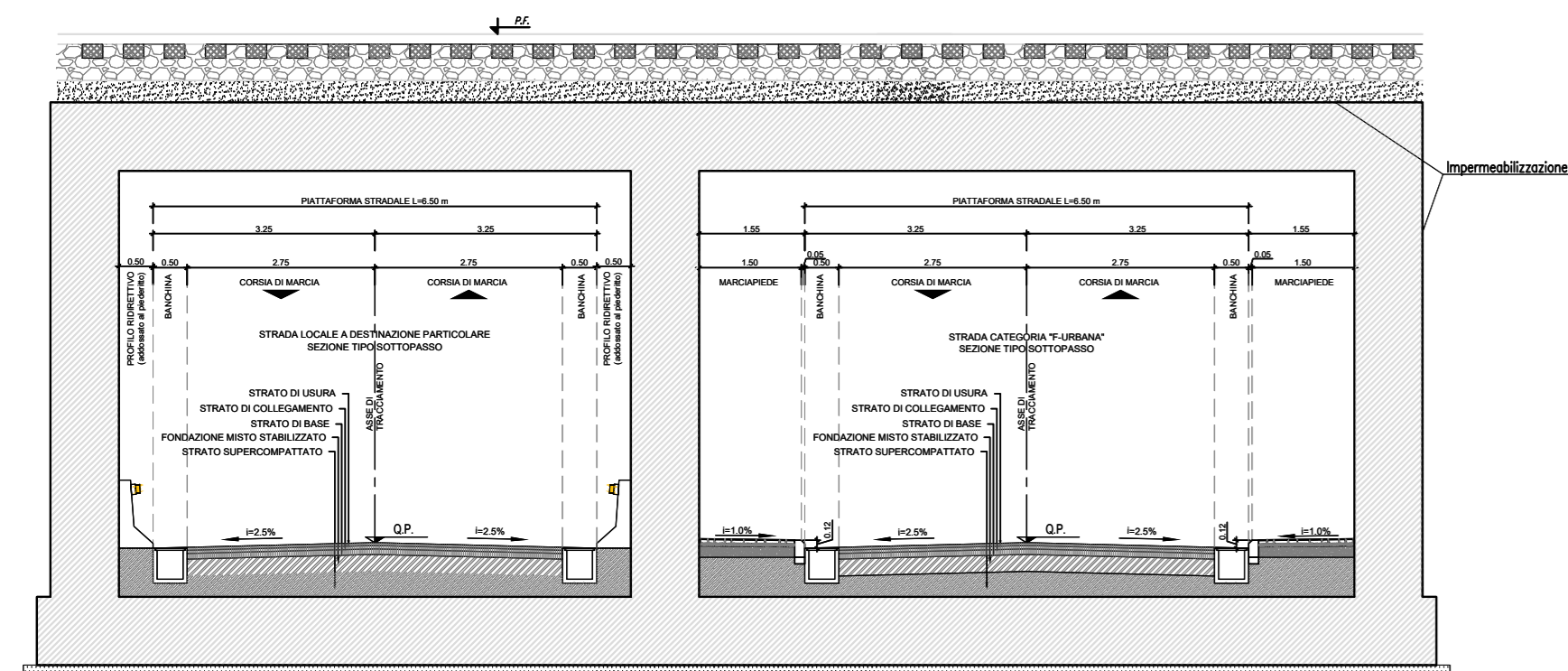
SEZIONE SCATOLARE A DOPPIO FORNICE Scala 1:100
