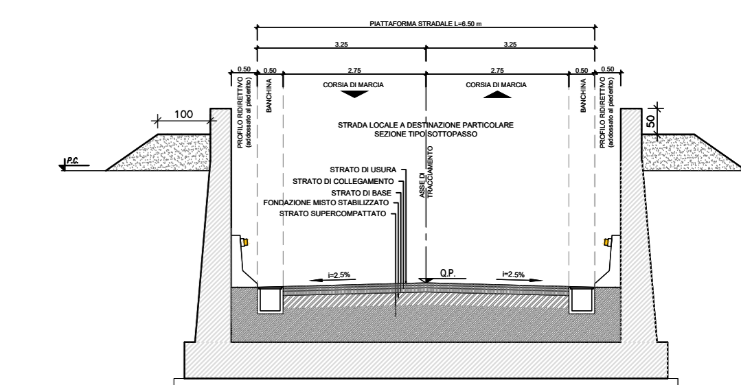
SEZIONE TRA MURI A U con strada da 6,50m Scala 1:100
