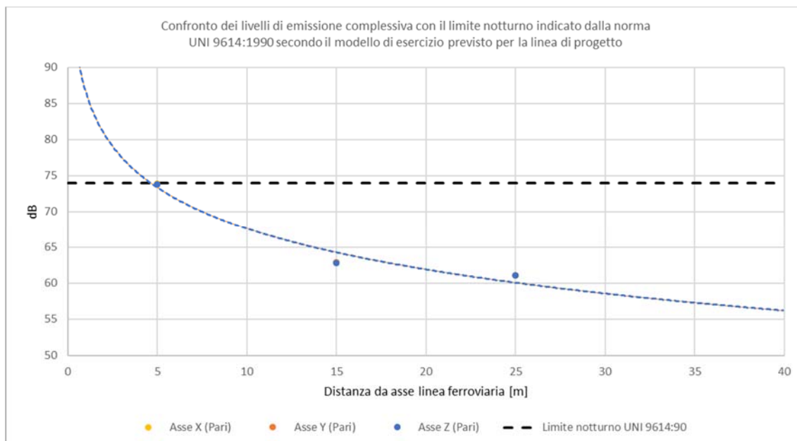
Figura 1-25 Confronto dei livelli di emissione complessiva all'interno degli edifici con i limiti UNI 9614:1990 in funzione della distanza dal binario pari secondo il modello di esercizio previsto - Periodo notturno
