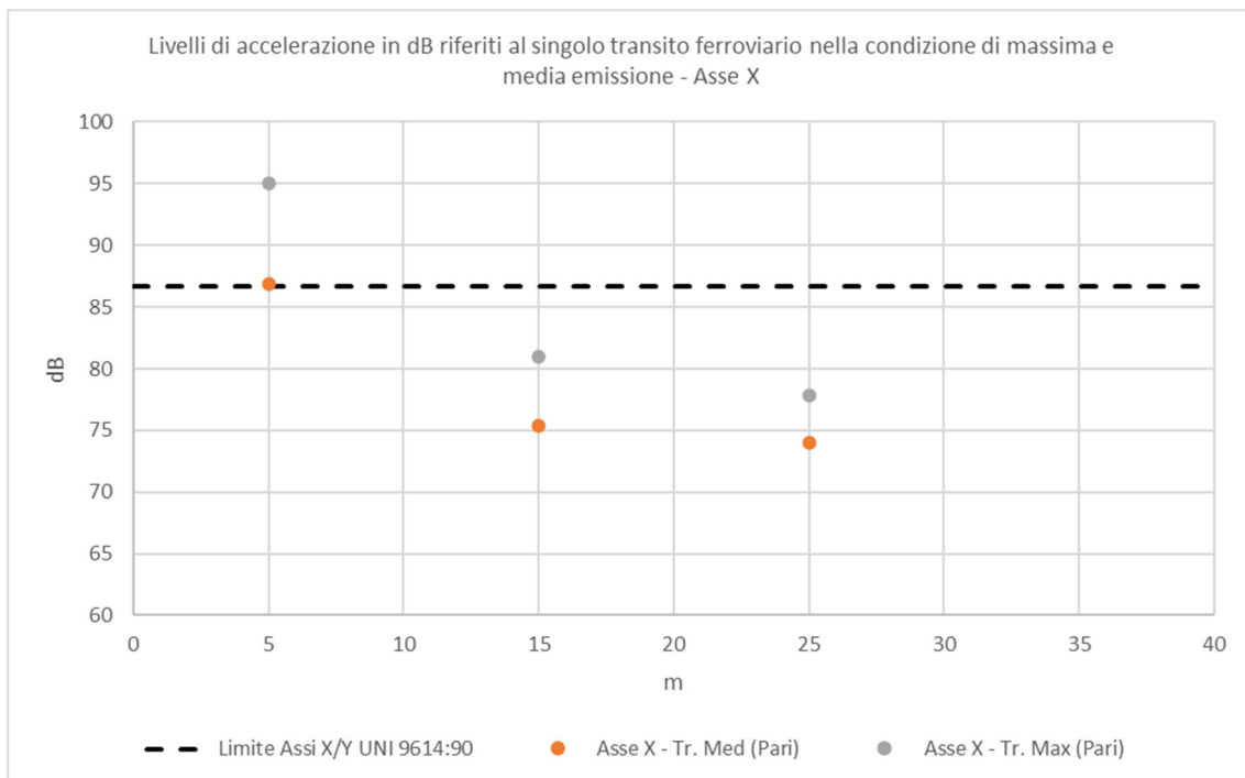
Figura 1-7 Livelli di accelerazione lungo l'asse X rappresentativi delle condizioni di massima e media emissione di un singolo transito ferroviario sul binario pari a 5, 15 e 25 m dall'asse del binario e confronto con il livello limite per gli assi X e Y della UNI 9614:1990 per i singoli transiti ferroviari (appendice A4)
