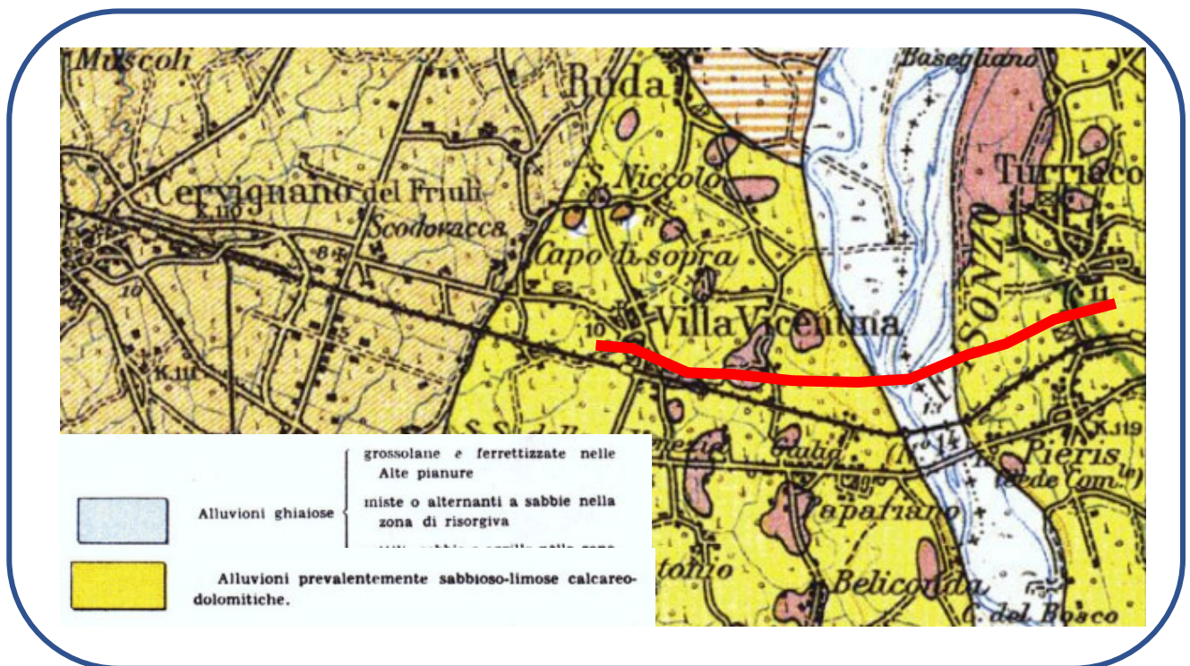
Figura 1-2 Stralcio non in scala della Carta Geologica d'Italia realizzata in scala 1:100.000 dal Servizio Geologico, Foglio n. 51
