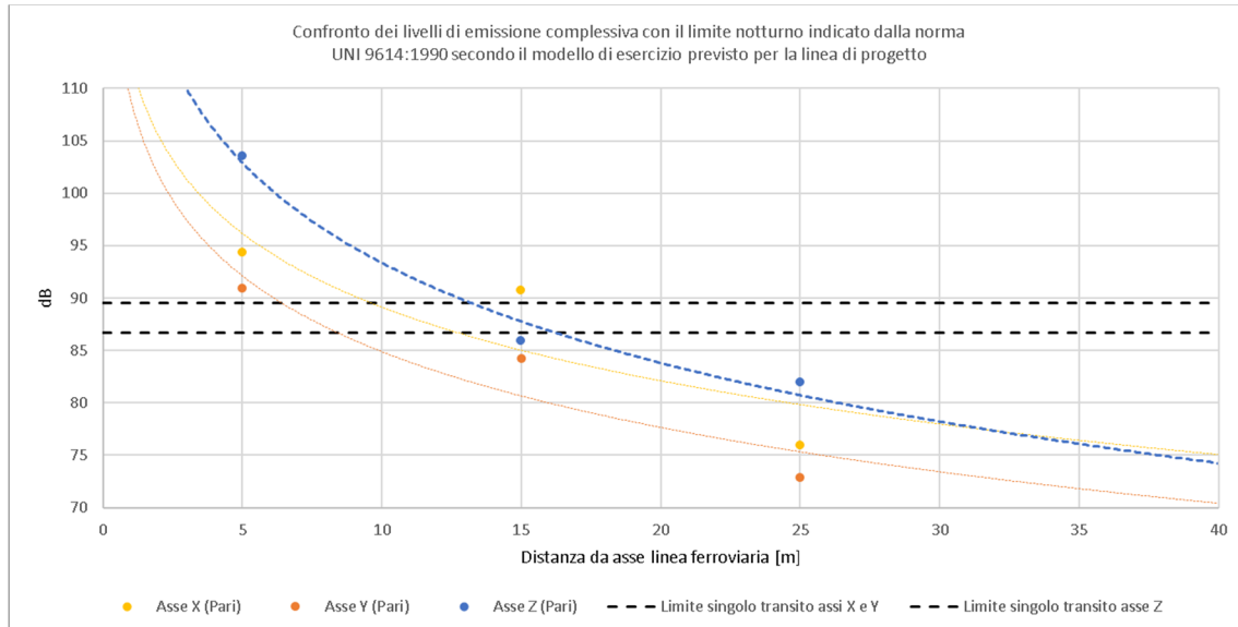
Figura 1-23 Confronto dei livelli di emissione massima riferiti al transito di un singolo convoglio ferroviario a 140 km/h in funzione della distanza dall'asse del binario pari con i limiti indicati dalla UNI 9614:1990 in Appendice A4
