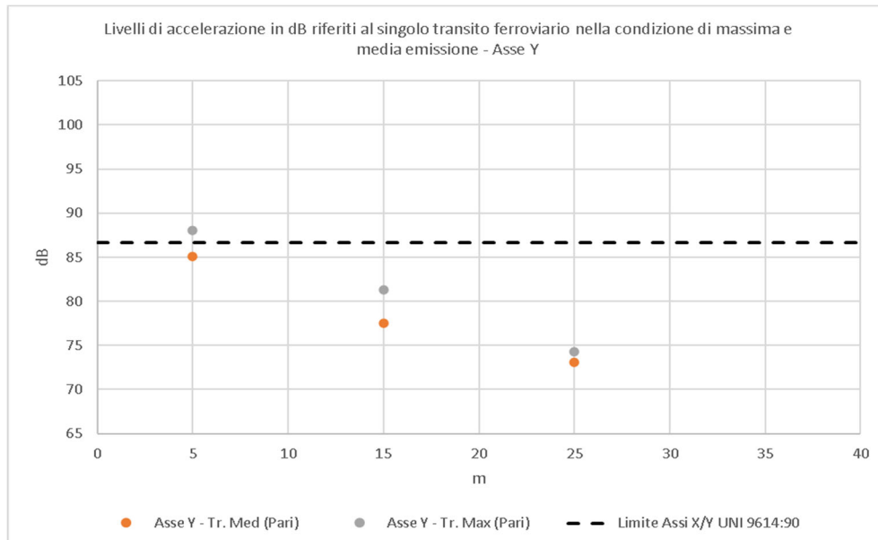
Figura 1-8 Livelli di accelerazione lungo l'asse Y rappresentativi delle condizioni di massima e media emissione di un singolo transito ferroviario sul binario pari a 5, 15 e 25 m dall'asse del binario e confronto con il livello limite per gli assi X e Y della UNI 9614:1990 per i singoli transiti ferroviari (appendice A4)
