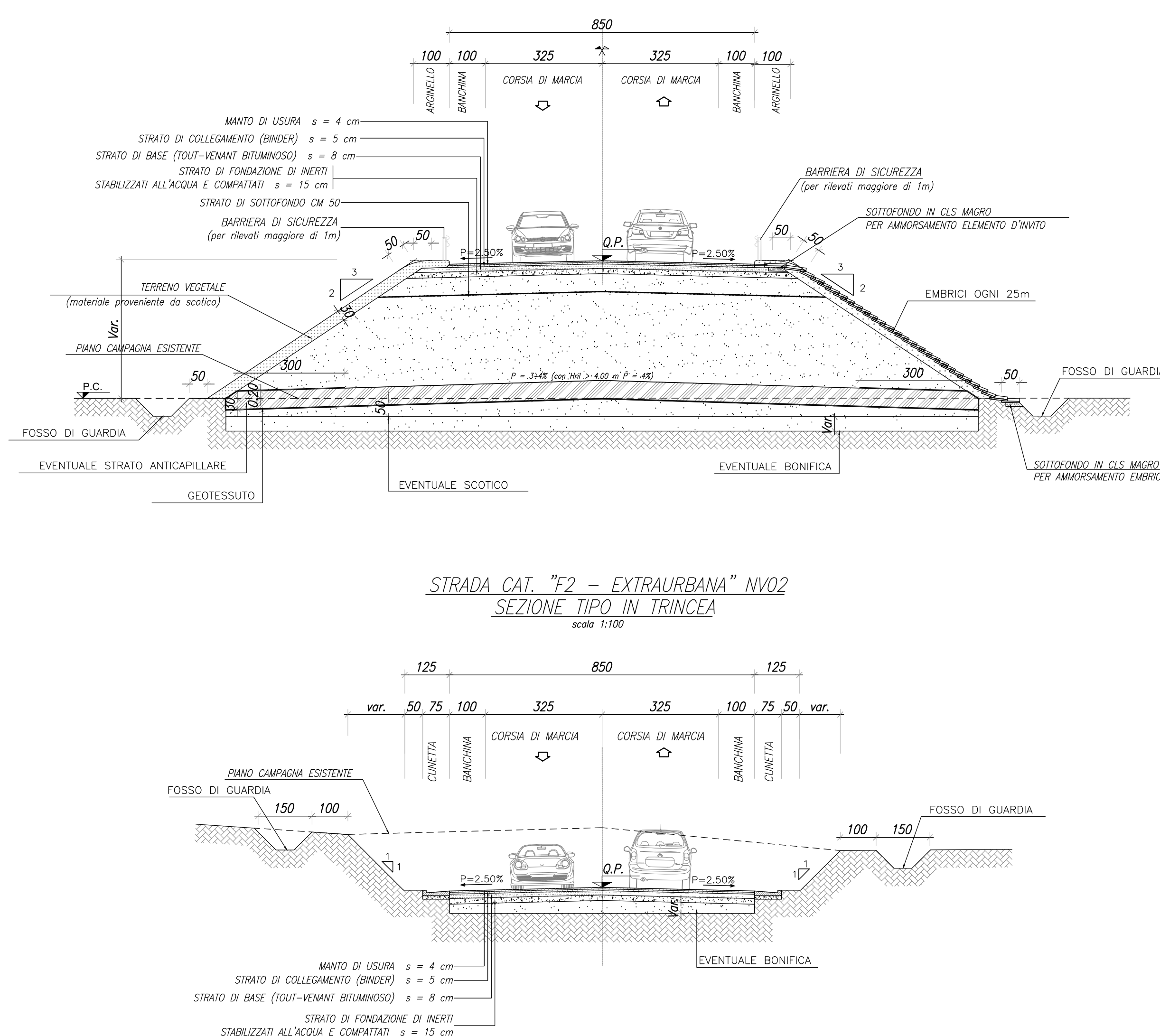
STRADA CAT. "F2 - EXTRAURBANA" NVO2 SEZIONE TIPO IN RILEVATO scala 1:100
