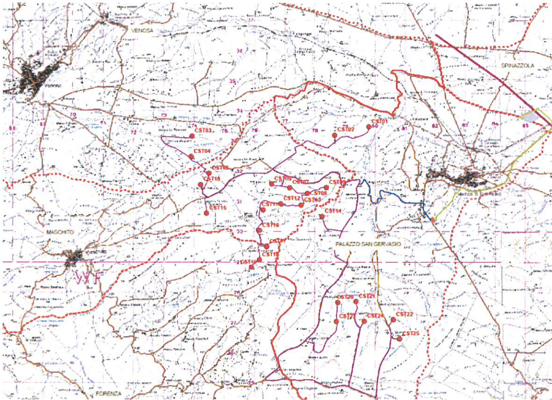
Layout di confronto tra la prima e la seconda soluzione progettuale. Nell'immagine sottostante quella oggetto della presente istanza di proroga.
