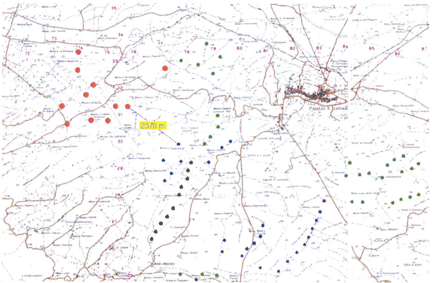
Figura 10: Inquadramento rispetto agli altri impianti: in rosso le torri di progetto; in blu le torri autorizzate; in verde quelle esistenti
