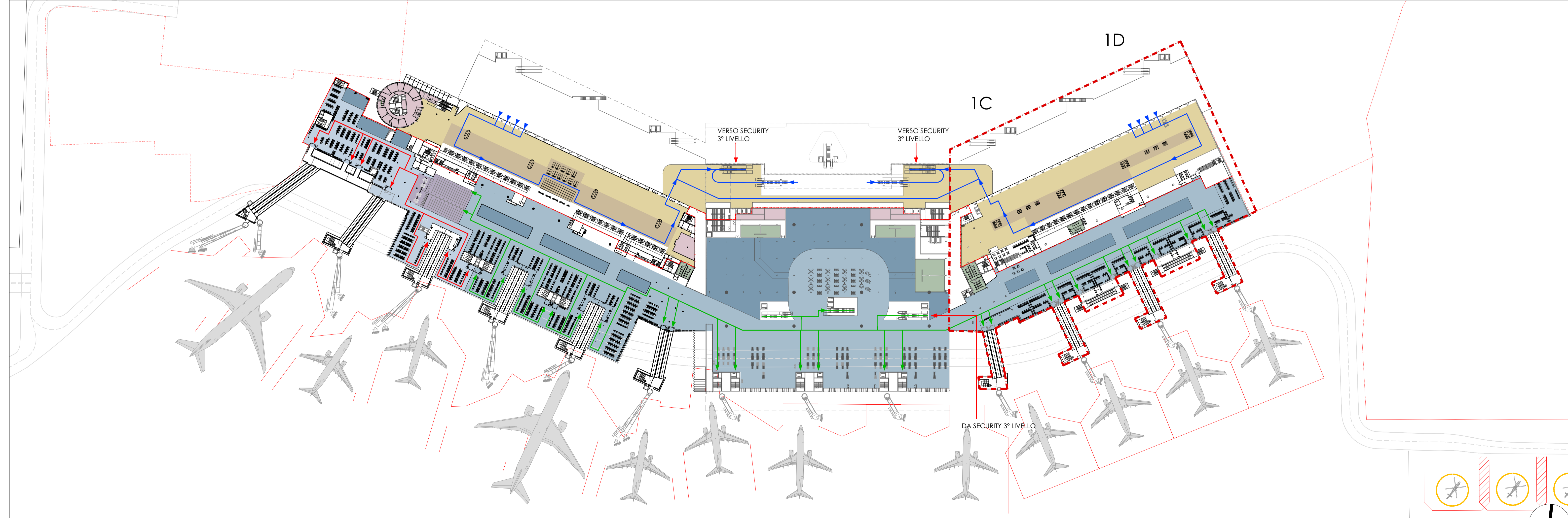
PIANTA LIVELLO PARTENZE
