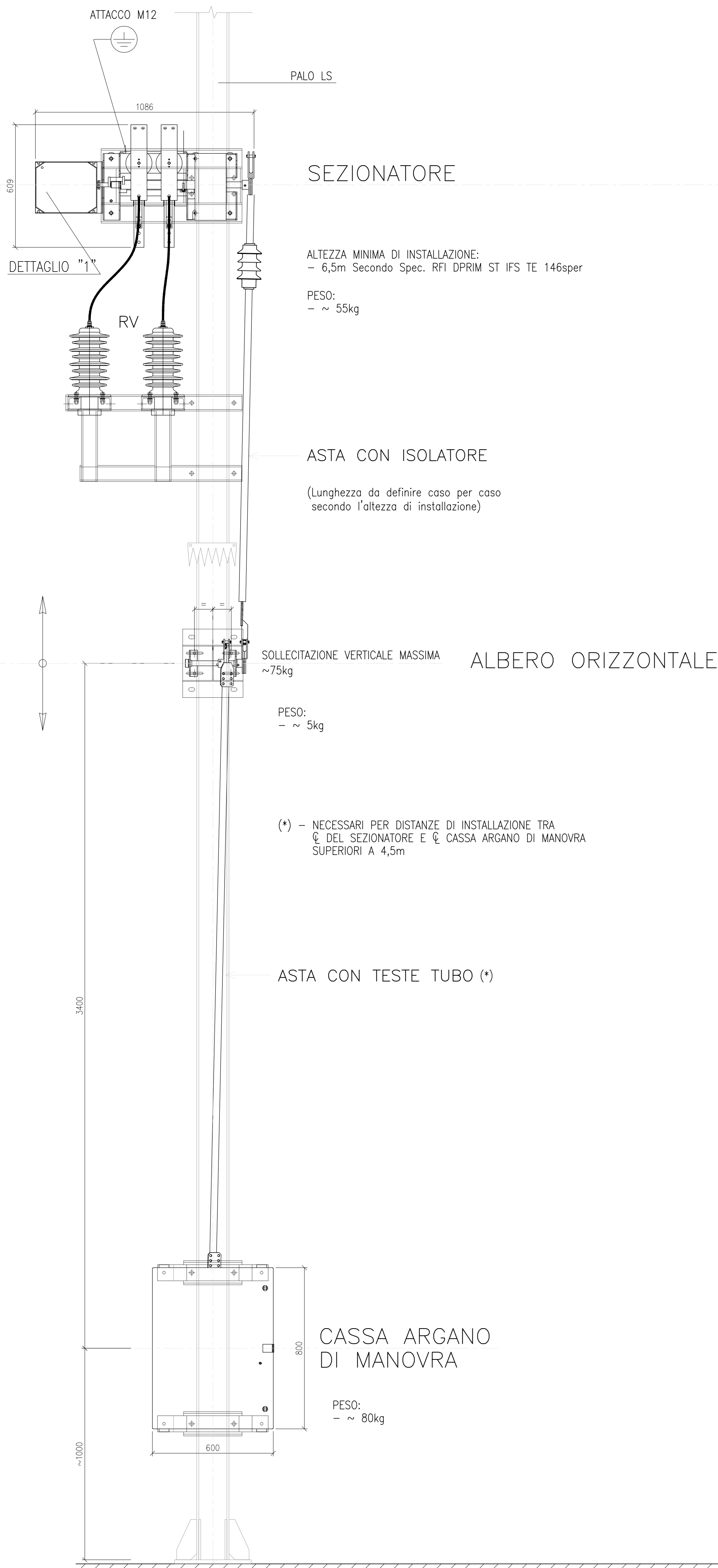
VISTA FRONTALE
