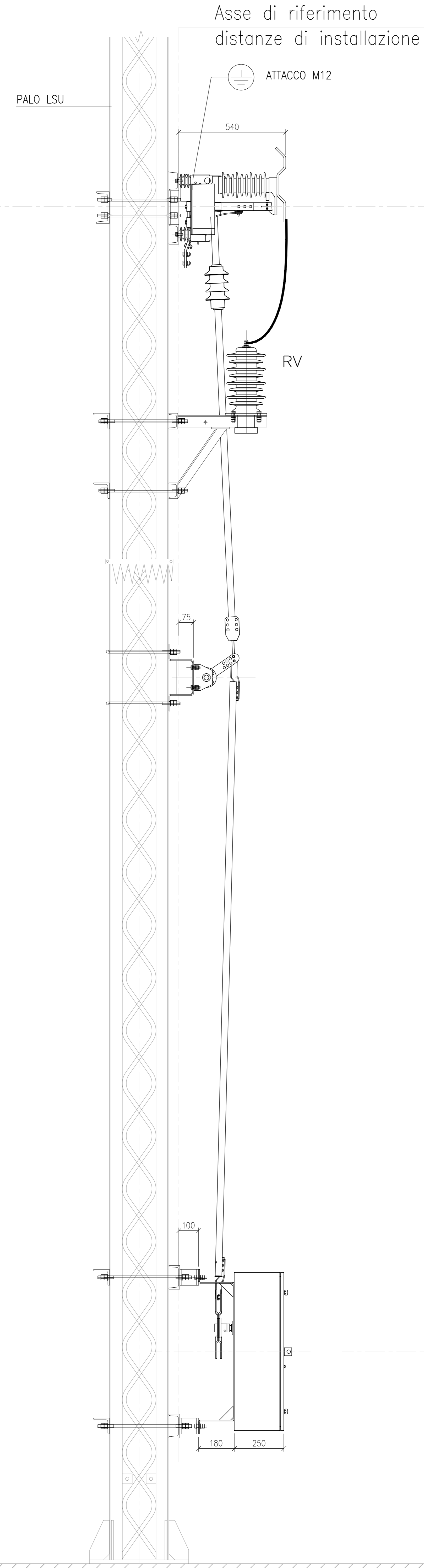
VISTA LATERALE
