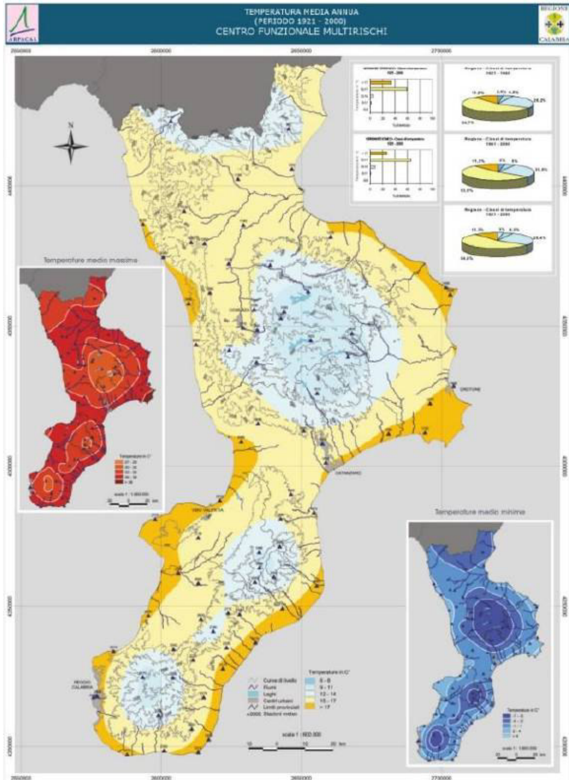
FIGURA 4 DISTRIBUZIONE DELLE TEMPERATURE MEDIE ANNUE IN CALABRIA (ARPA CAL 1921-2000) TRATTO DAL PIANO FORESTALE REGIONALE 2014-2020
