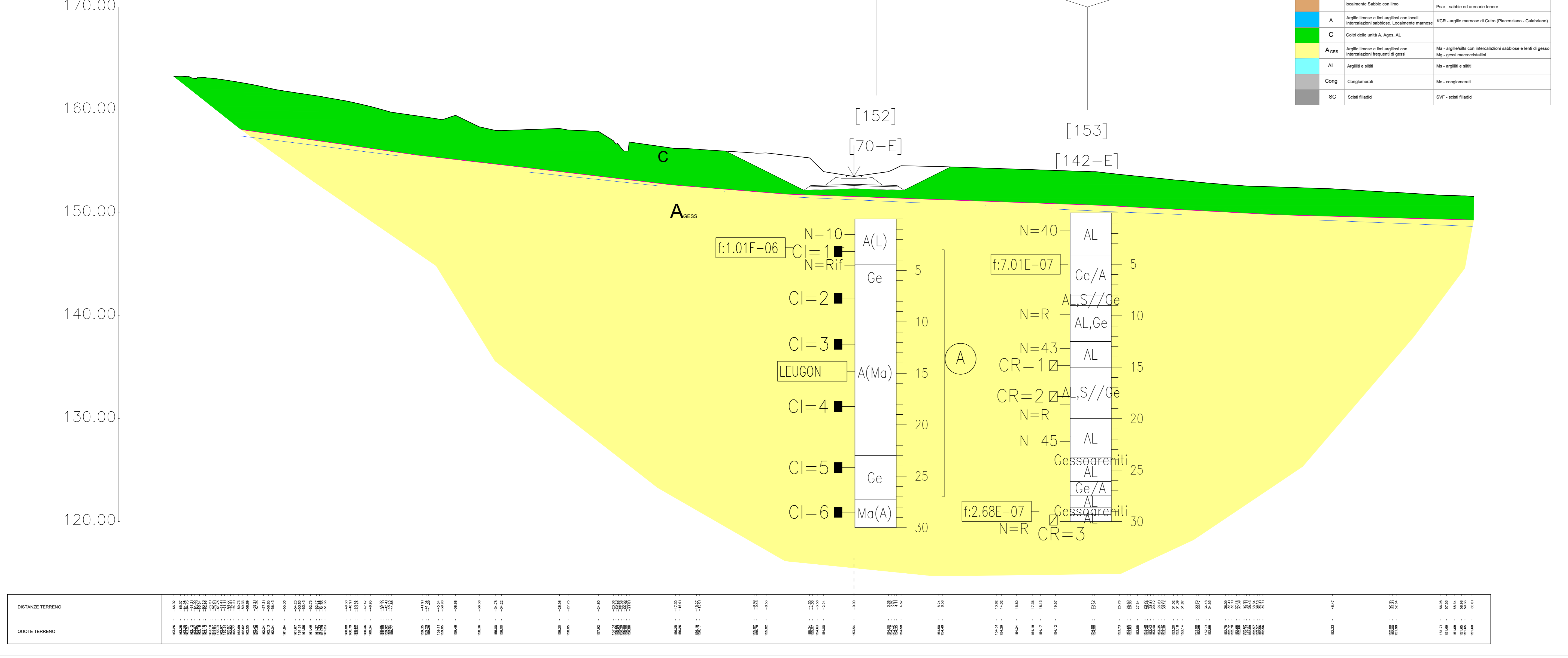
SEZIONE AA' - GEOTECNICA SCALA 1:200
