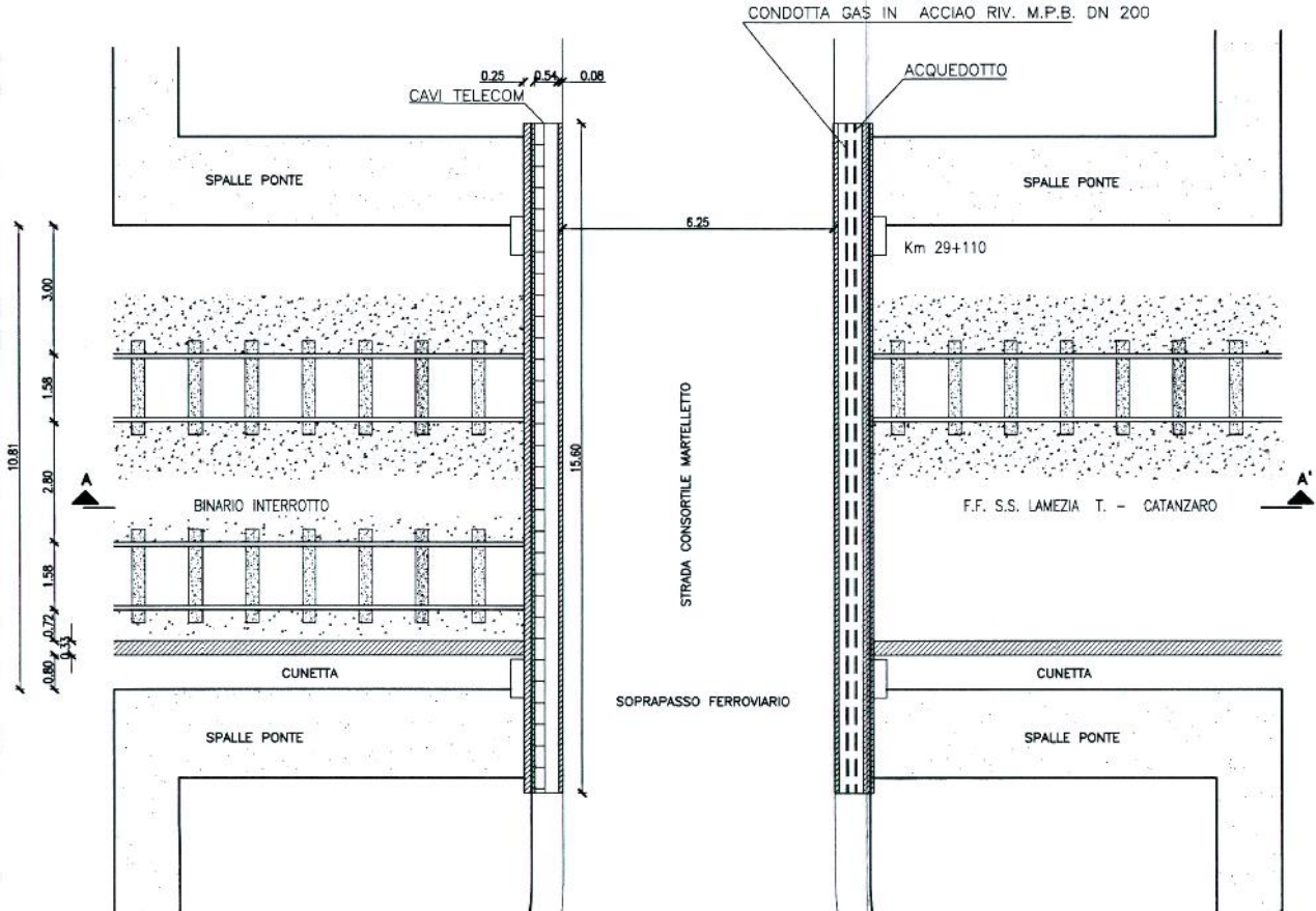
SEZIONE A-A' Scala 1:100
