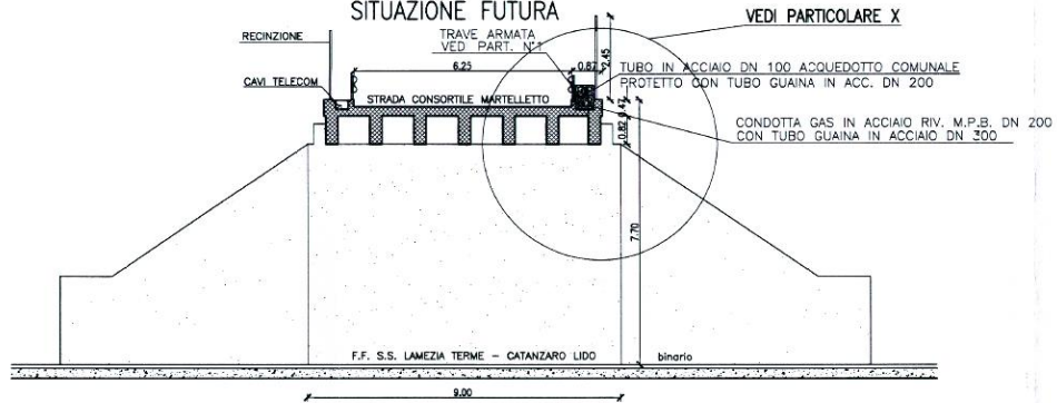
PROSPETTO A' SCALA 1:100
