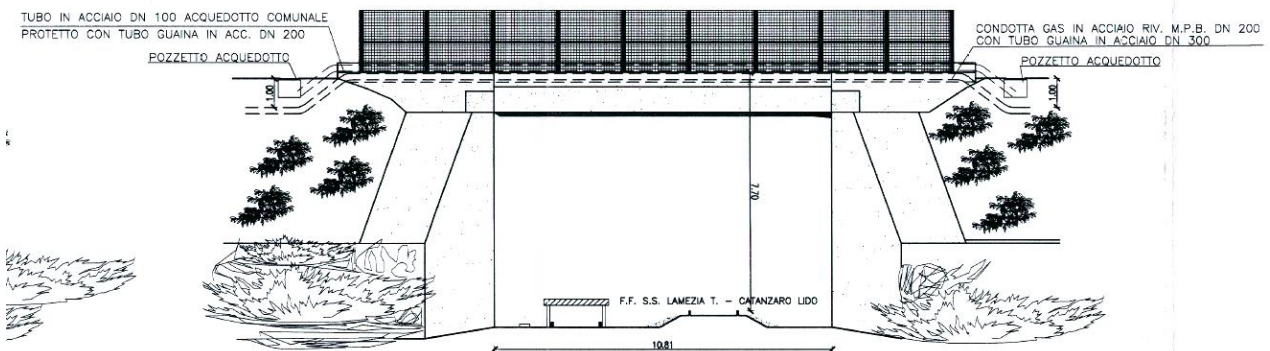
PROSPETTO A' SCALA 1:100
