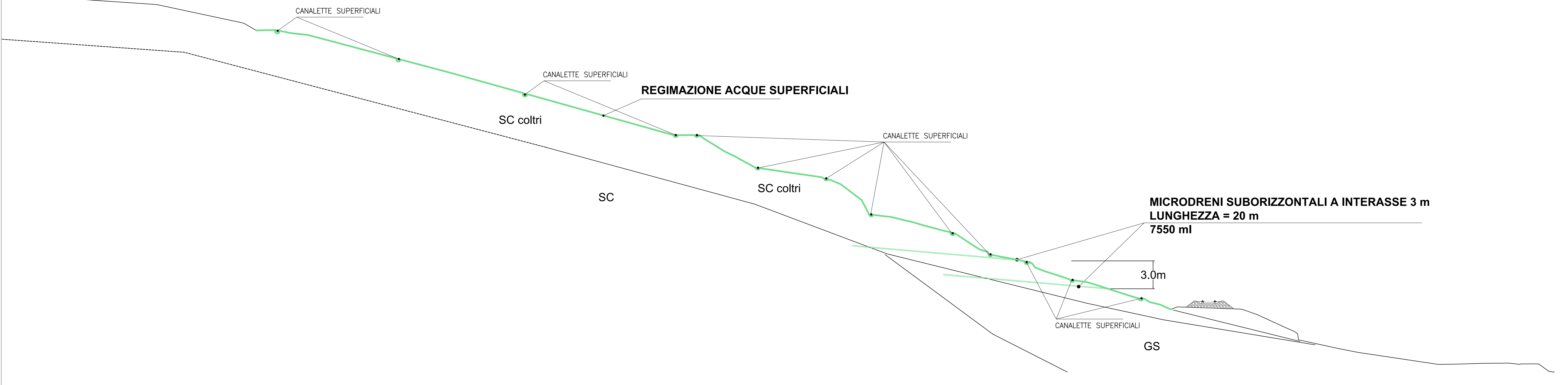
SEZIONE AA' - GEOTECNICA SCALA 1:500
