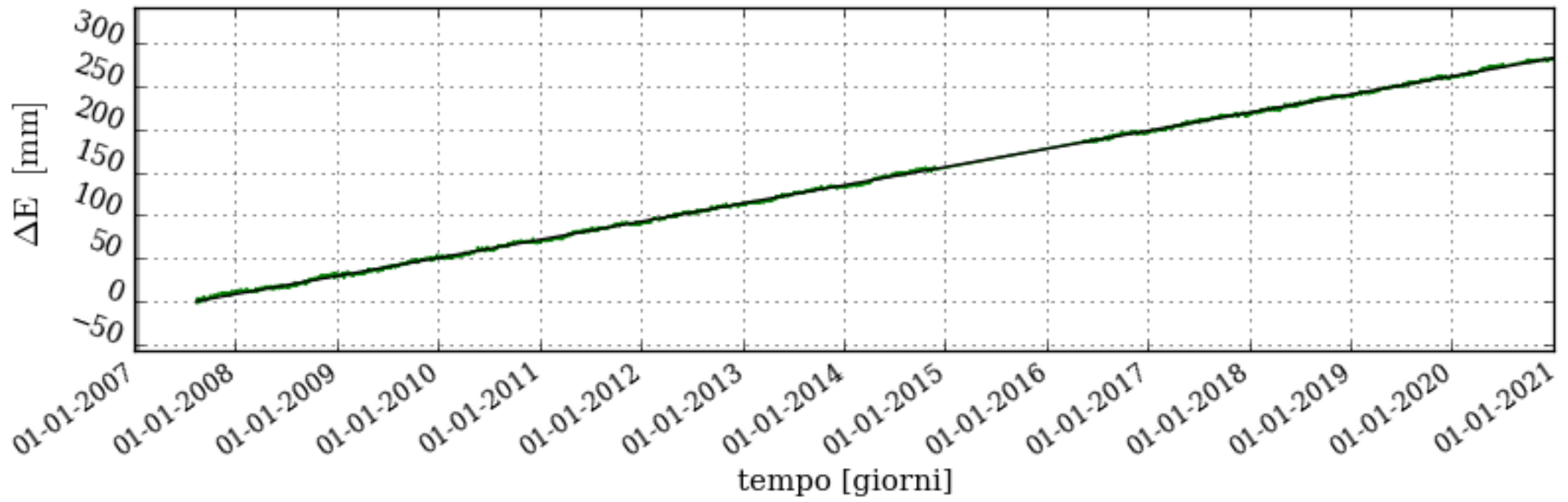
Serie Storica Est dal 08-08-2007 al 31-12-2020 AnemoneB
