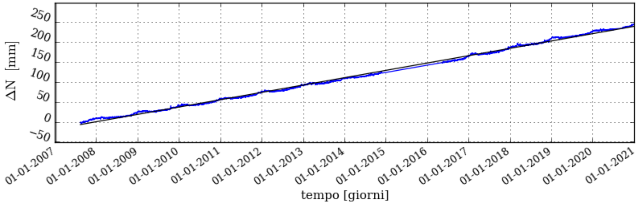
Serie Storica Nord dal 08-08-2007 al 31-12-2020 AnemoneB
