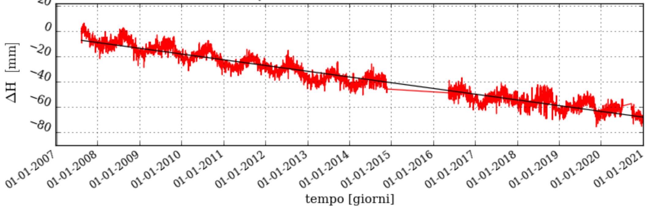
Serie Storica Quota dal 08-08-2007 al 31-12-2020 AnemoneB
