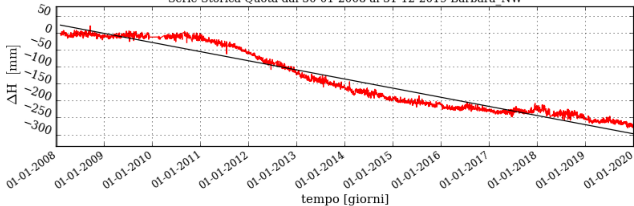
Serie Storica Quota dal 30-01-2008 al 31-12-2019 Barbara_NW
