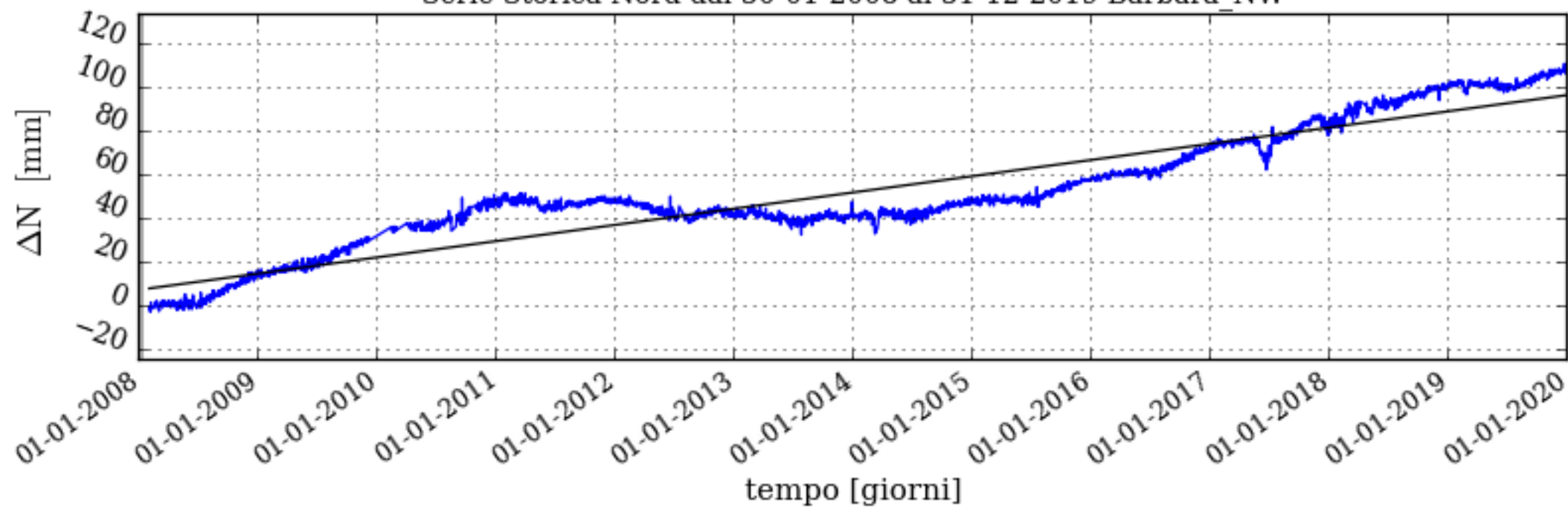
Serie Storica Nord dal 30-01-2008 al 31-12-2019 Barbara_NW
