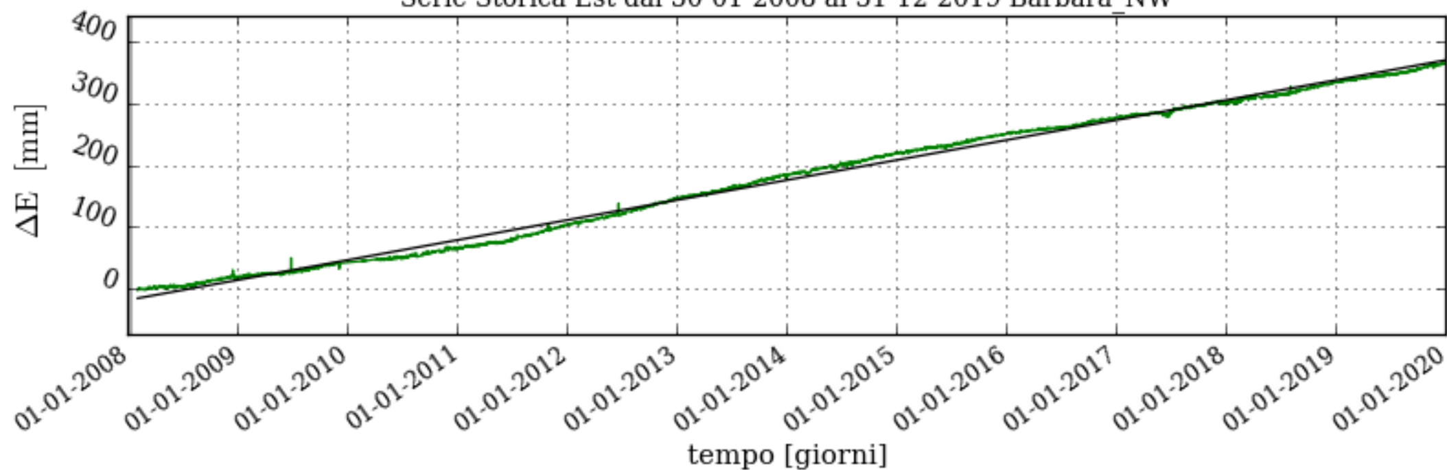
Serie Storica Est dal 30-01-2008 al 31-12-2019 Barbara_NW
