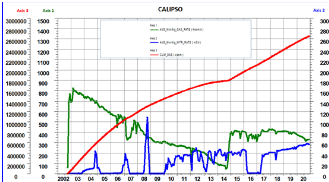
Figura 3 - Campo di Calipso: grafico di produzione storica
