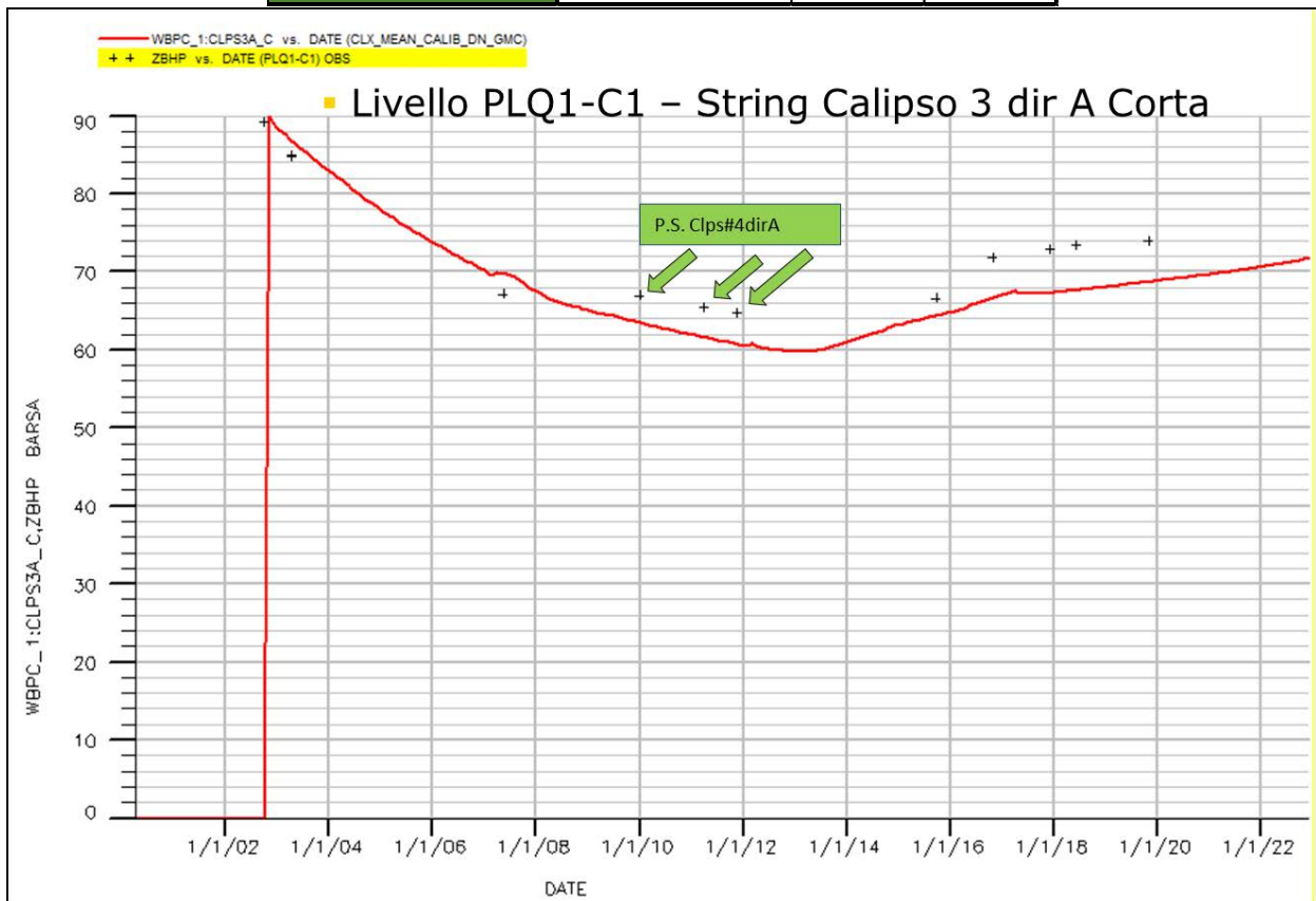
Figura 7 - Campo di Calipso: pressioni statiche misurate e modello Eclipse 2017 (livello PLQ1-C1)
