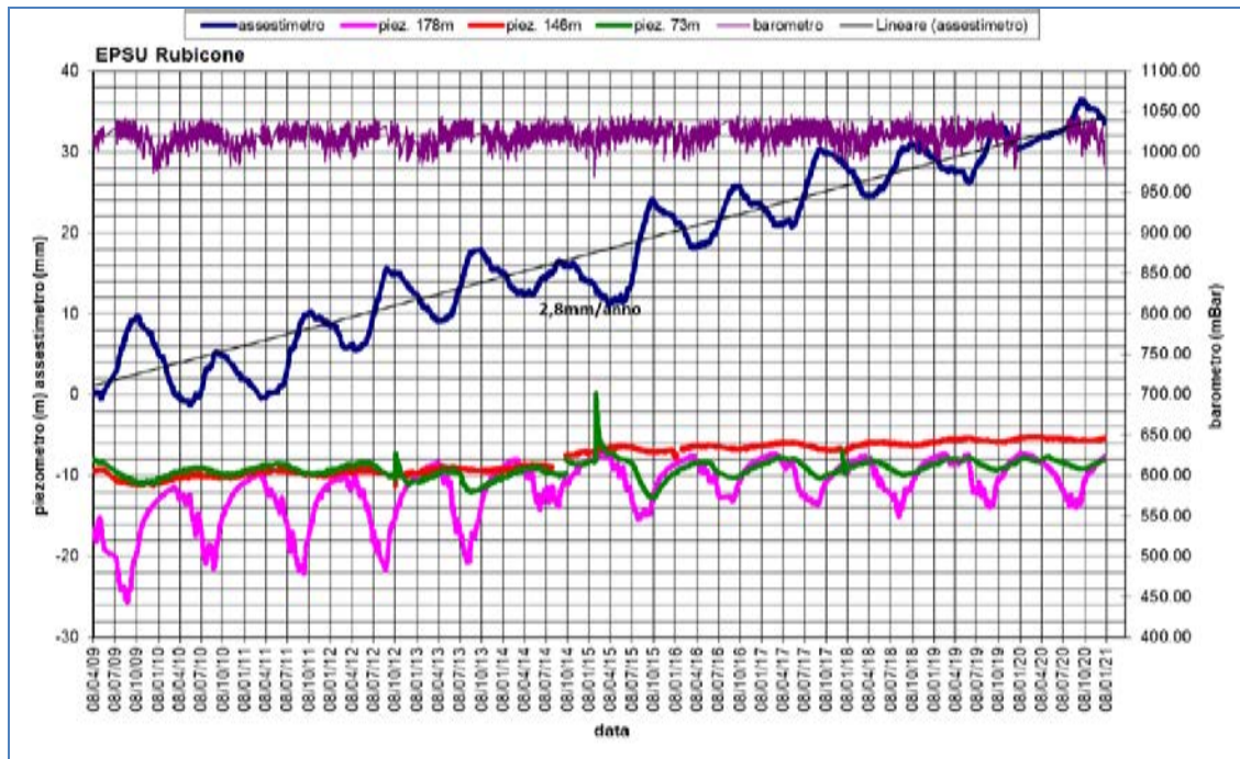
Figura 6B - Stazione EPSU di Rubicone: misure piezometriche, assestimentiche e barometriche
