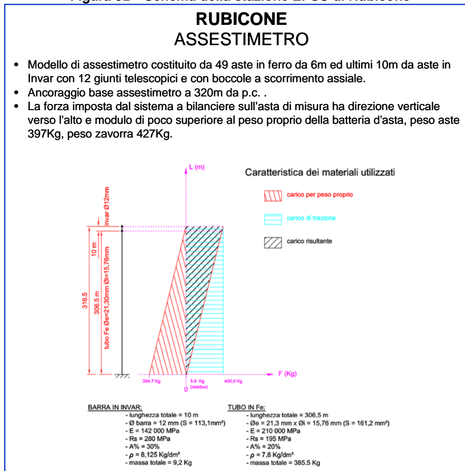
Figura 3B - Schema della stazione EPSU di Rubicone
