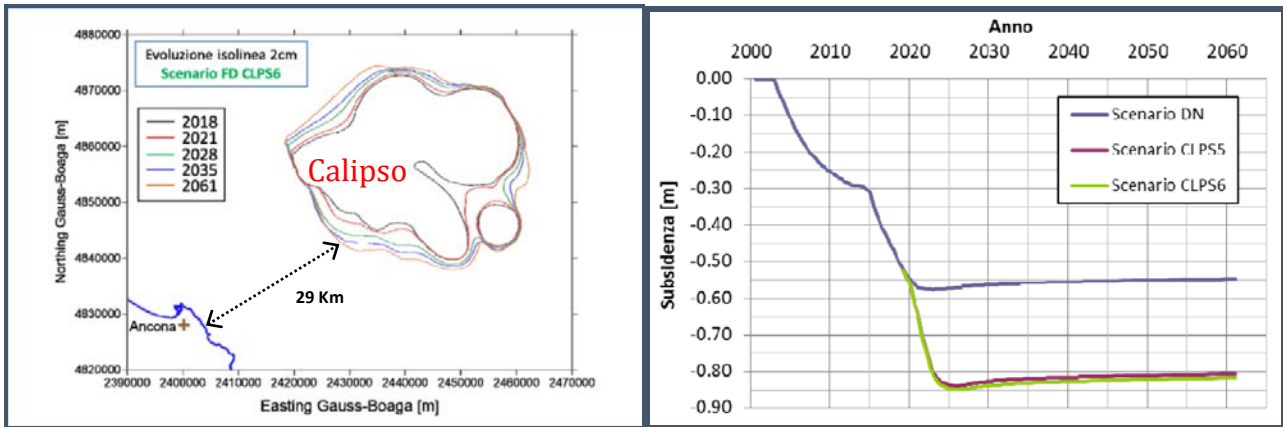
Figura 8 - Evoluzione nel tempo, rispettivamente della linea di iso-subsidenza di 2 cm (scenario CLPS6) e della subsidenza prevista nel punto di massimo, per i 3 scenari considerati
