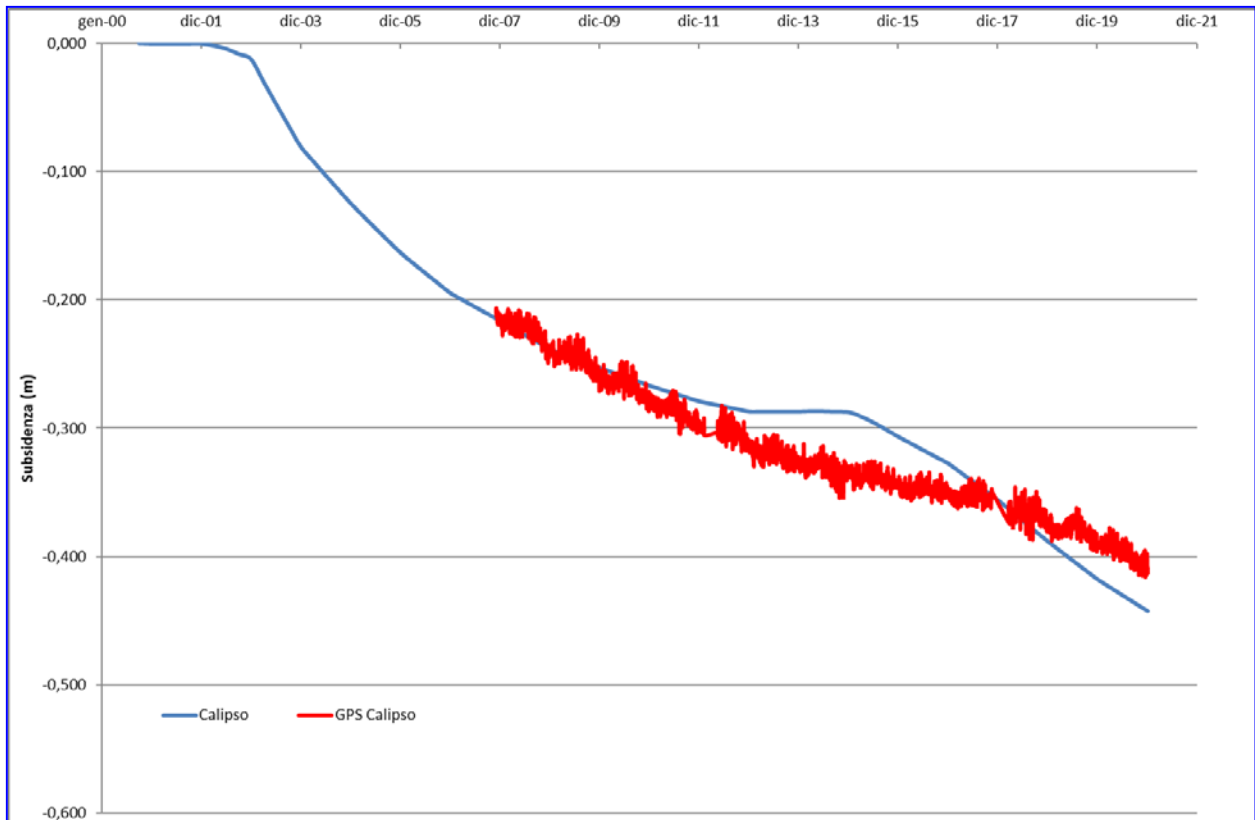
Figura 14 - Calipso: andamento della subsidenza misurata (CGPS in p.ma) vs. modello (scenario DN)
