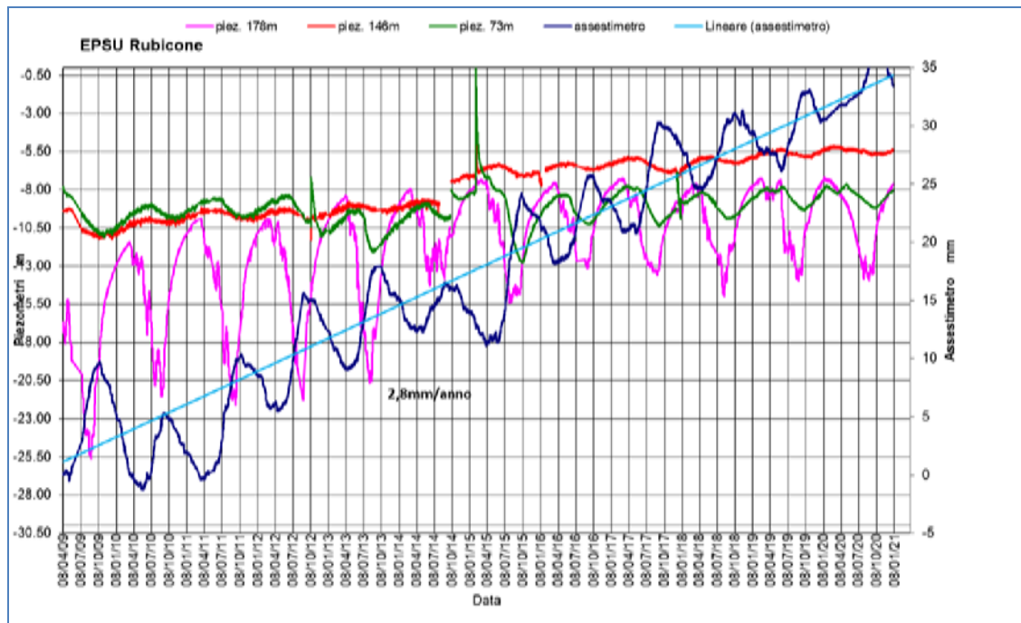
Figura 7B - Stazione EPSU di Rubicone: misure piezometriche e assestimentiche.
