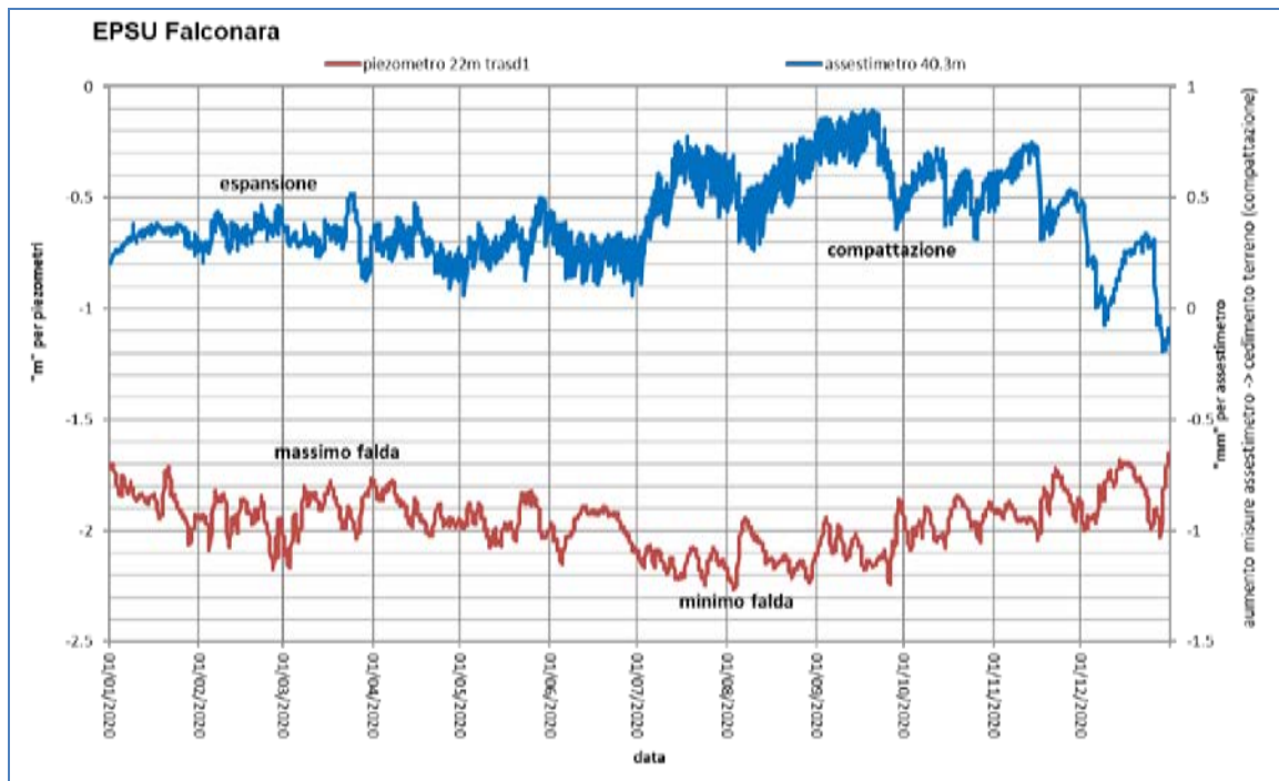
Figura 18B - Stazione EPSU di Falconara: misure piezometrico-assestimetriche, ultimo anno di da-
