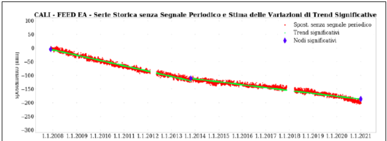
Figura 12 - Campo di Calipso: analisi della serie storica di misure CGPS
