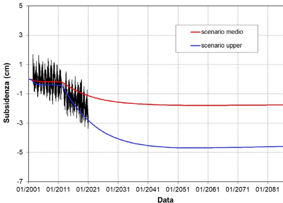
Figura 14 - Campo di Naomi-Pandora: misure CGPS depurate dalla componente naturale (agg. 31 dic. 2020) vs. modello di subsidenza (modello geomeccanico dicembre 2017)
