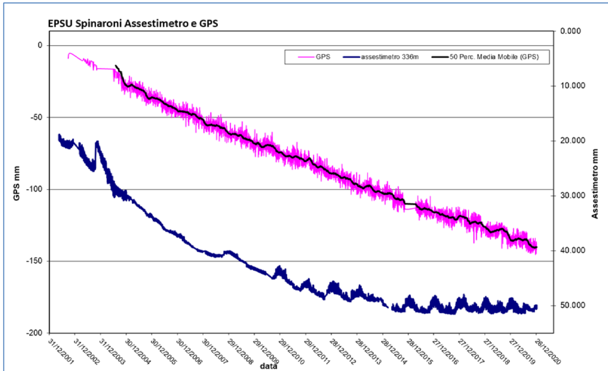
Figura 12B - Confronto fra misure da CGPS vs. misure di compattazione (assestmetro della stazione EPSU di Spinaroni)
