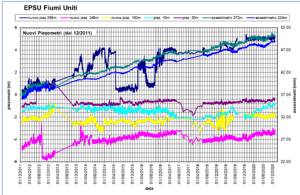
Figura 20B – Stazione EPSU Fiumi Uniti: misure piezometriche e assestimetriche dal 2011 al 2020
