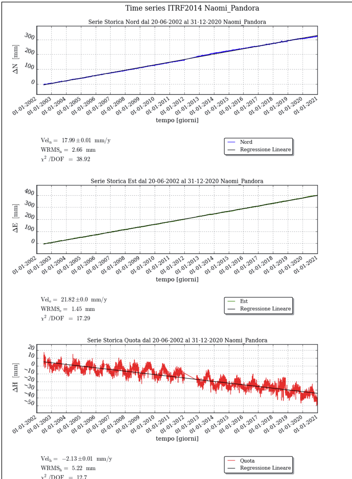
Figura 11 - Campo di Naomi-Pandora: serie storiche di misure CGPS al 31/12/2020
