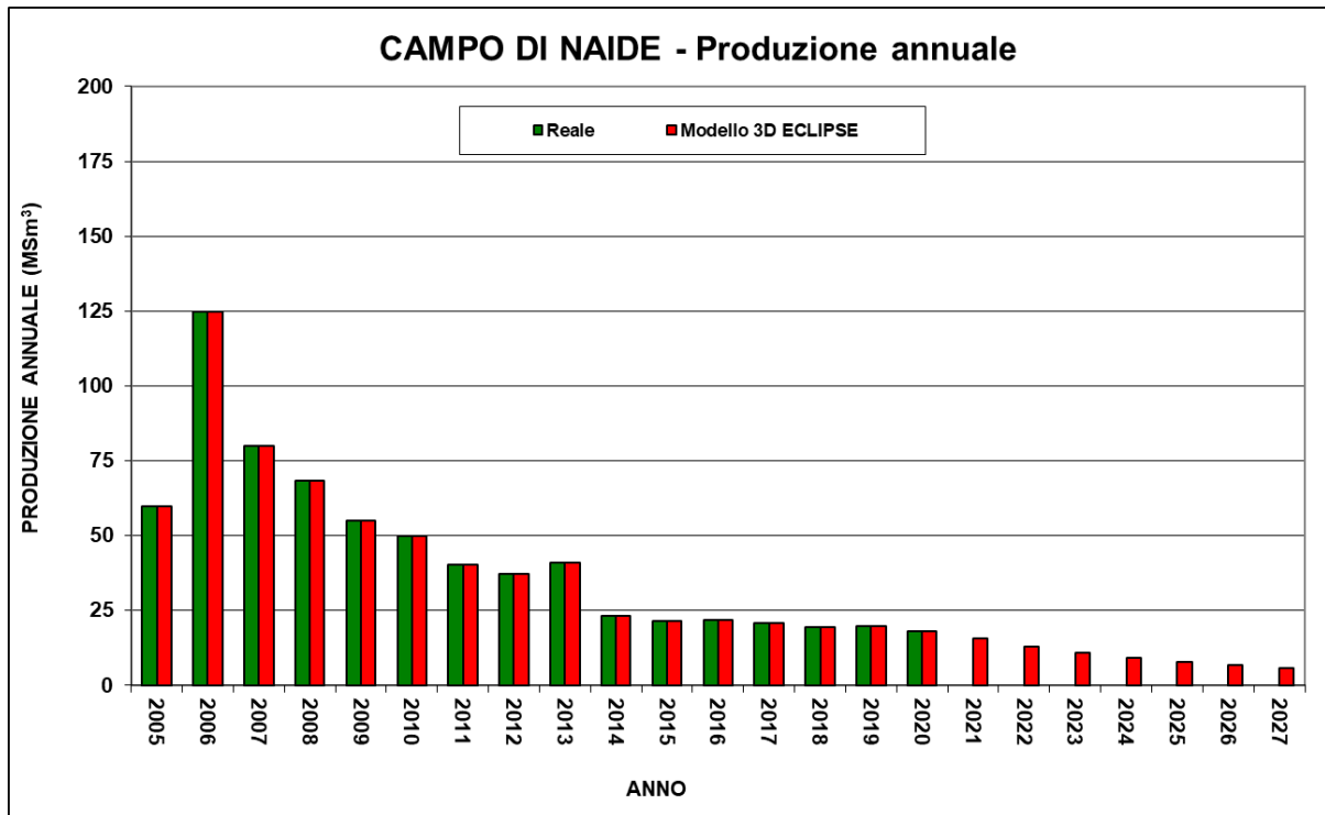
Figura 6 - Campo di Naide: produzione (annuale) reale e da modello Eclipse 2021
