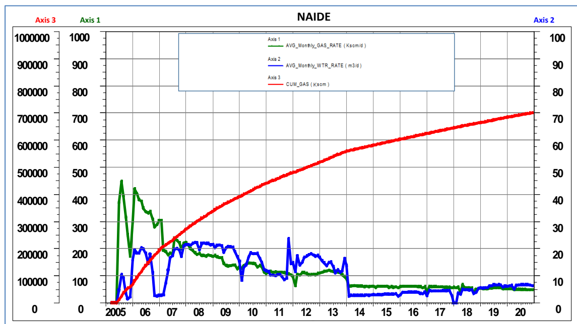
Figura 3 - Campo di Naide: produzione storica
