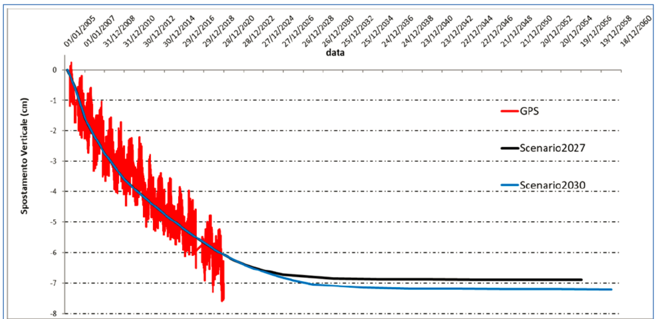
Figura 13 – Campo di Naide: subsidenza misurata e calcolata in corrispondenza della stazione CGPS
