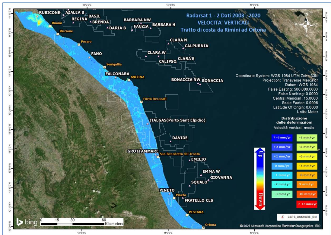
Figura 10 - Campo di Naide: analisi dati SAR dal 2003 al 2020
