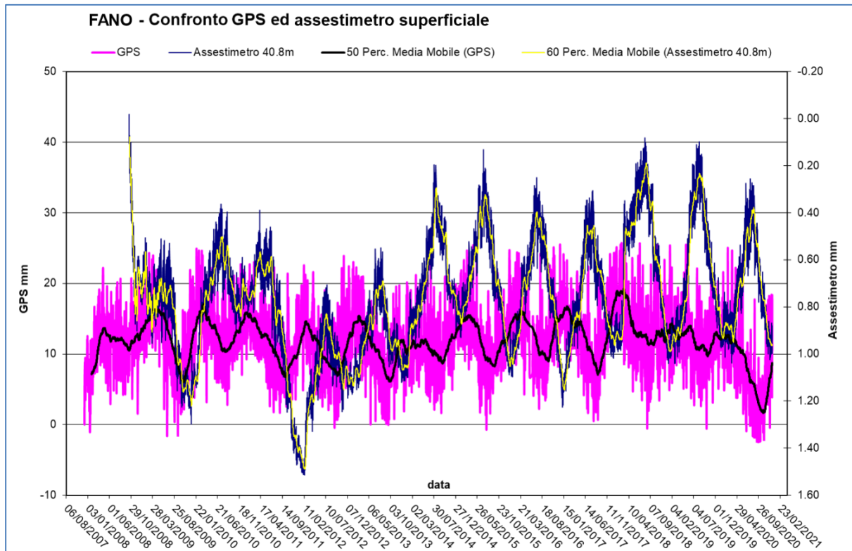
Figura 14B - Stazione EPSU di Fano: confronto fra misure CGPS vs. misure assestmetriche
