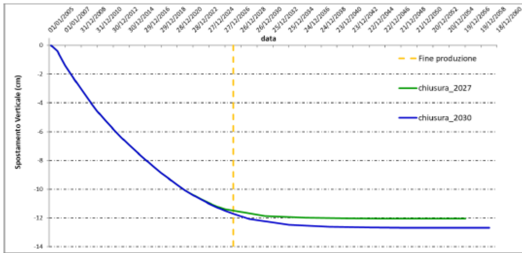
Figura 8 - Campo di Naide: evoluzione nel tempo del valore della subsidenza nel caso Do Nothing - caso base (fine produzione 2027) e Do Nothing – caso massimo (fine produzione 2030)
