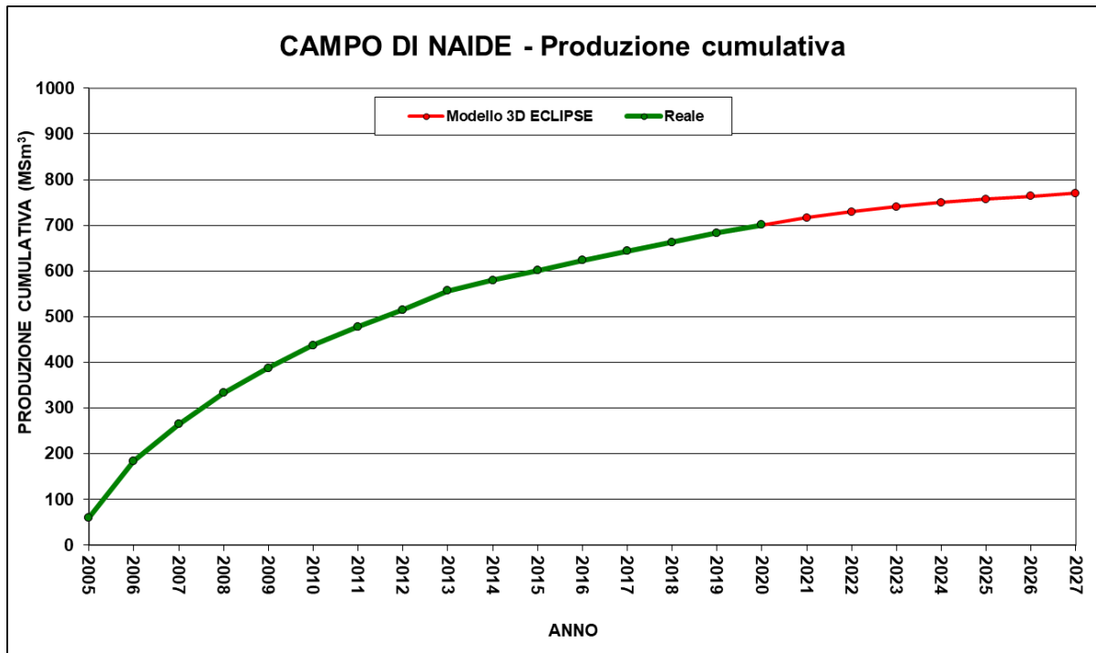
Figura 5 - Campo di Naide: grafico di produzione reale e da modello Eclipse 2021
