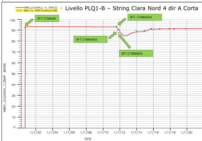
Figura 7 - Campo di Clara Nord: confronto fra i dati misurati di pressione statica e i profili di pressione calcolati da modello Eclipse 2017 - (livelli PLQ-HH1 e PLQ1-B)
