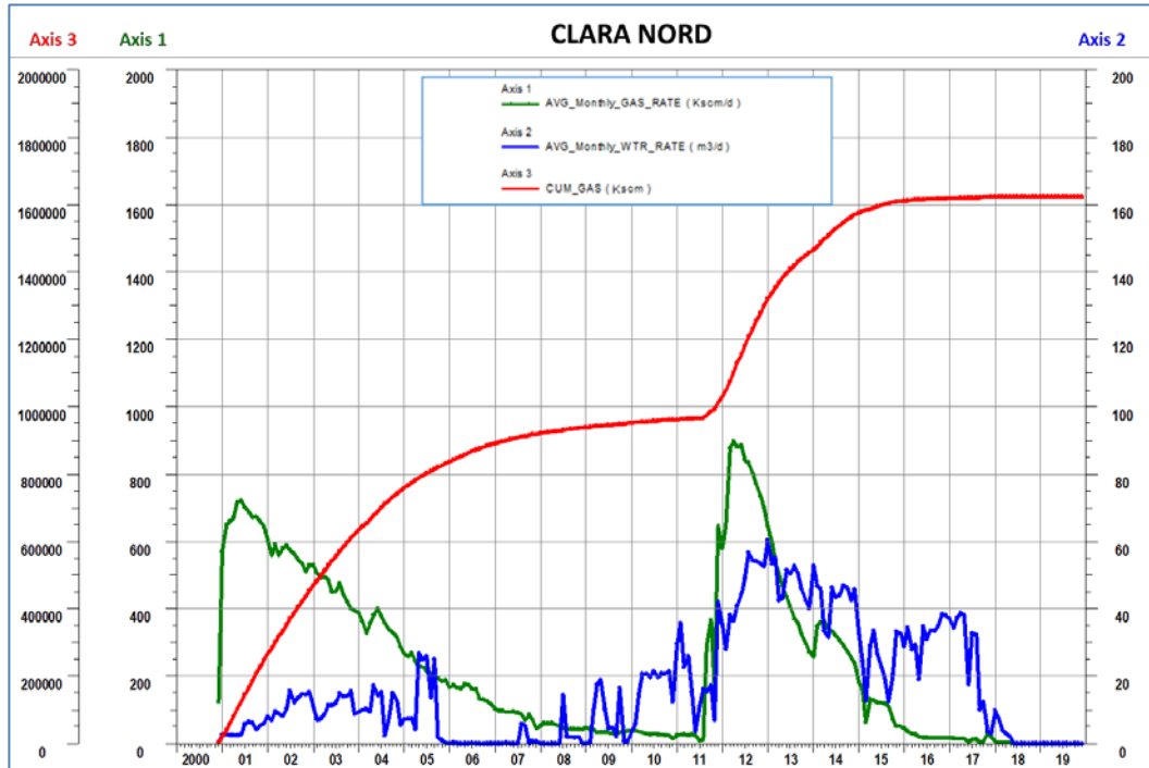
Figura 3 - Campo di Clara Nord: grafico di produzione storica
