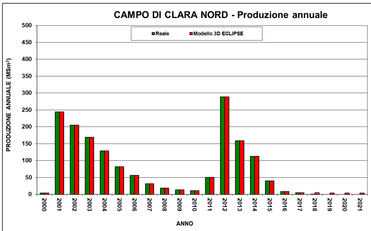
Figura 6 - Campo di Clara Nord: produzione (annuale) e da modello Eclipse 2017
