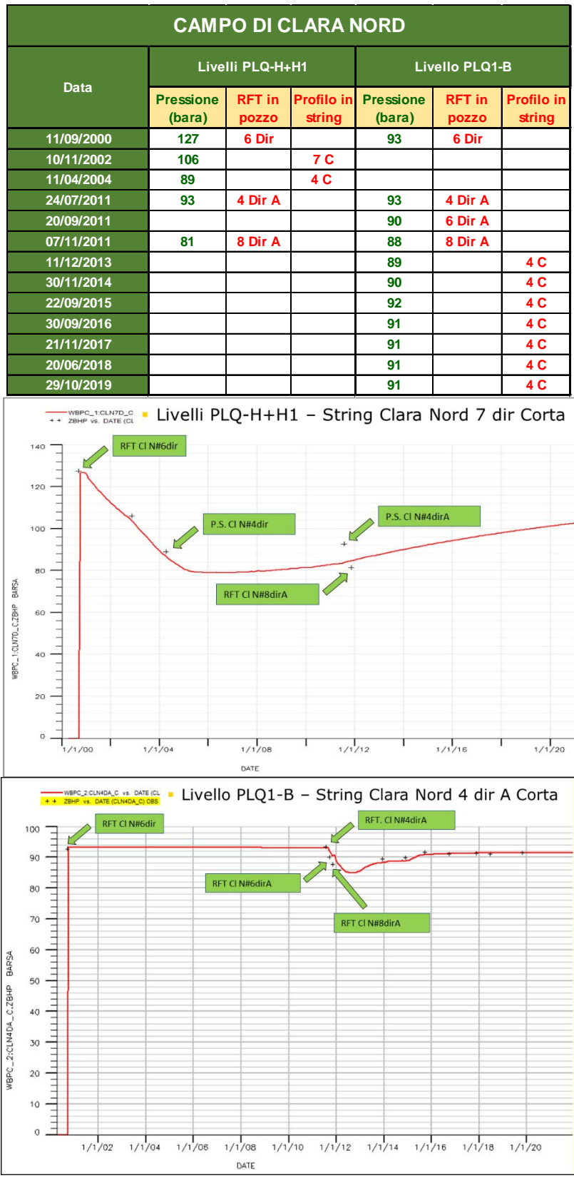
Figura 7 - Campo di Clara Nord: confronto fra i dati misurati di pressione statica e i profili di pressione calcolati da modello Eclipse 2017 - (livelli PLQ-HH1 e PLQ1-B)
