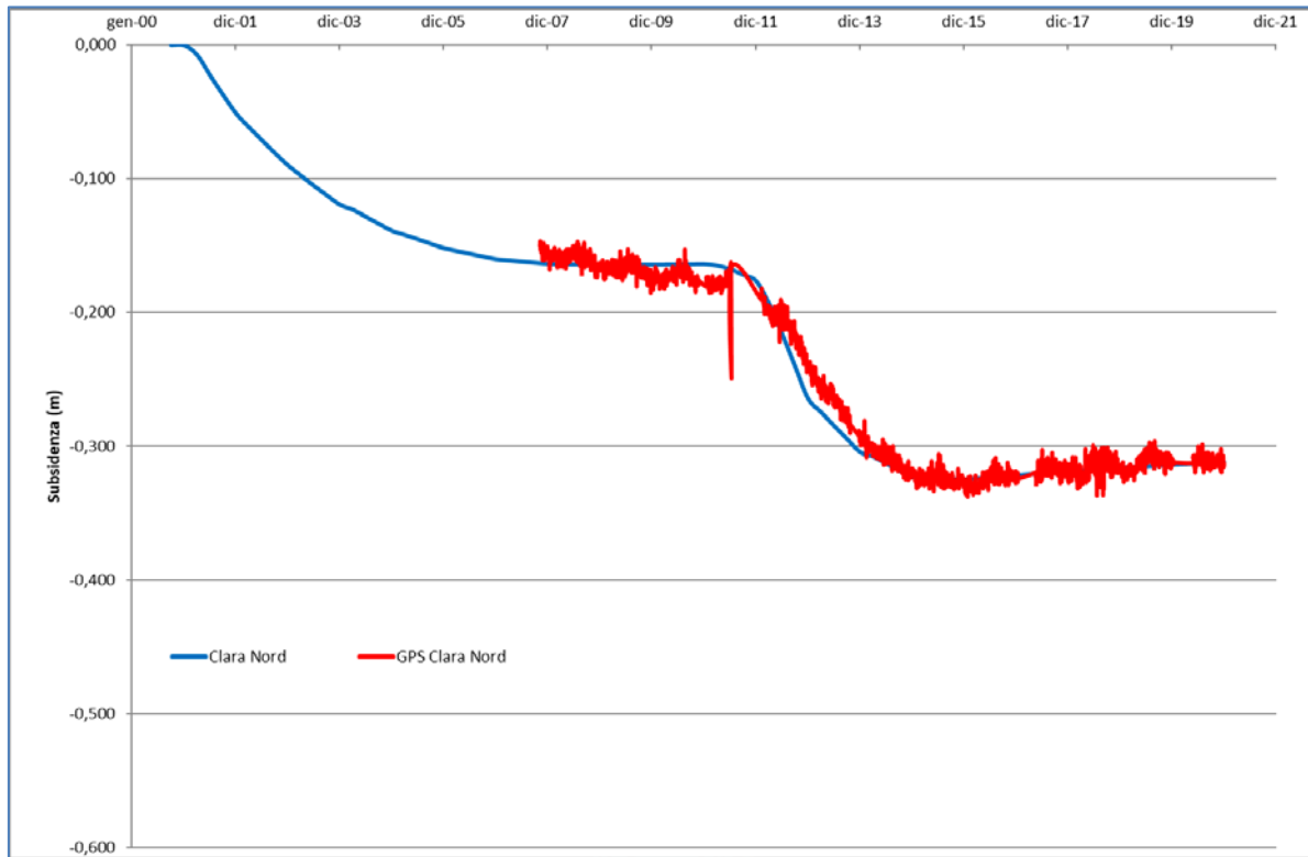
Figura 16 - Clara Nord: andamento della subsidenza misurata (CGPS in p.ma) vs. modello (scenario DN)
