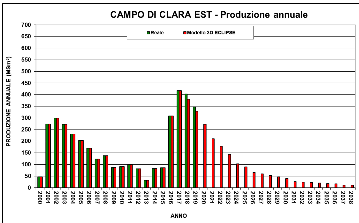
Figura 6 - Campo di Clara Est: produzione (annuale) reale e da modello Eclipse 2017
