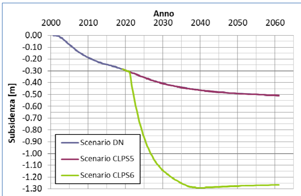
Figura 9 - Evoluzione temporale della subsidenza prevista nel punto di massimo di Clara Est
