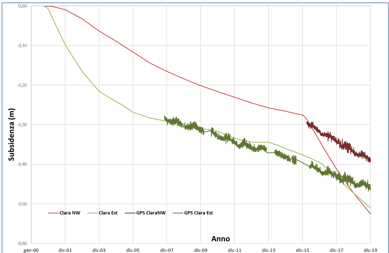
Figura 15 - Andamento della subsidenza misurata (CGPS Clara Est e Clara NW) comparata con la simulazione per il campo di Clara Est.
