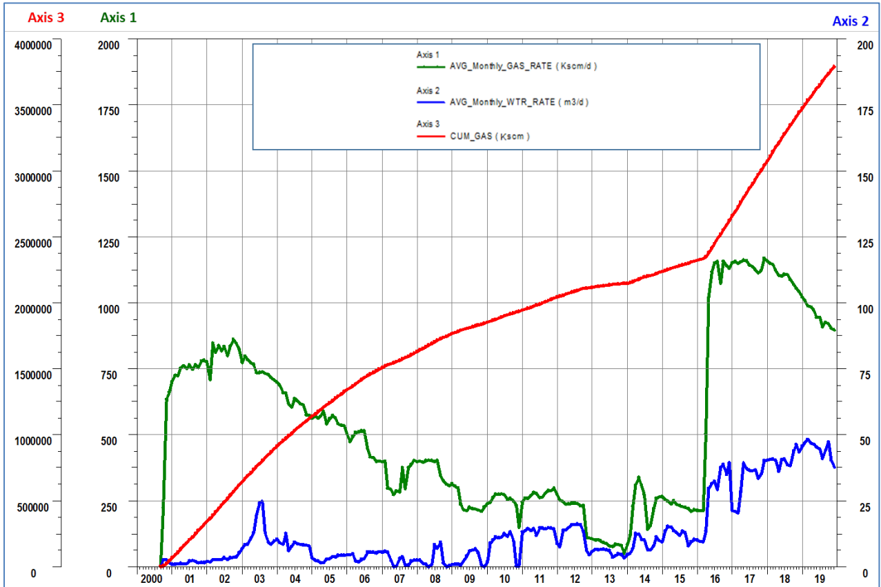
Figura 3 - Campo di Clara Est: grafico di produzione storica
