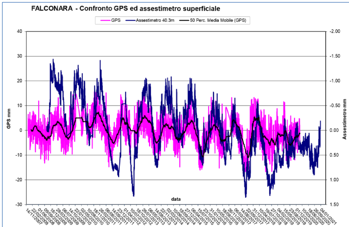
Figura 19B - Stazione EPSU di Falconara: confronto misure CGPS vs. misure assestimentriche
