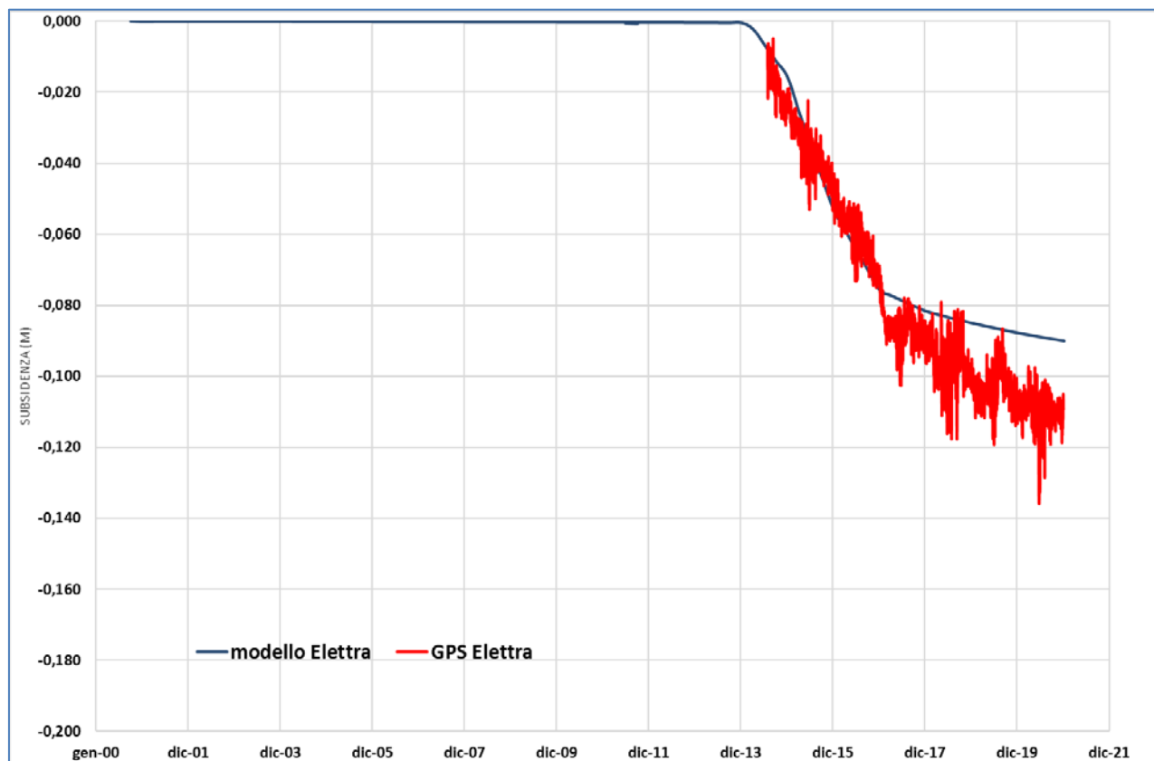
Figura 15 - Elettra: andamento della subsidenza misurata (CGPS in p.ma) vs. modello (scenario DN)
