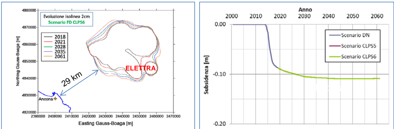
Figura 8 - Campo di Elettra: evoluzione nel tempo, rispettivamente della linea di iso-subsidenza dei 2 cm (scenario CLPS6) e della subsidenza prevista nel punto di massimo, per lo scenario CLPS6
