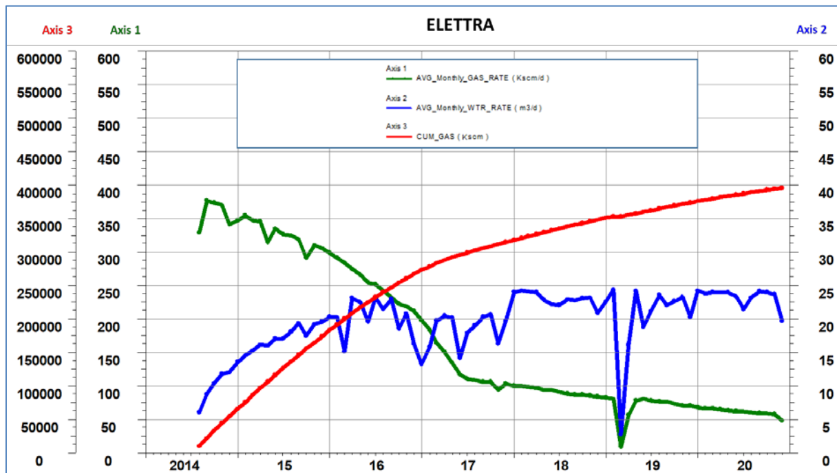
Figura 3 - Campo di Elettra: produzione storica
