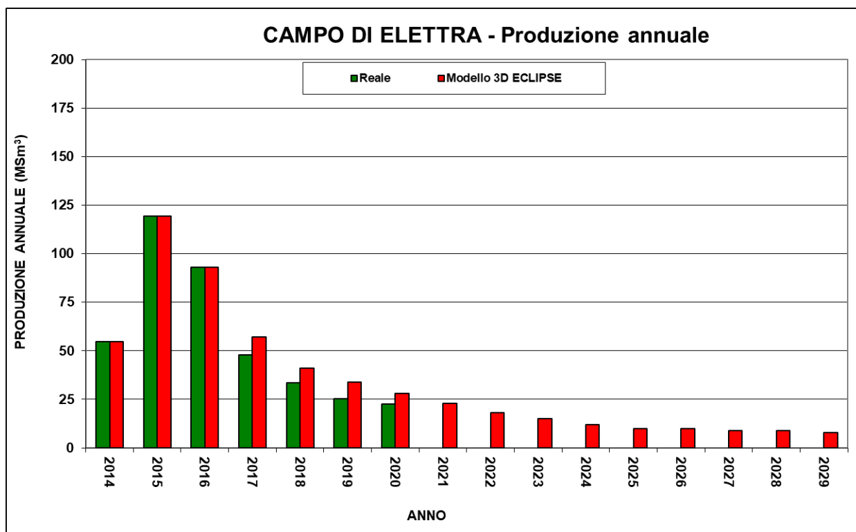
Figura 6 - Campo di Elettra: produzione (annuale) reale e da modello Eclipse 2017
