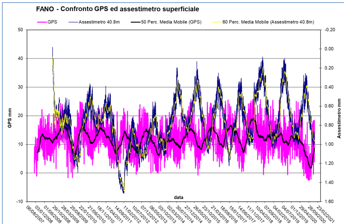
Figura 14B - Stazione EPSU di Fano: confronto fra misure CGPS vs. misure assestimentriche
