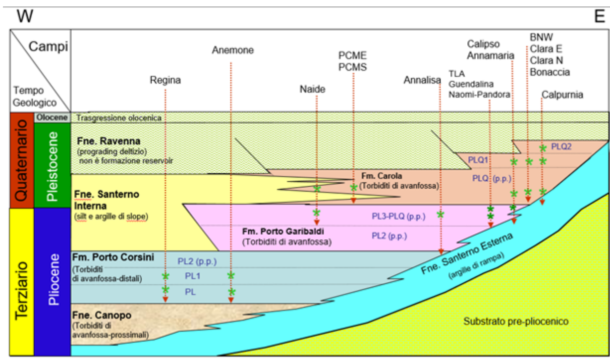
Figura 2 - Bacino Adriatico settentrionale: esempio di schema dei rapporti stratigrafici e dei principali reservoir (*) sviluppati dai campi
