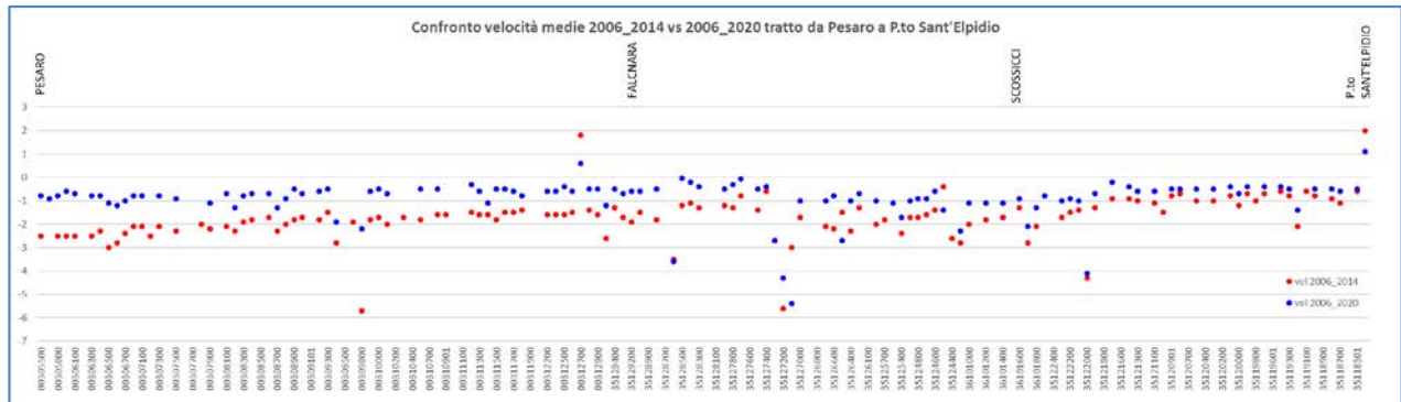
Figura A – Tratta Pesaro - Sant’Elpidio: velocità medie di subsidenza nei periodi 2006-2014 e 2006-2020
