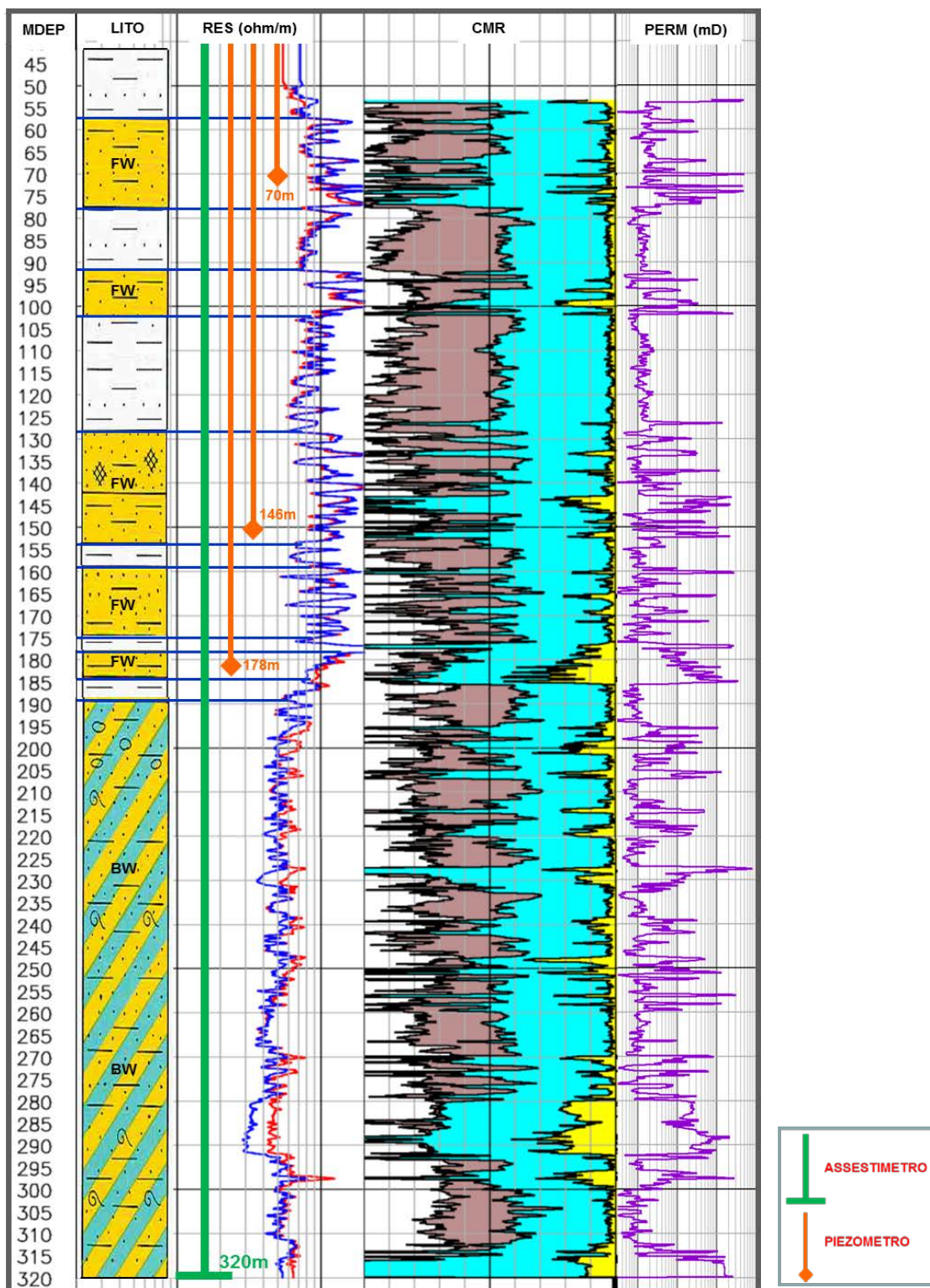
Figura 5B - Litologia dei terreni monitorati dalla stazione EPSU di Rubicone
