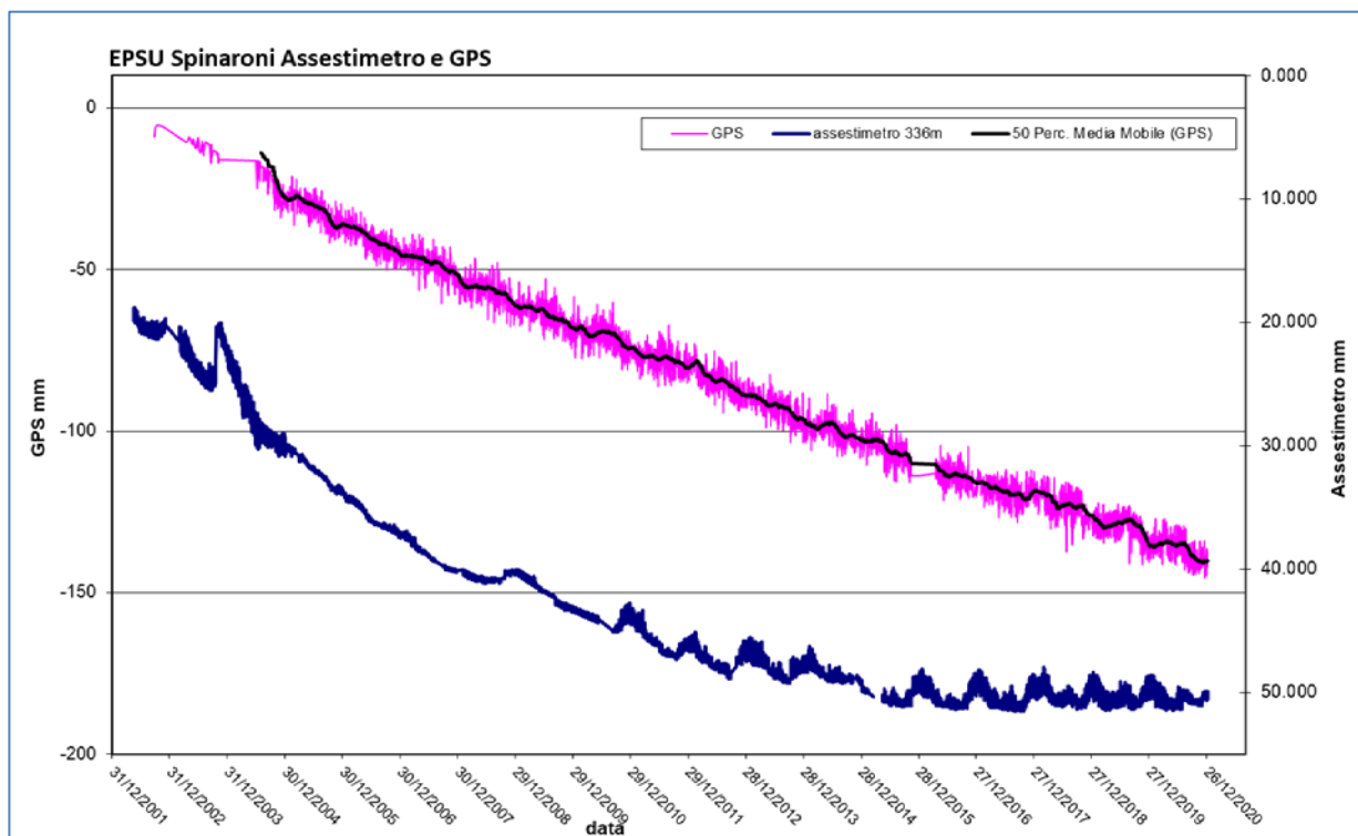
Figura 12B - Confronto fra misure da CGPS vs. misure di compattazione (assessimetro della stazione EPSU di Spinaroni)
