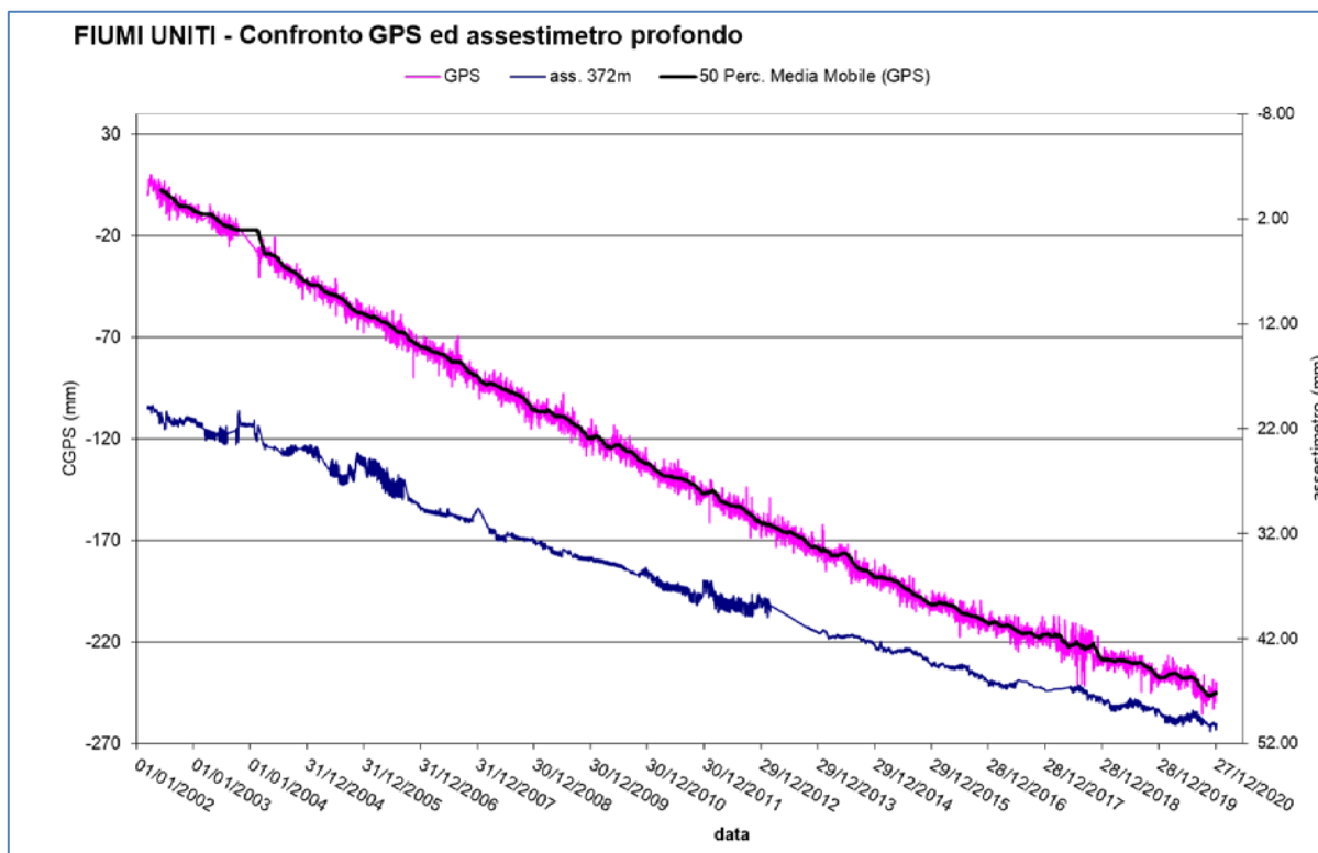
Figura 19B - Confronto fra misure da CGPS vs. misure di compattazione (Assestometro profondo della stazione EPSU di Fiumi Uniti)
