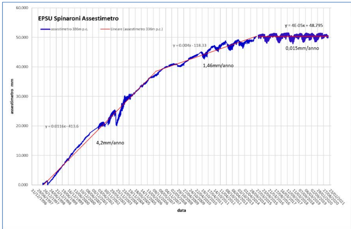
Figura 10B – Trend curva di compattazione dell’assestimetro della stazione EPSU di Spinaroni
