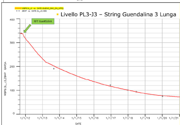
Figura 7 - Campo di Guendalina: confronto tra dati di pressione da profili statici e modello Eclipse 2018 (liv. PL3-I1 e PL3-J3)
