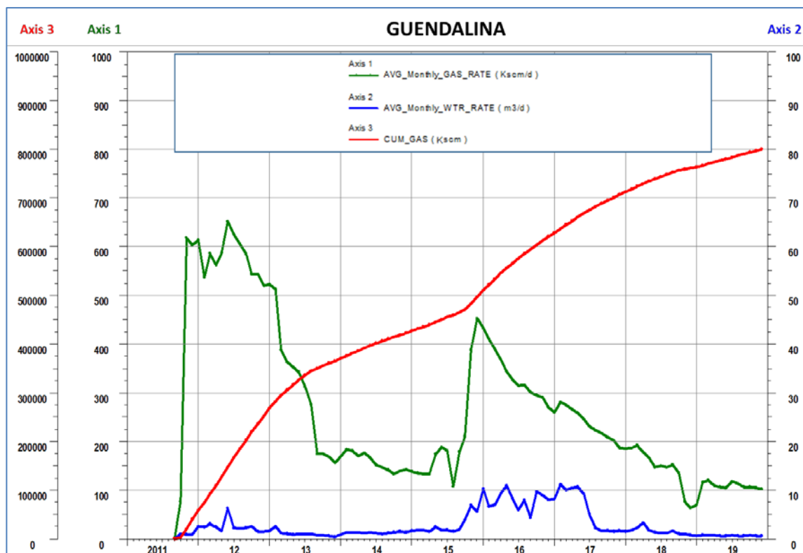
Figura 3 - Campo di Guendalina: produzione storica
