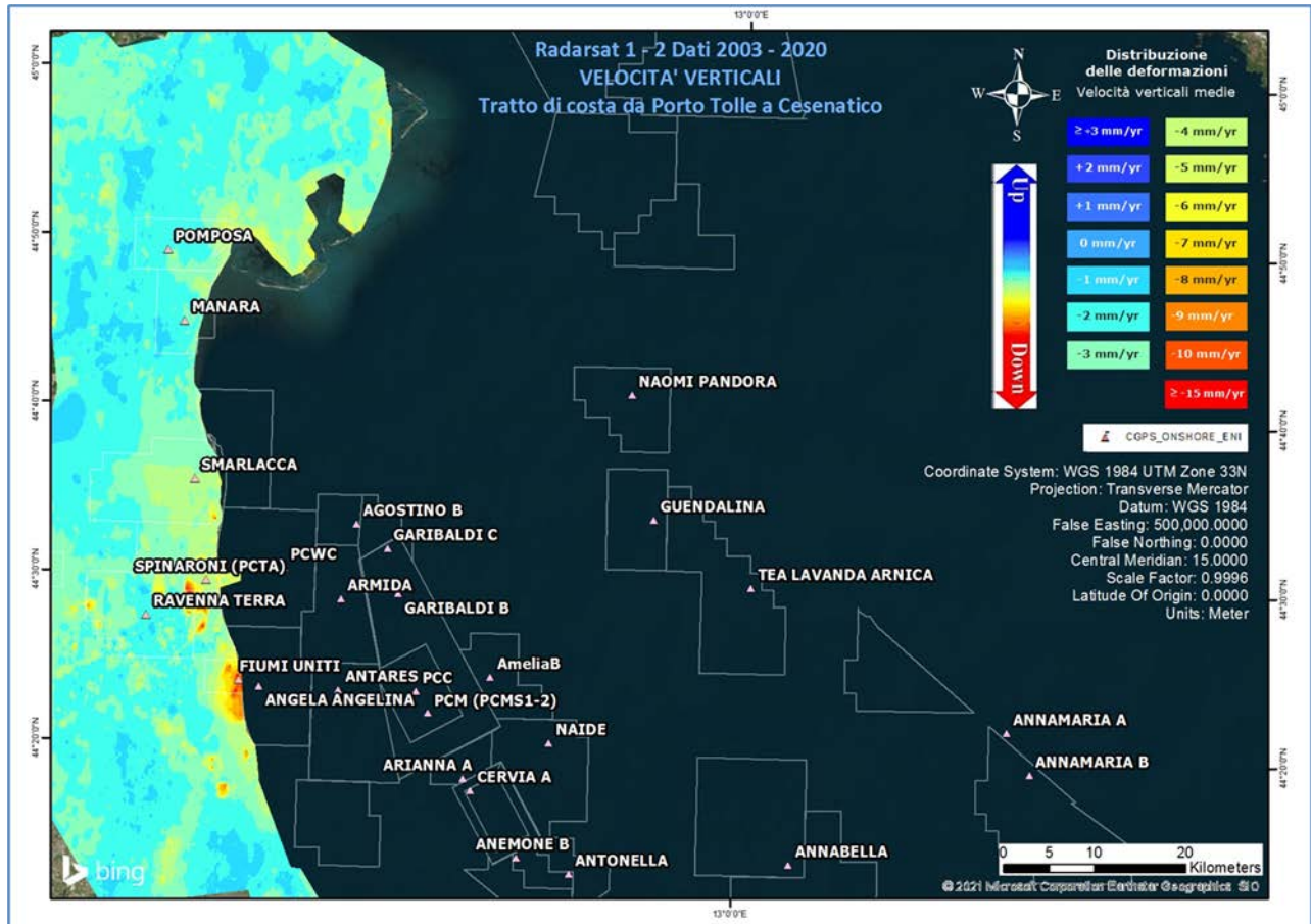
Figura 13 - Campo di Guendalina: analisi dei dati SAR dal 2003 al 2020.
