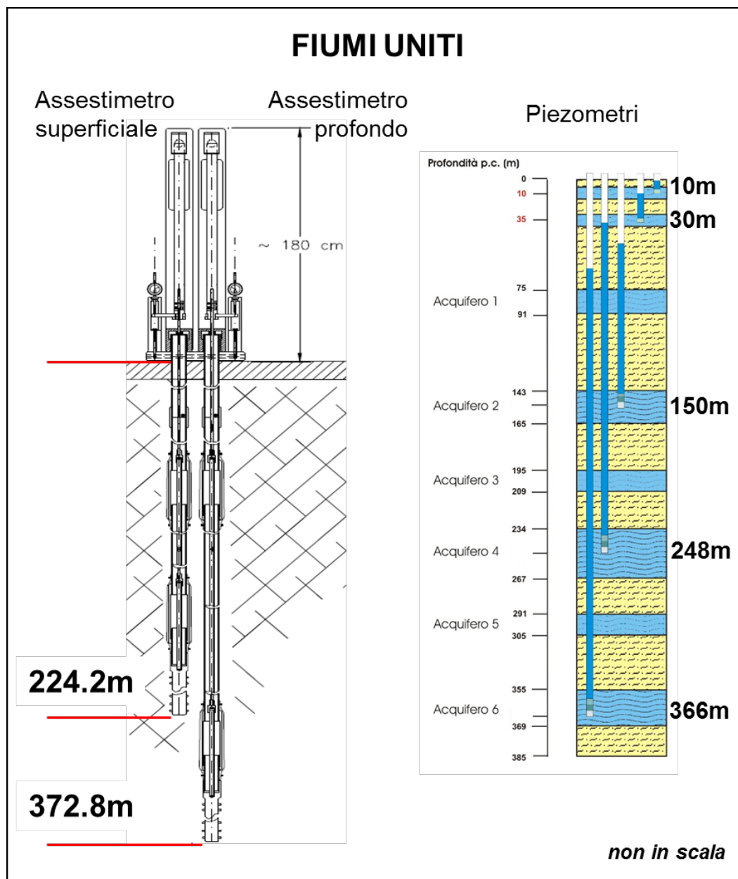
Figura 13B - Schema della stazione EPSU di Fiumi Uniti. Le profondità dei piezometri sono riferite alla quota centrale del tratto filtrante
