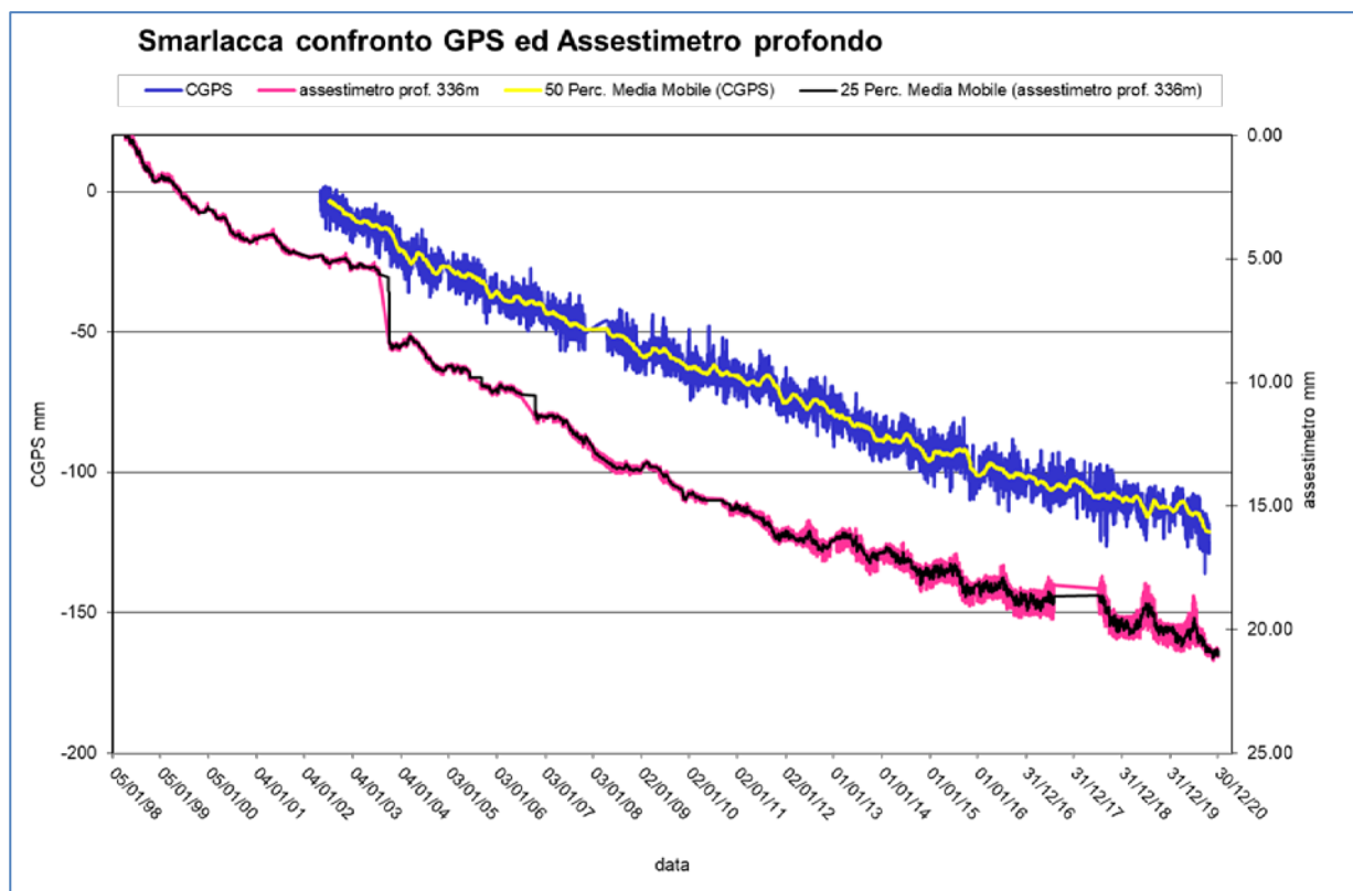
Figura 7B - Confronto fra misure da CGPS vs. misure di compattazione (assestimetro profondo della stazione EPSU di Smarlacca)
