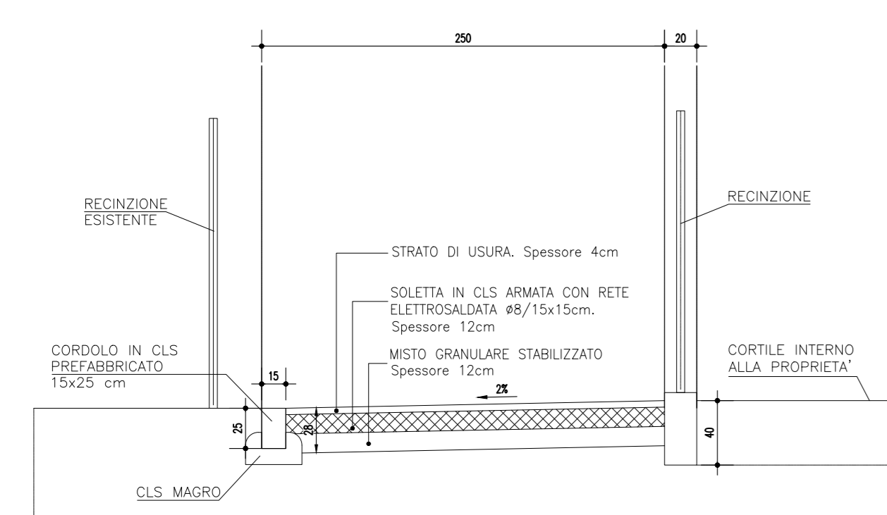
SEZIONE TIPO -3- 1:25
