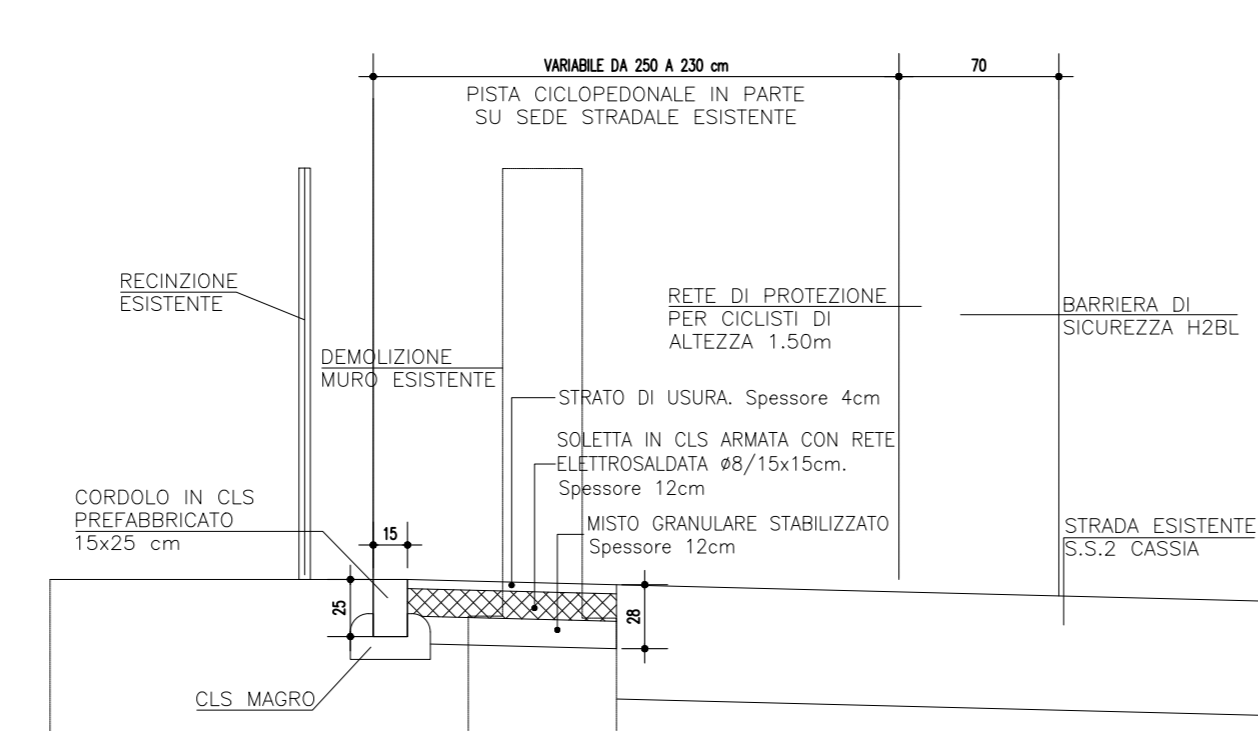
SEZIONE TIPO -4- 1:25
