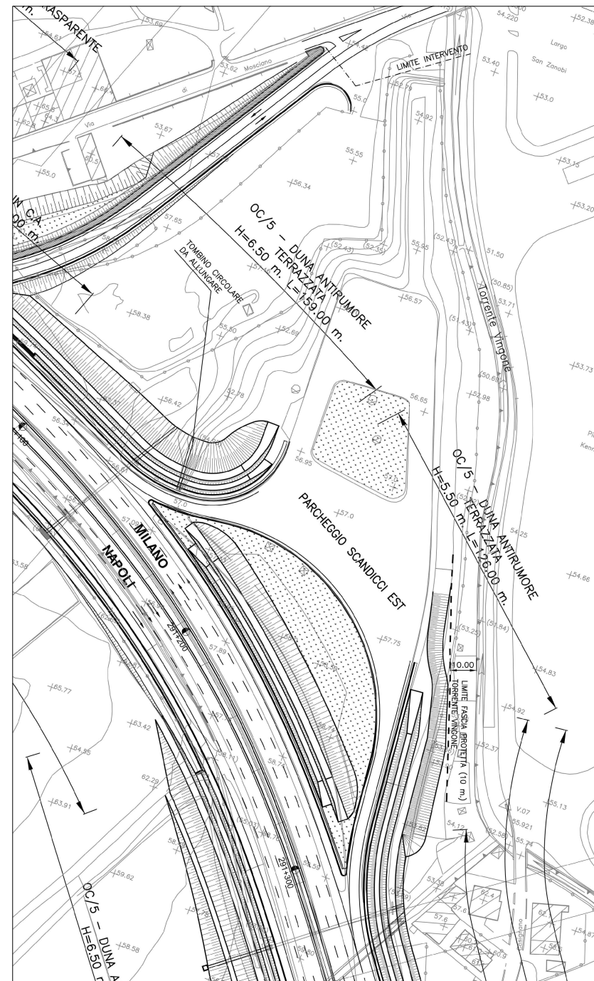
PLANIMETRIA PROGETTO ESECUTIVO
