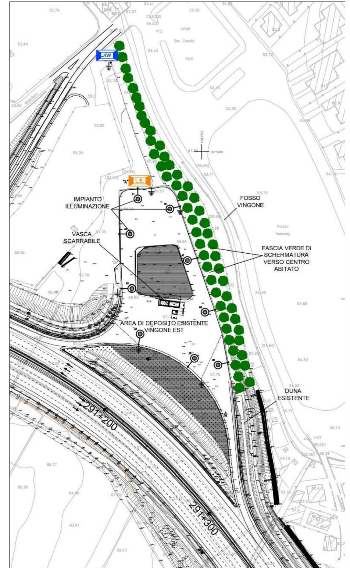
PLANIMETRIA DI PROGETTO OPERE A VERDE
