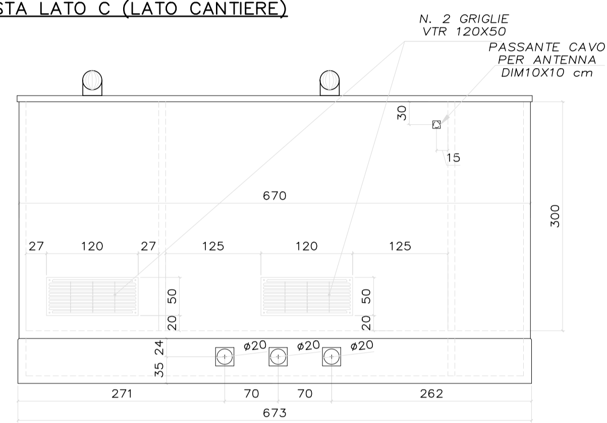
VISTA LATO C (LATO CANTIERE)
