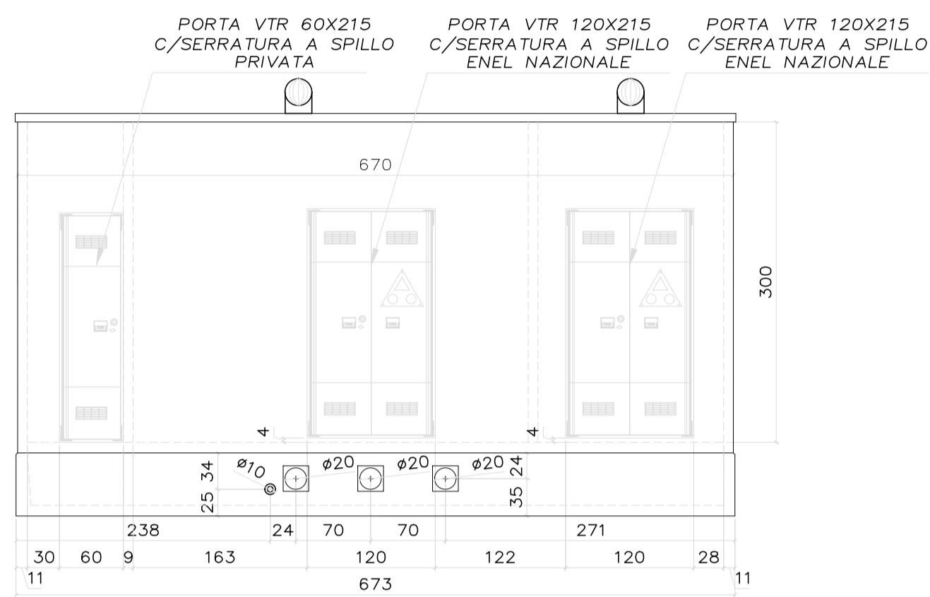
VISTA LATO A (LATO ACCESSO PUBBLICO)
