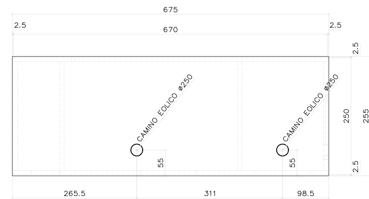
PIANTA COPERTURA
