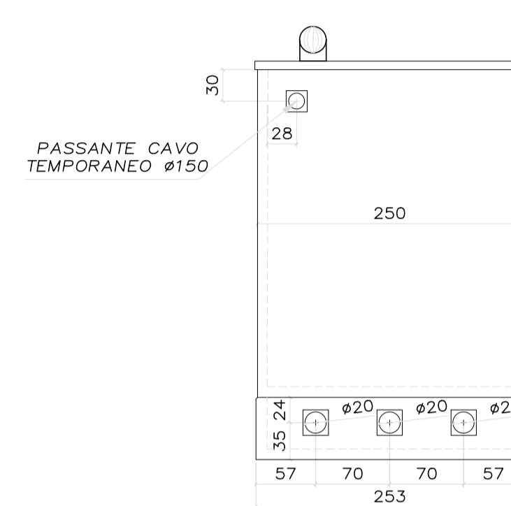
VISTA LATO D
