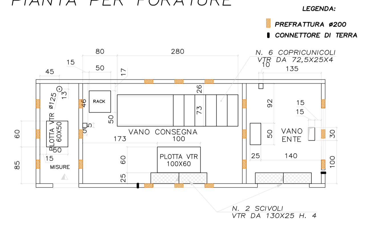
PIANTA PER FORATURE
