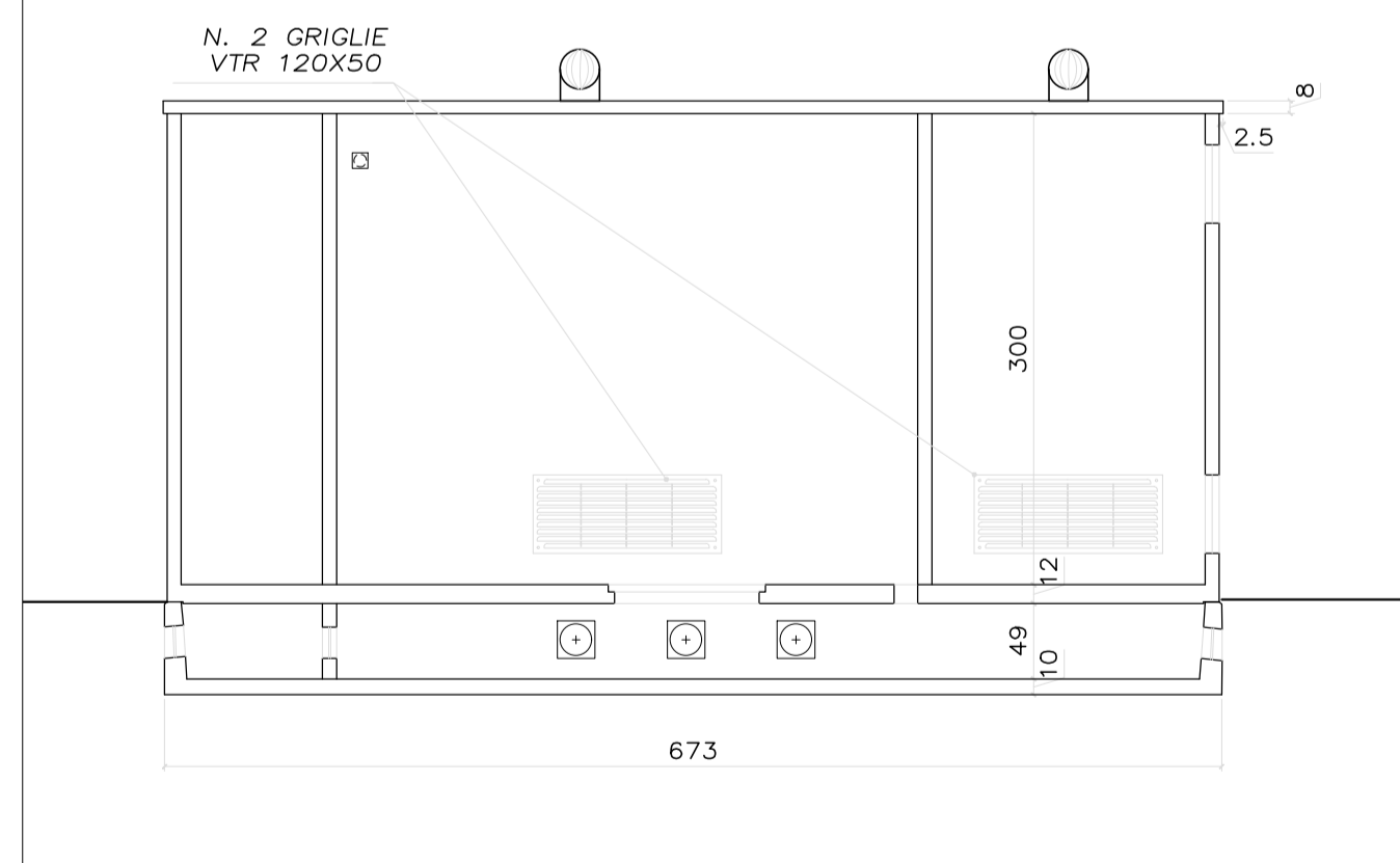
SEZ. X-X
