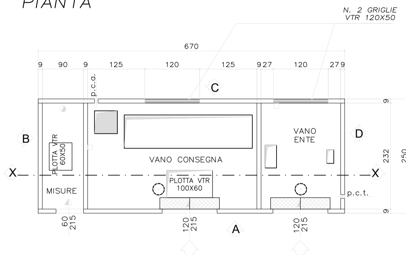
PIANTA
