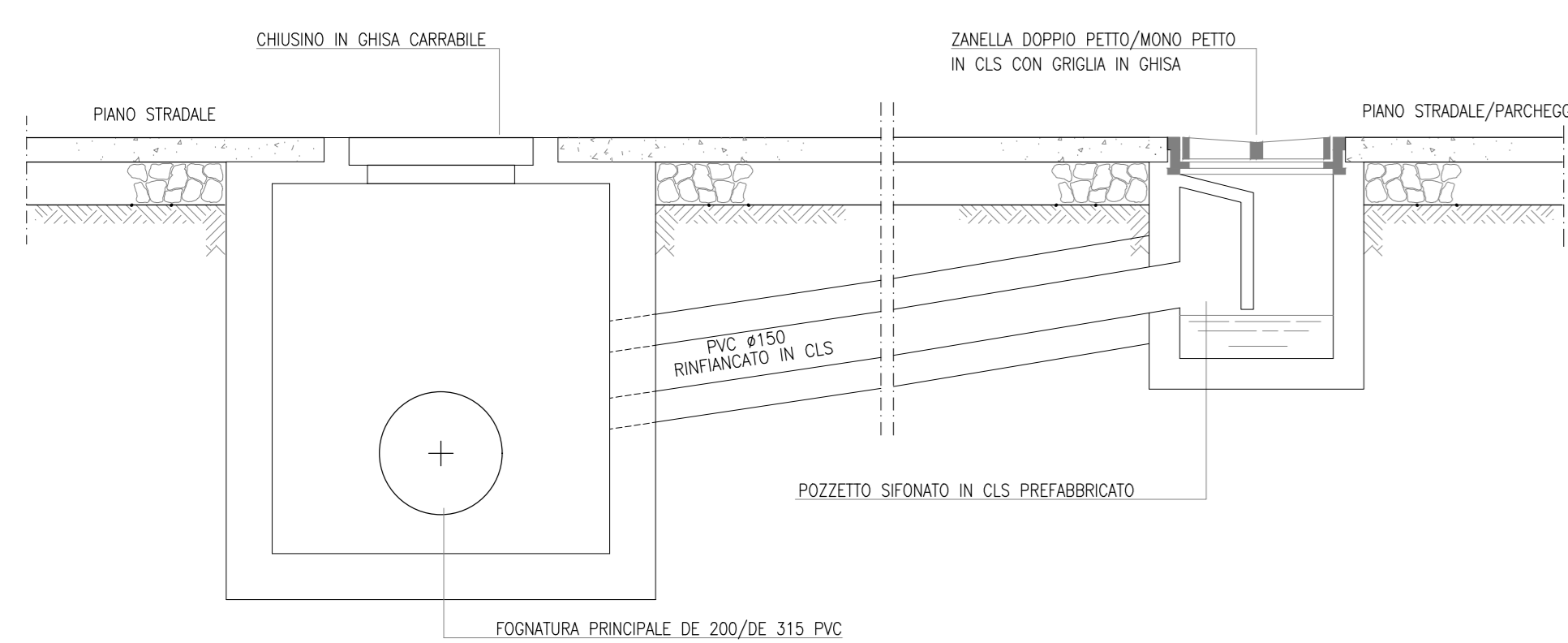
SEZIONE A-A 1:20
