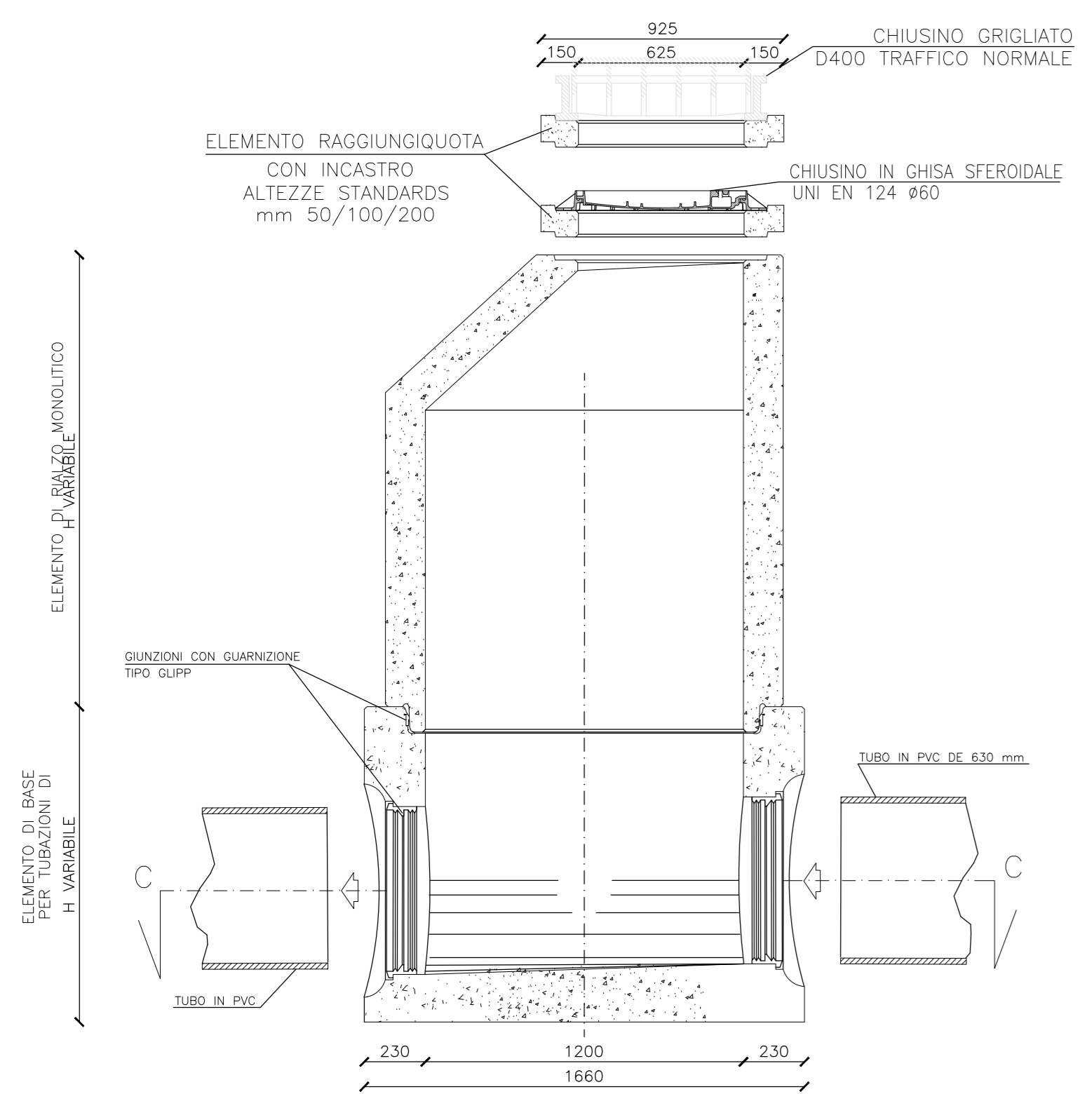
SEZIONE A-A 1:20
