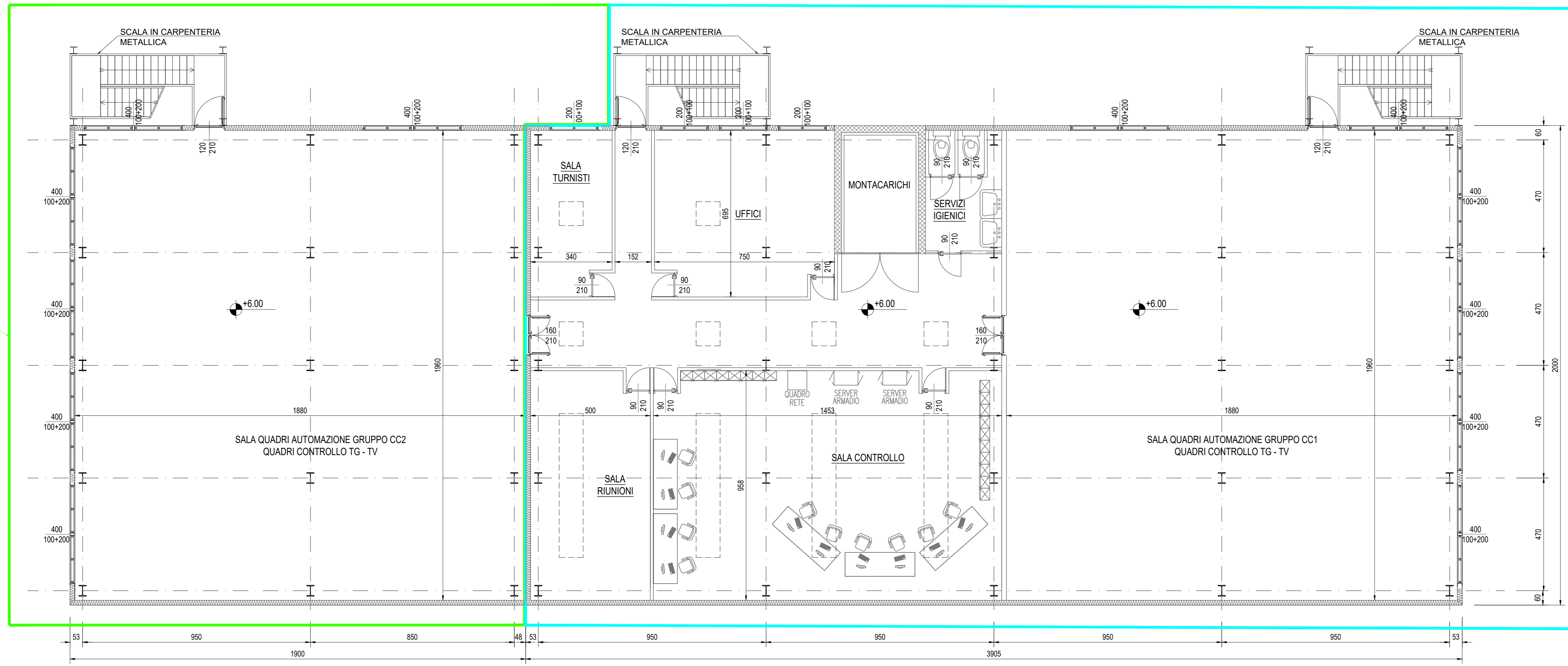
EDIFICIO ELETTRICO PIANTA A PIANO PRIMO Scala: 1:100
