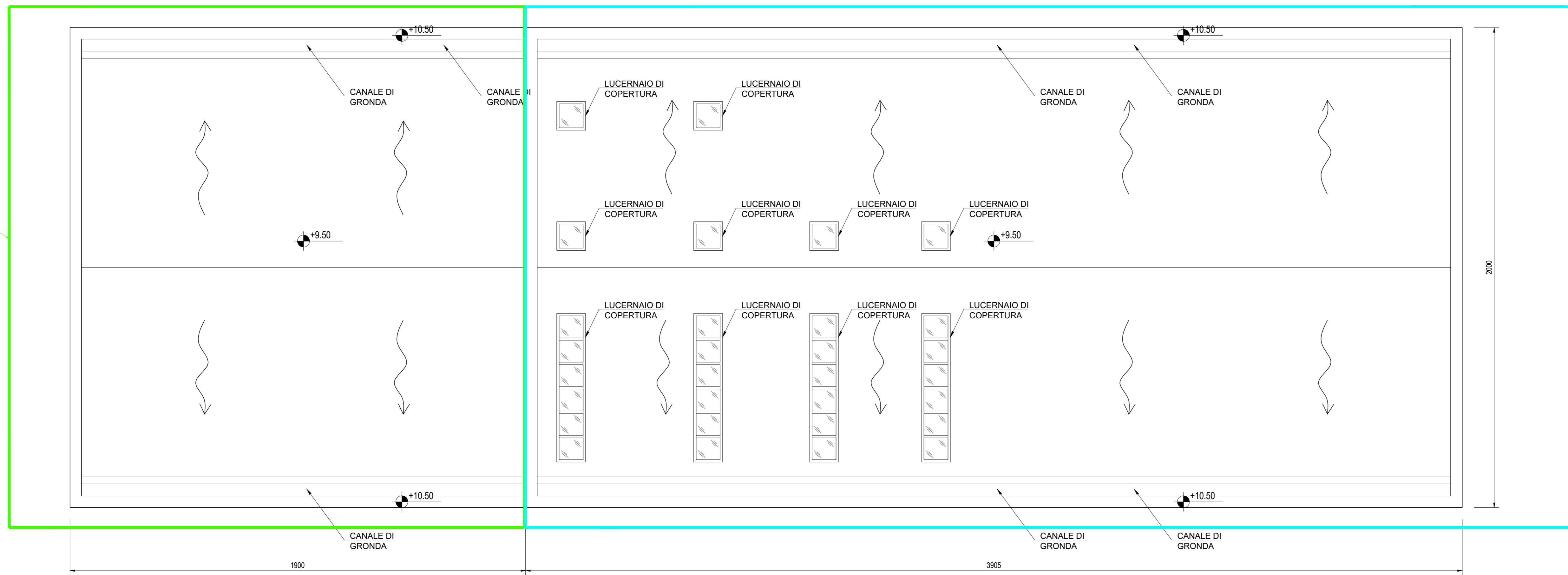
EDIFICIO ELETTRICO PIANTA COPERTURA Scala: 1:100
