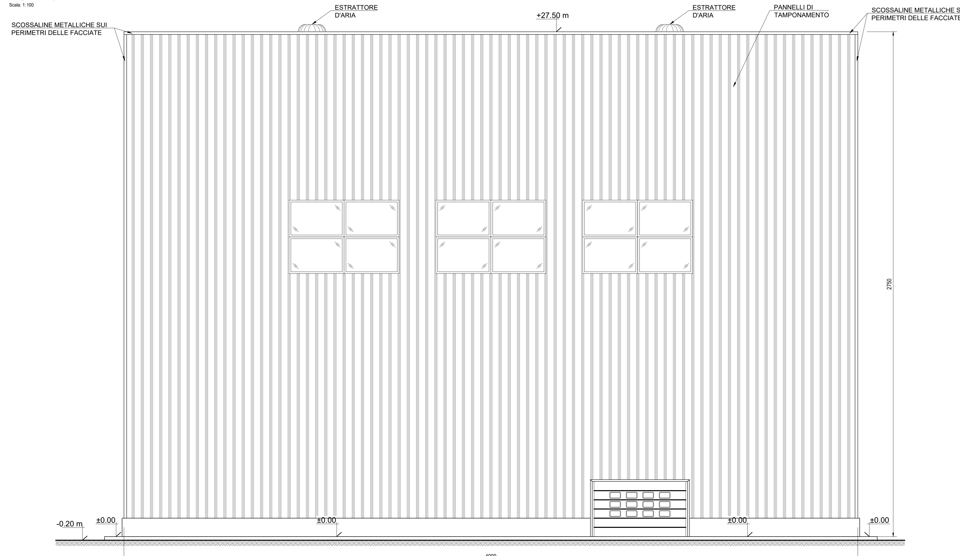
PROSPETTO VISTA B Scala 1:100
