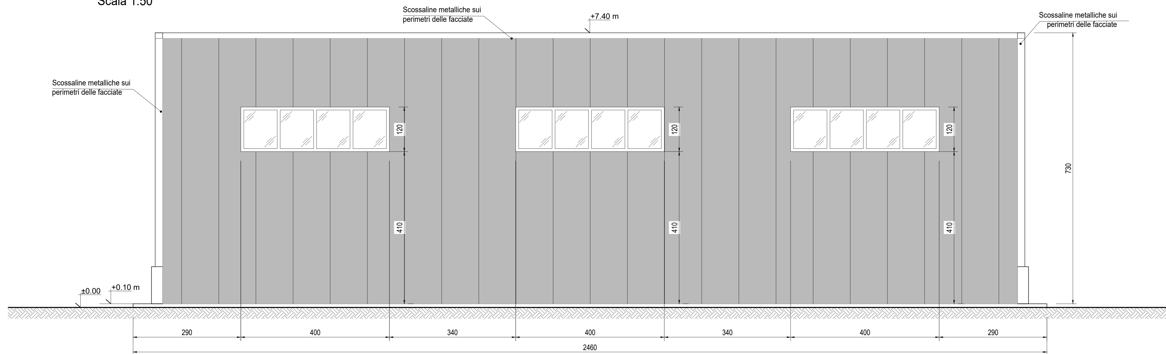
VISTA B Scala 1:50
