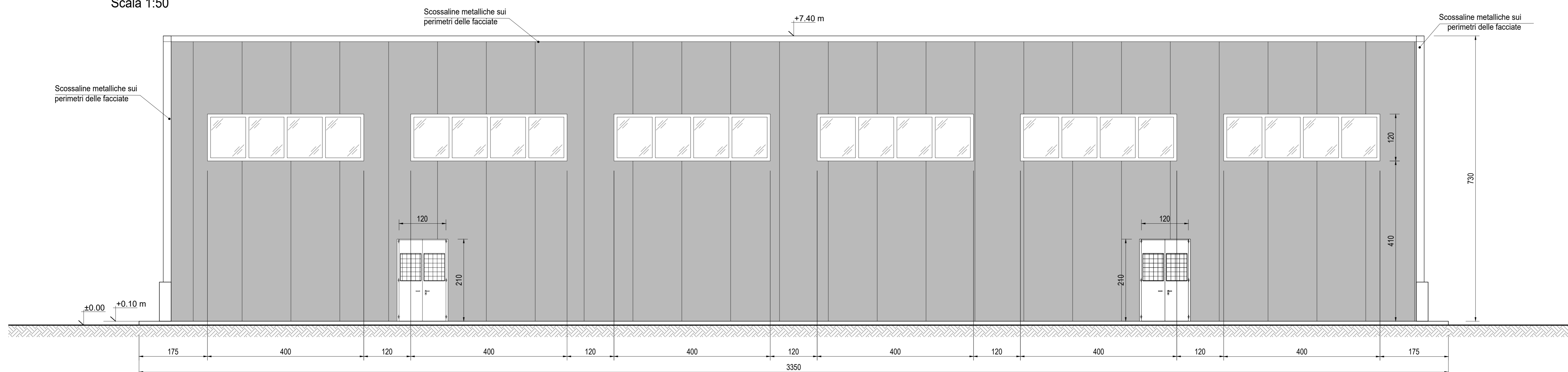
VISTA C Scala 1:50
