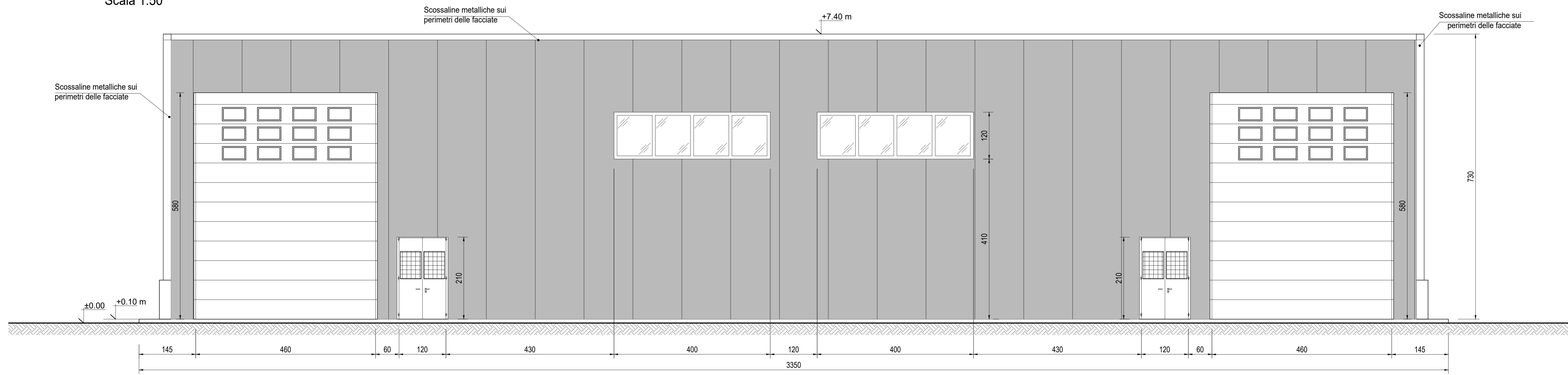
VISTA A Scala 1:50
