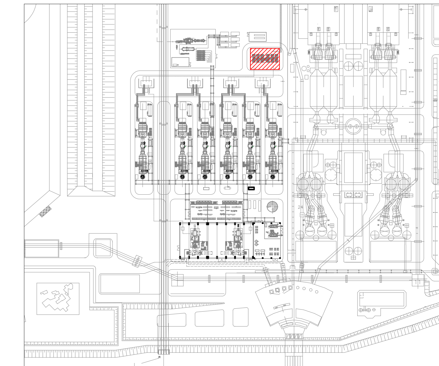
PLANIMETRIA GENERALE
