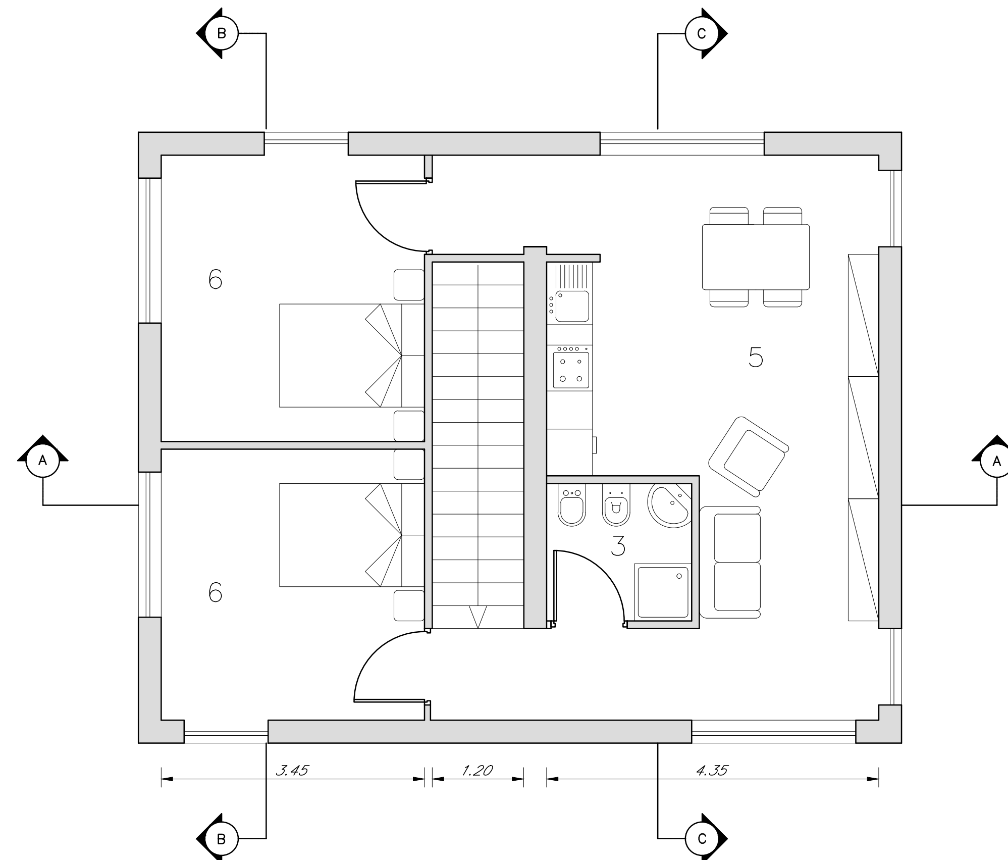
PIANTA PRIMO PIANO SCALA 1:50
