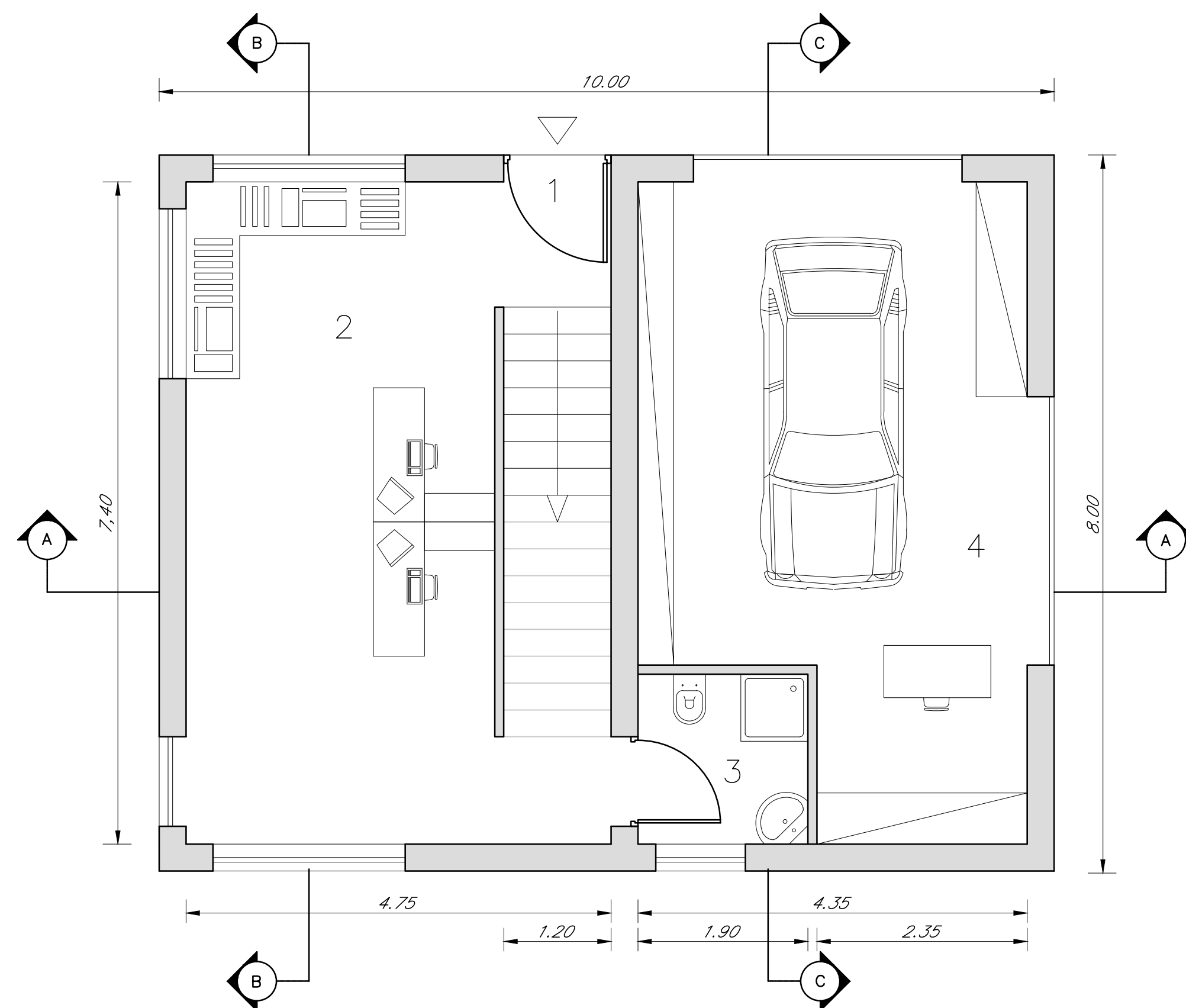
PIANTA PIANO TERRA SCALA 1:50
