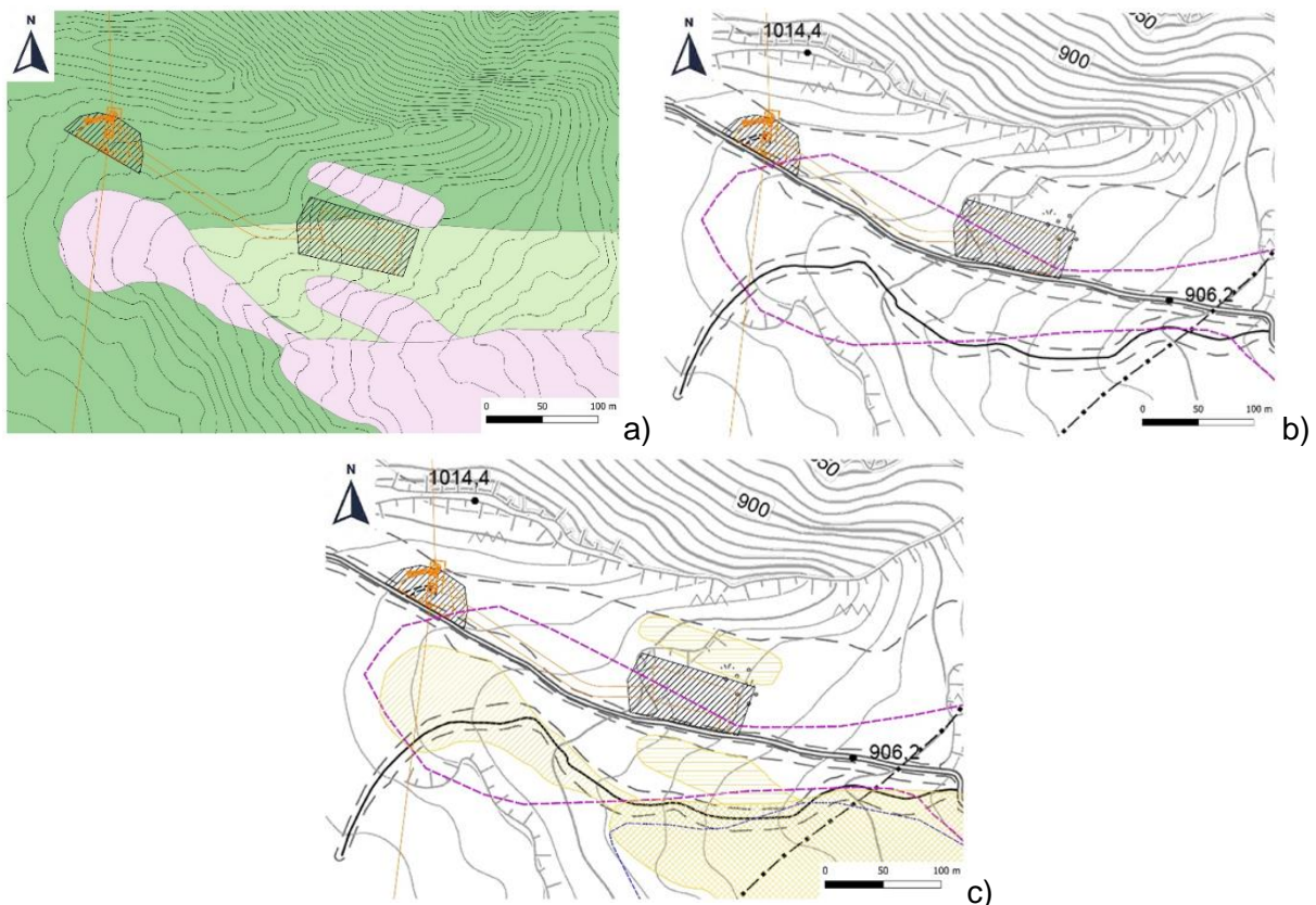
Figura 10 - Stralci cartografici dell'area della torre piezometrica: a) carta geologica; b) carta delle PG3 del P.A.I.; c) carta delle frane compressive
