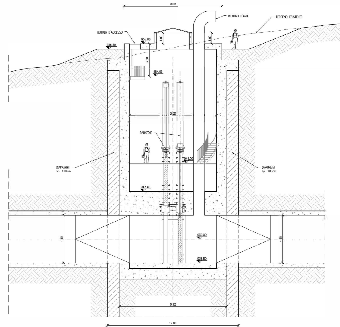
SEZIONE A-A
