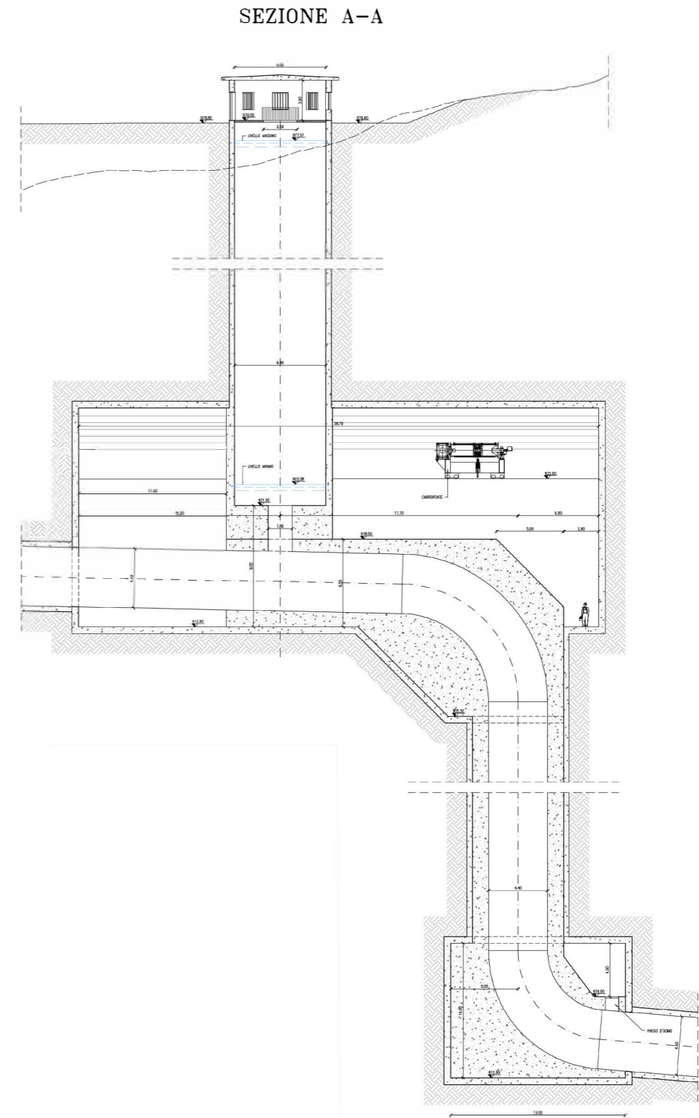
FIGURA 4.4 POZZO PIEZOMETRICO PLANIMETRIA E SEZIONI
