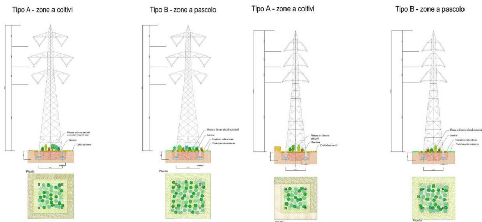
Figura 59. Interventi di mitigazione presso i sostegni previsti.
