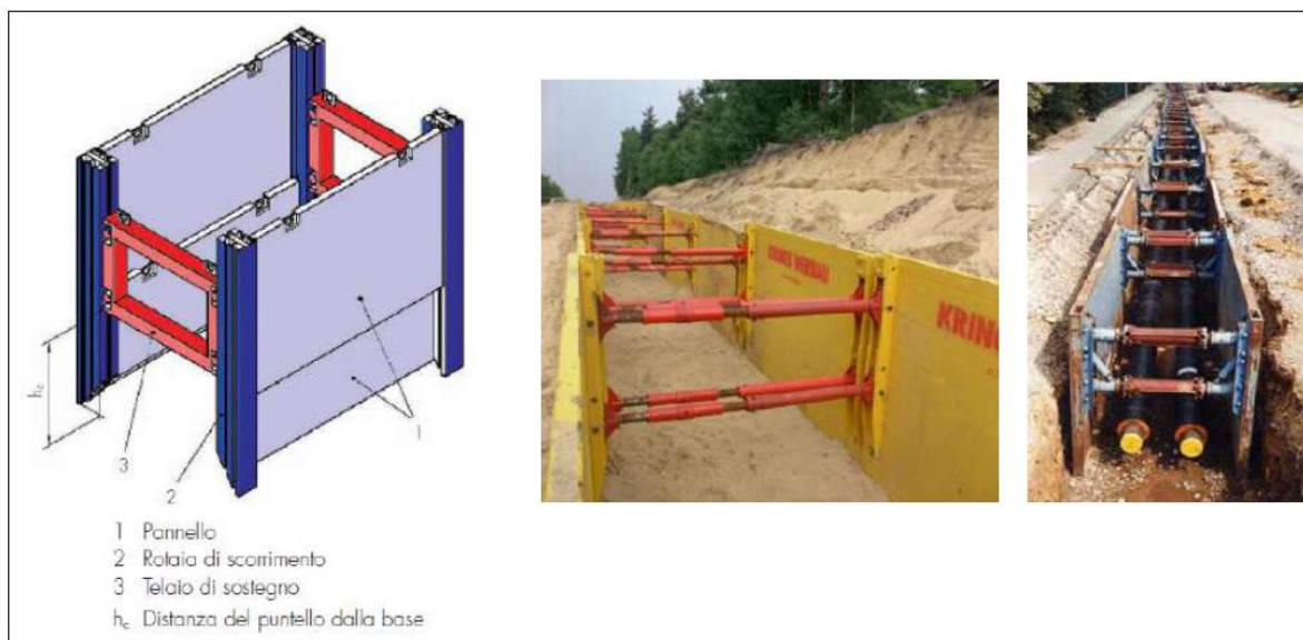
Fig. 6.1.6/a: Opere provvisorie - sbadacchiature con legname e sistemi di puntellazione per scavi
