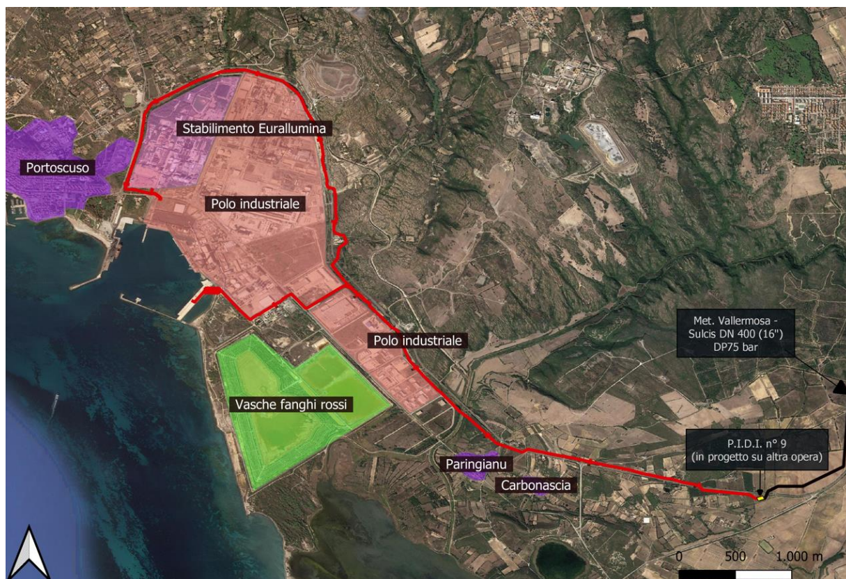
Fig. 3.3/A – Inserimento dei tracciati di progetto nel contesto territoriale
