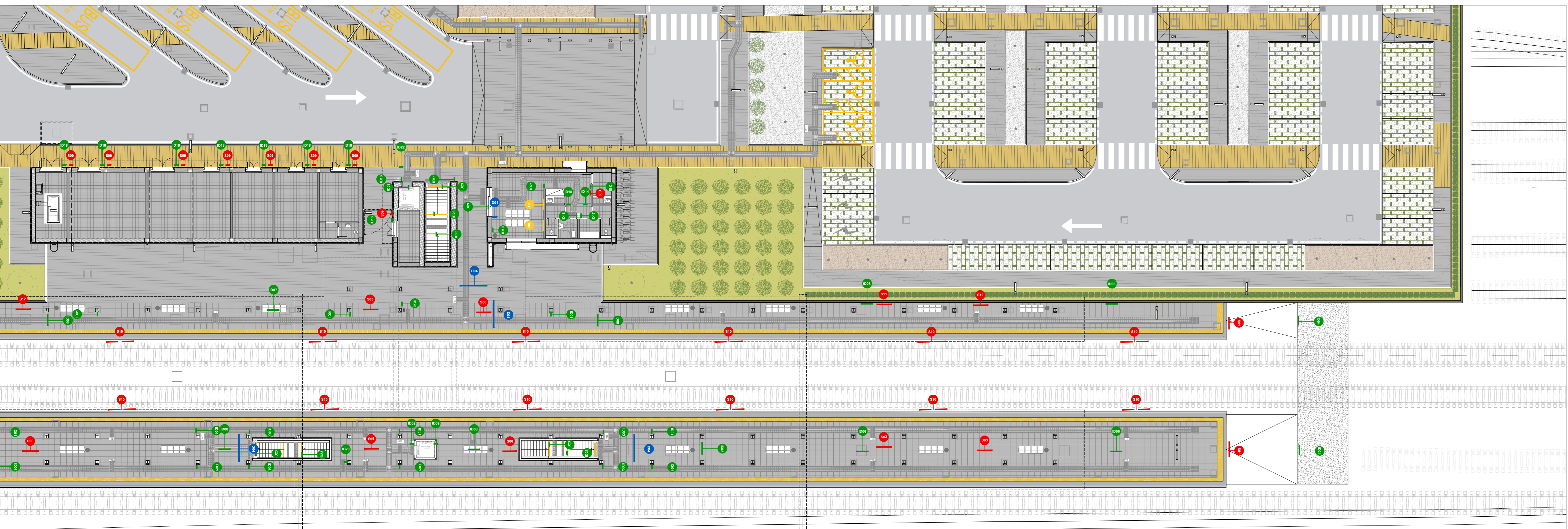
B PIANTA QUOTA BANCHINA STRALCIO B scala 1:200
