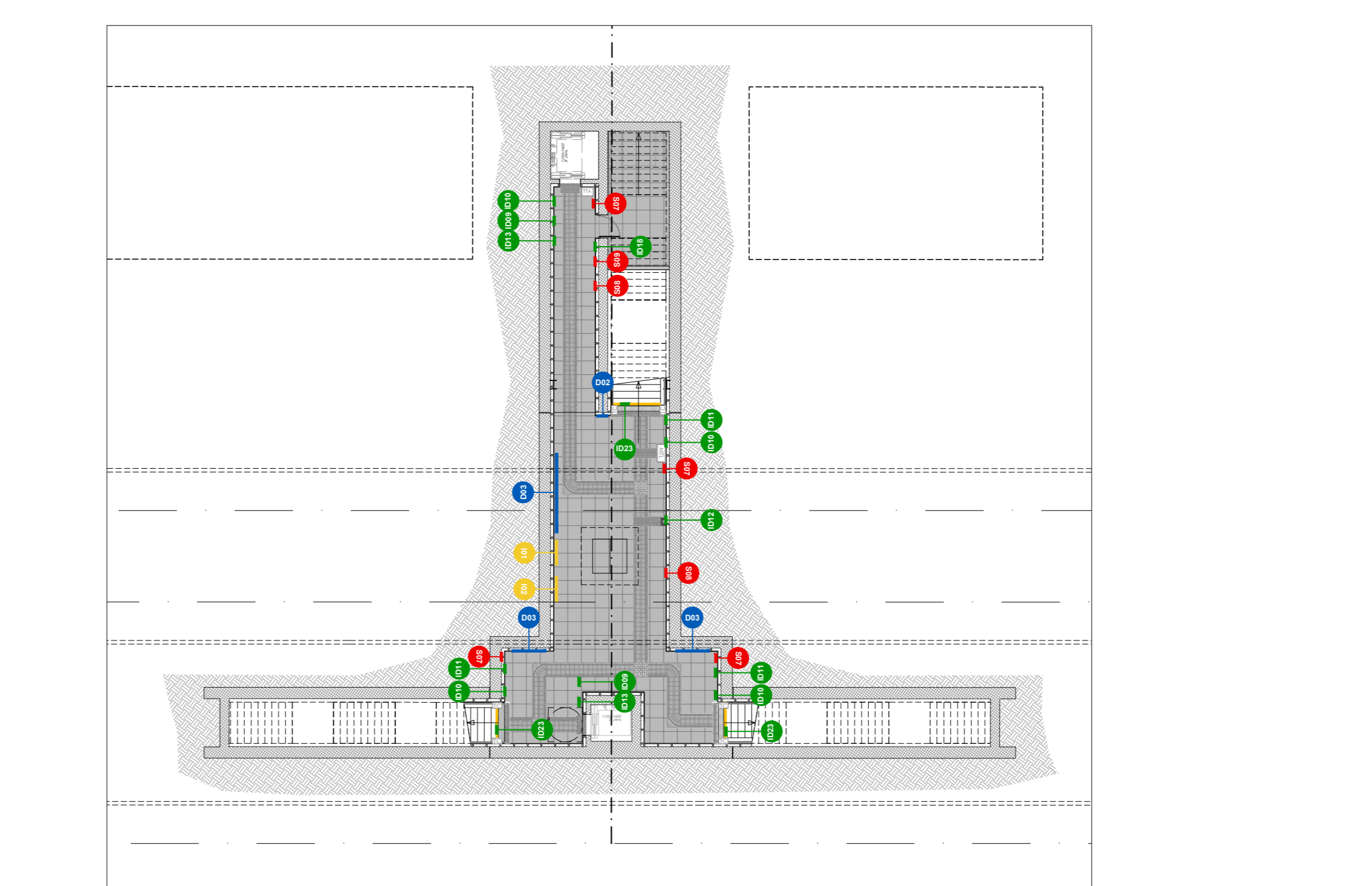
PIANTA QUOTA SOTTOPASSO scala 1:200
