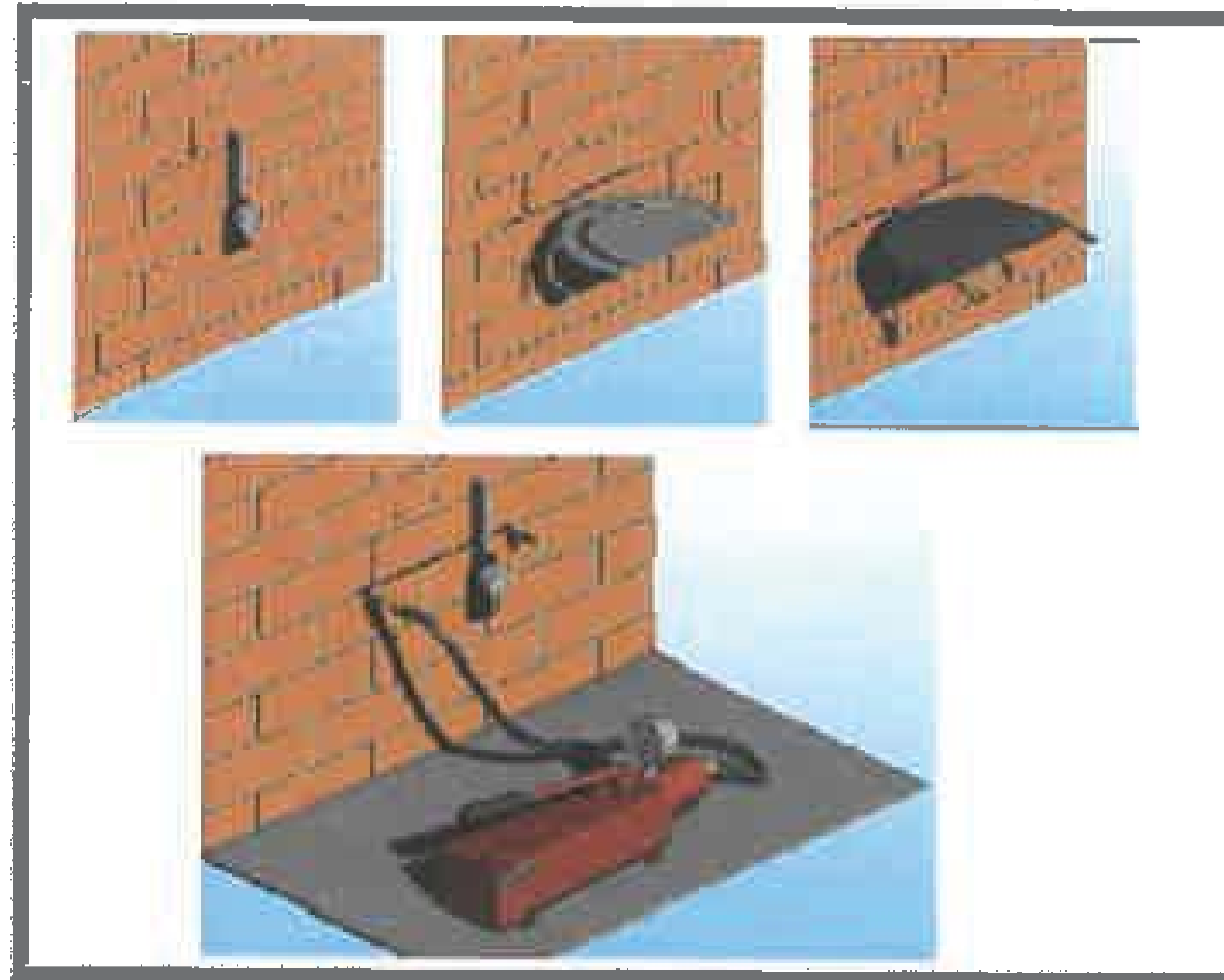
Fig. A.2.h.b -Esecuzione del taglio, inserimento del martinetto, misura degli spostamenti
