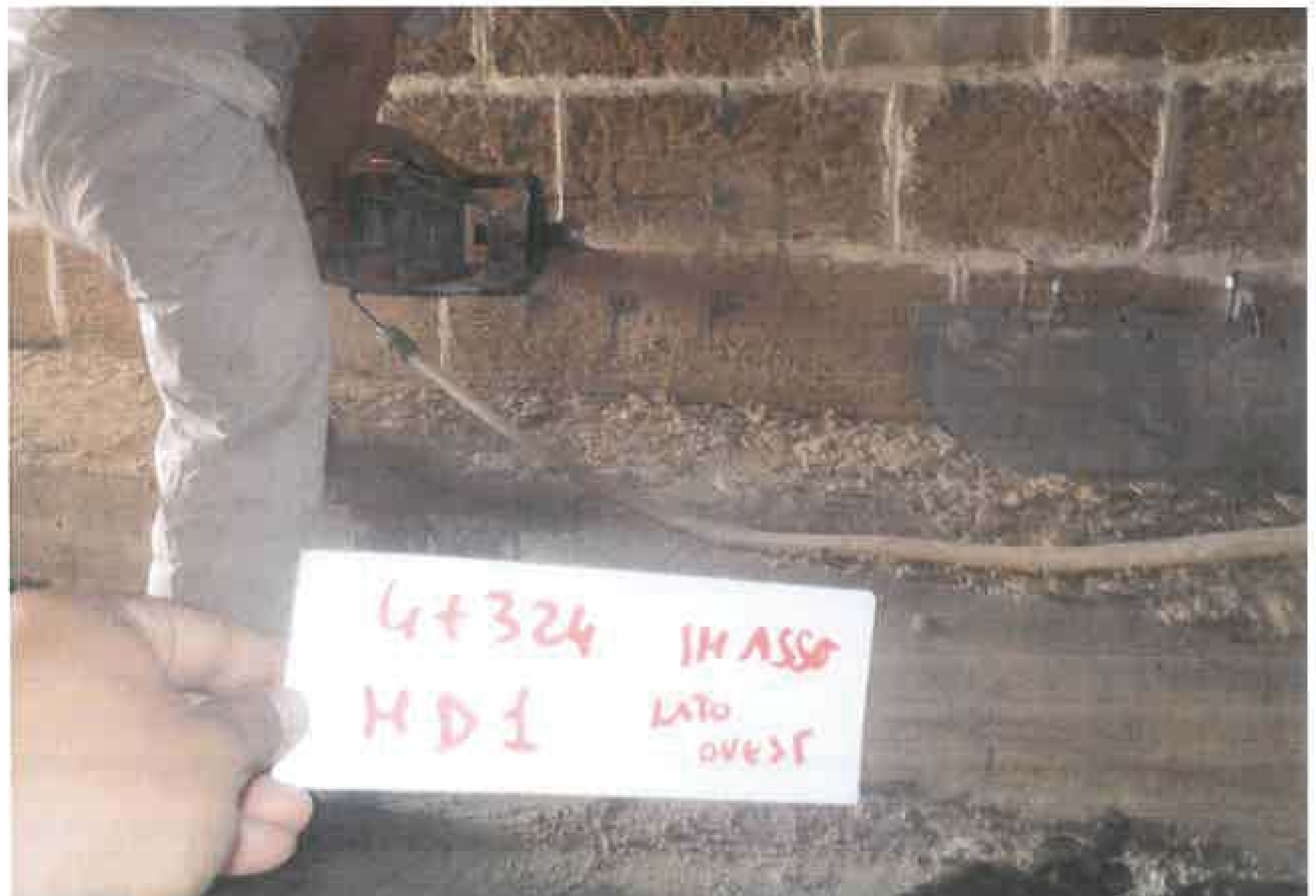
Foto 16 - Taglio inferiore della muratura MD1
