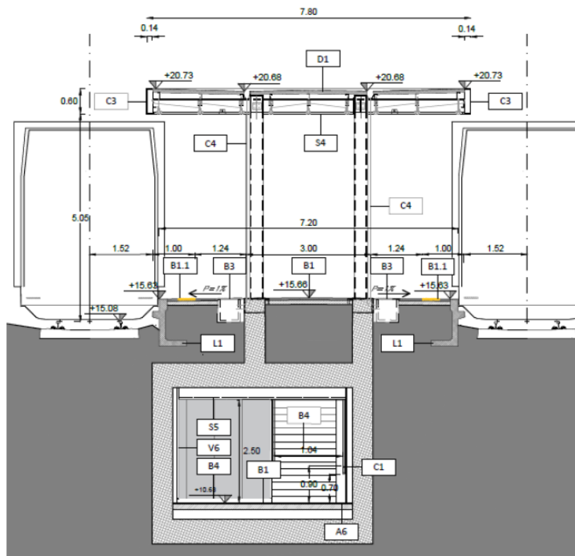
Figura 5-3: sezione pensilina del secondo marciapiede a doppio appoggio
