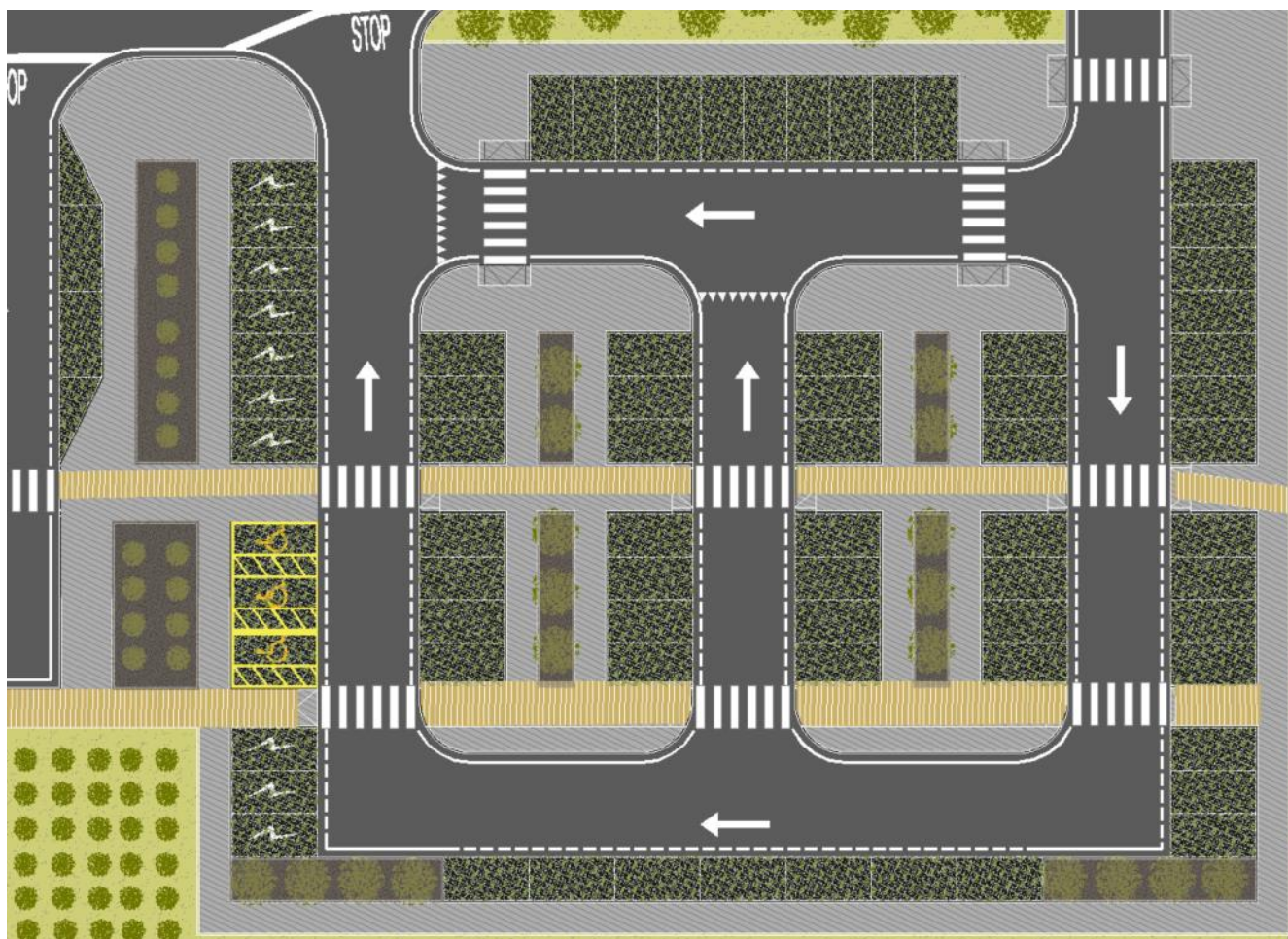
Figura 5-3: Piazzale di stazione con pavimentazione in masselli autobloccanti
