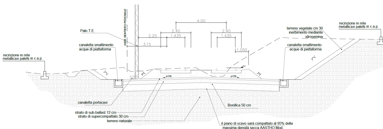
Figura 5-9: Sezione tipo doppio binario in trincea
