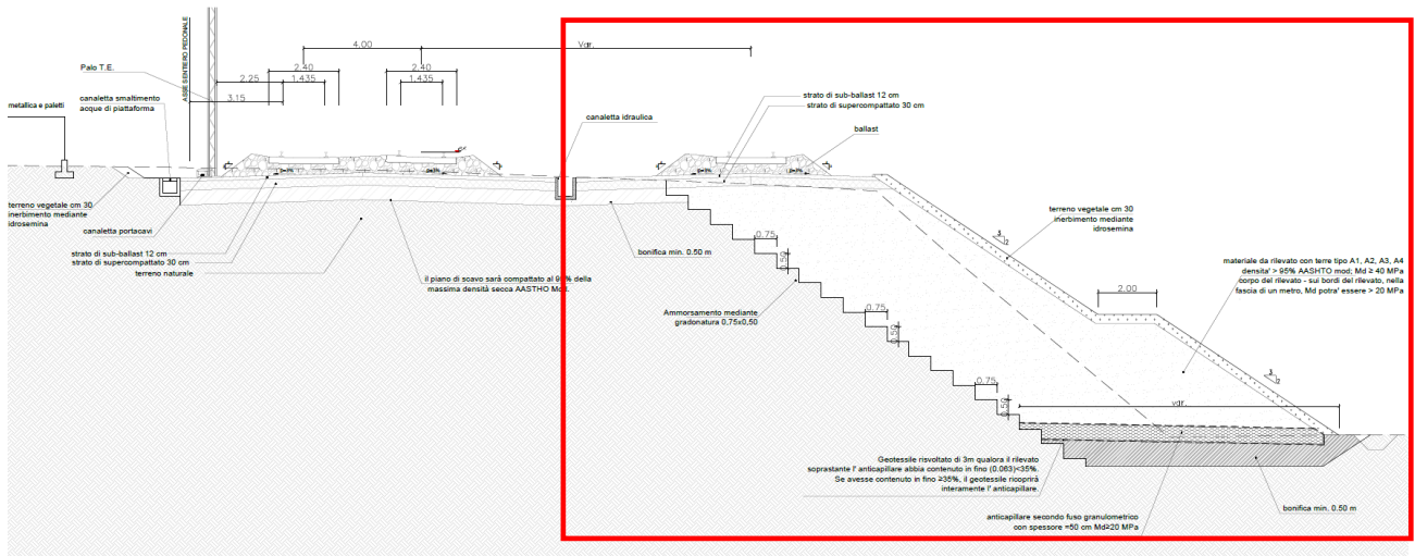
Figura 5-7: Sezione tipo a tre binari in mezzacosta con ammortamento
