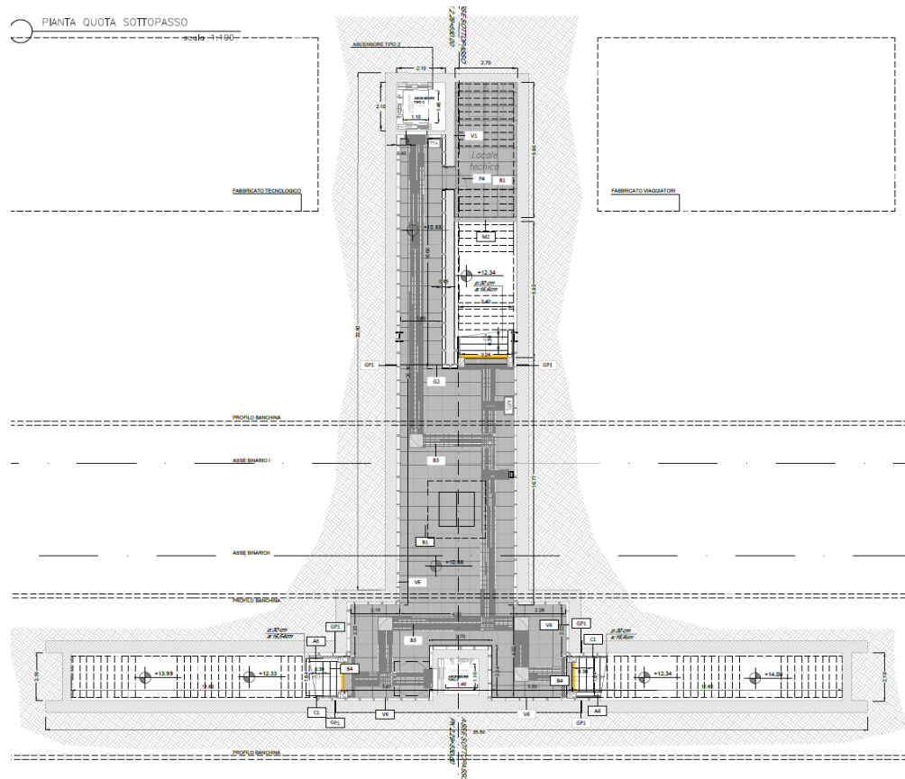
Figura 5-5 Pianta Sottopasso
