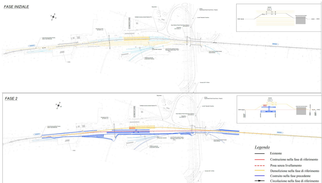
Figura 5-14 Stralcio della tavola Fasi costruttive
