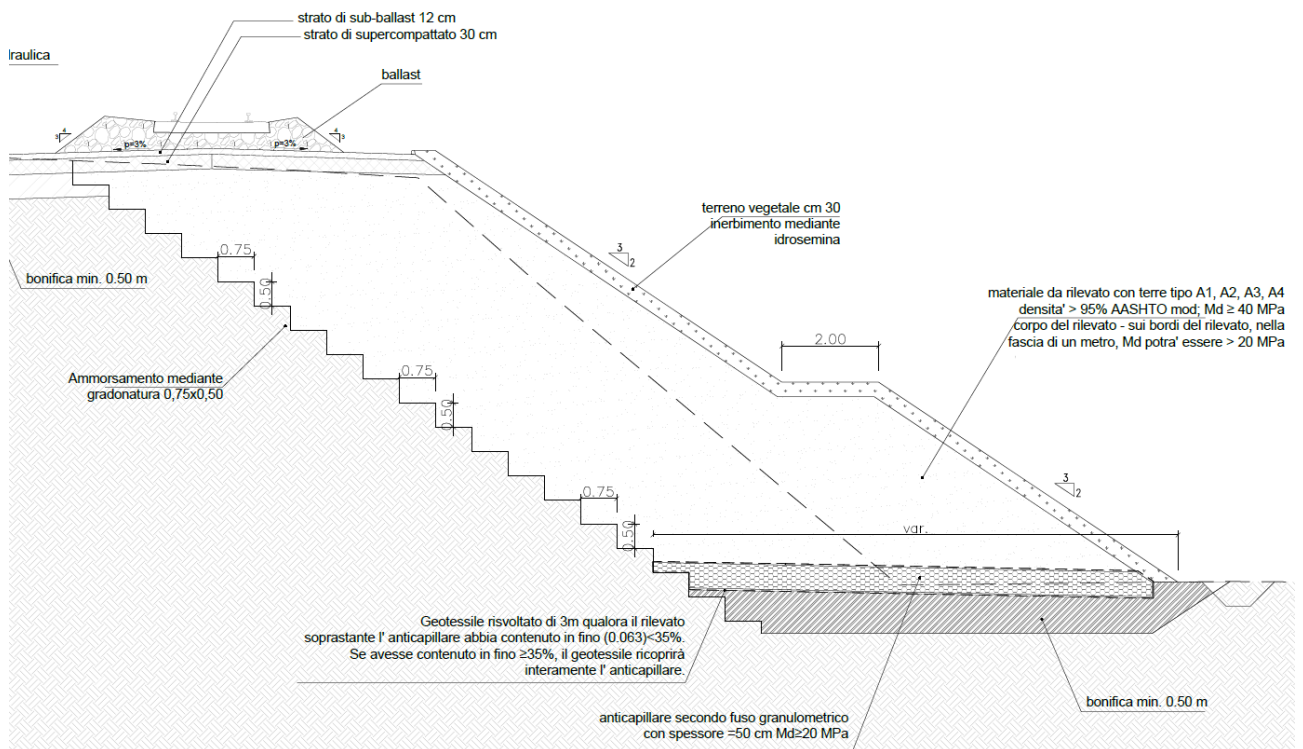
Figura 5-8: Dettaglio della precedente sezione (riquadro rosso)
