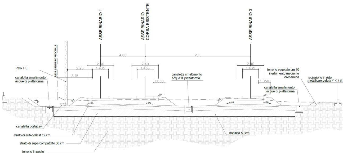
Figura 5-10: Sezione tipo tre binari in trincea
