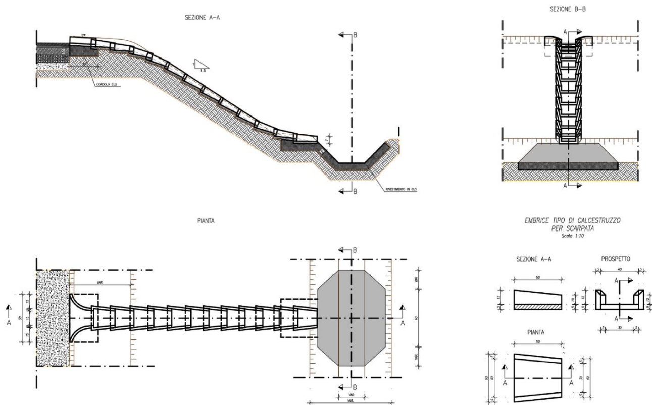
Figura 5-11: Dettaglio degli embrici in pianta e in sezione
