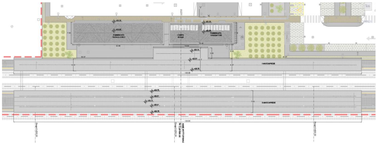
Figura 5-2 Pianta copertura pensiline
