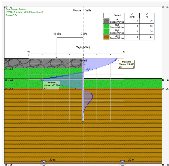
Figura 7: forza di taglio allo SLU-STR
