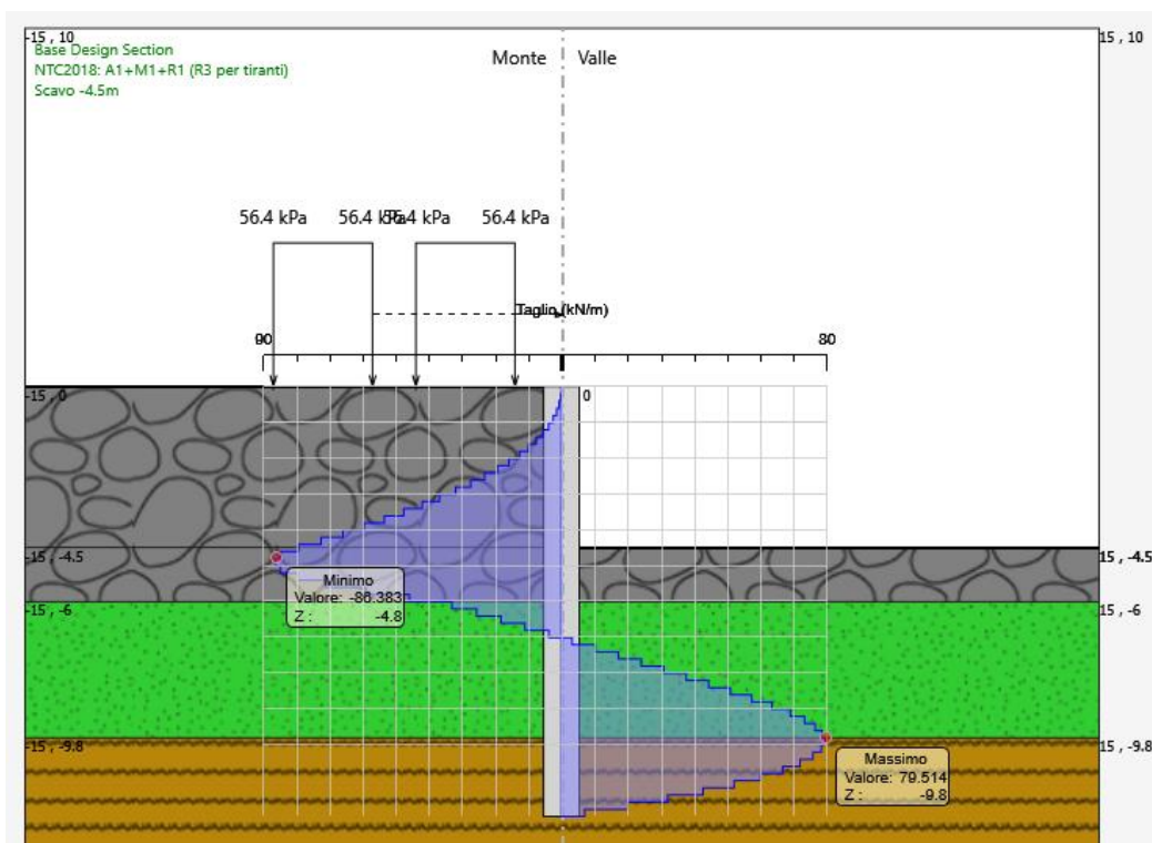
Figura 4: forza di taglio allo SLU-STR
