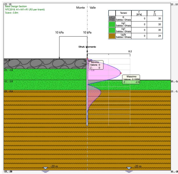
Figura 8: tasso di sfruttamento a flessione
