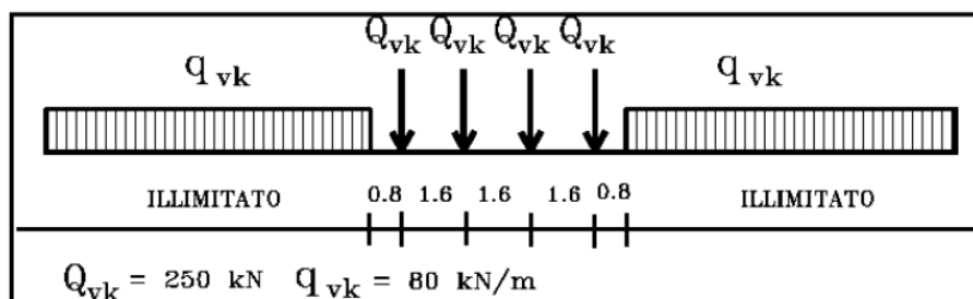
Figura 1 – Modello di carico LM71
