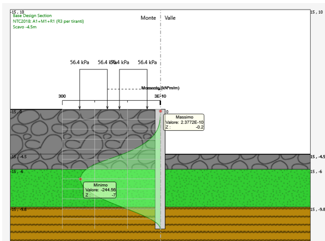
Figura 3: momento flettente allo SLU-STR
