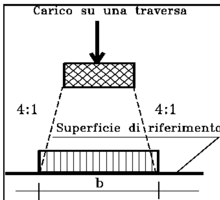
Figura 2 – Distribuzione longitudinale dei carichi attraverso il ballast
