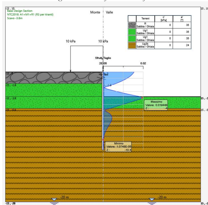
Figura 9: tasso di sfruttamento a taglio
