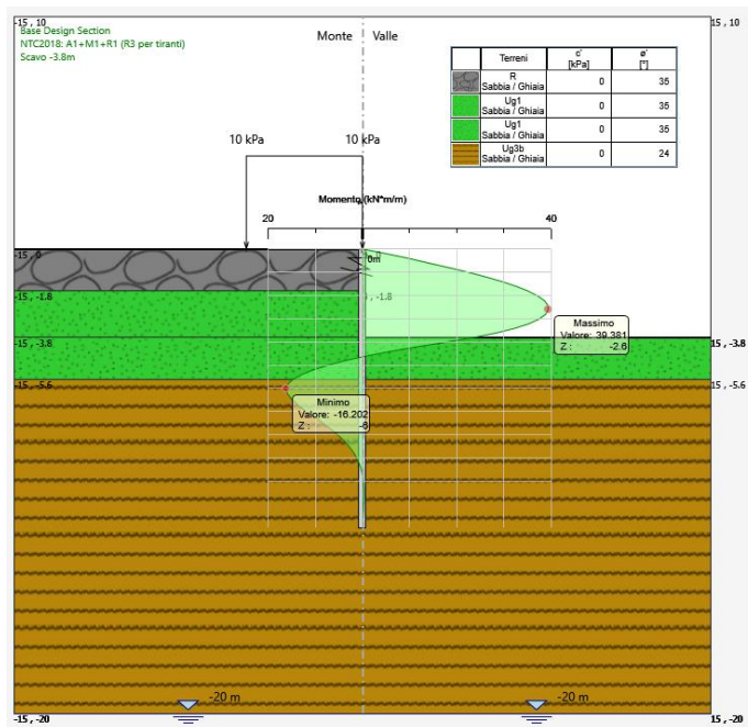
Figura 6: momento flettente allo SLU-STR
