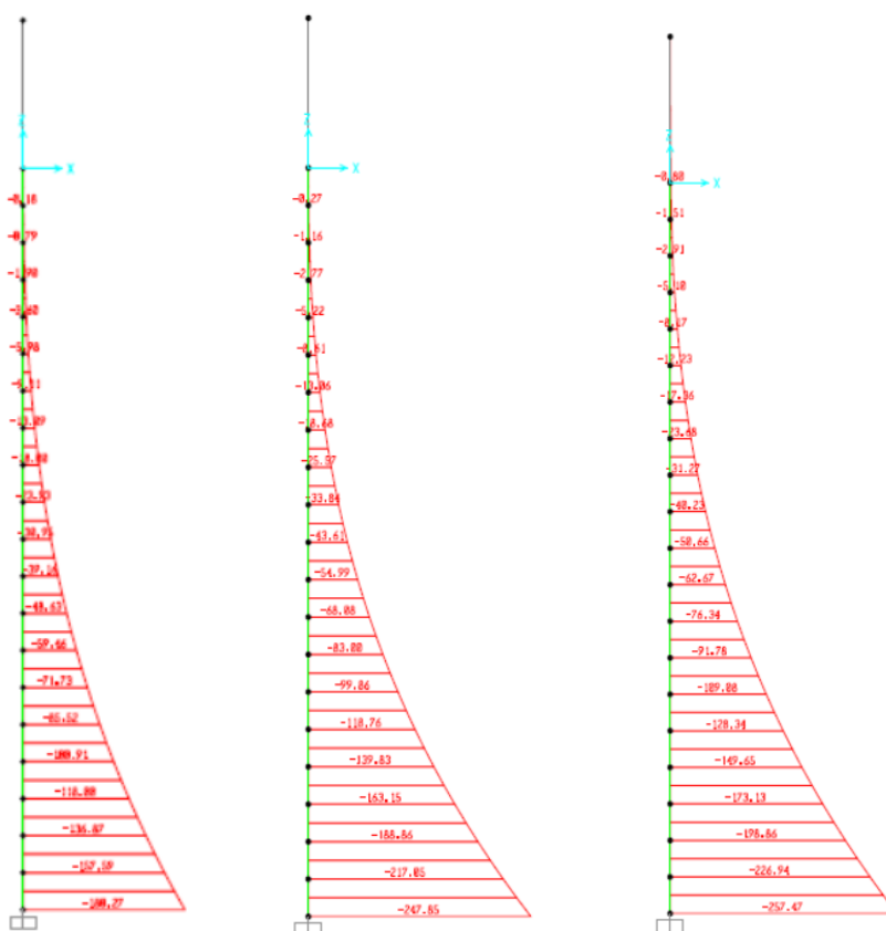
Figura 8: sezione tipo muro in testa alla paratia B – momenti flettenti per le combinazioni SLE, SLU-STR e SLV (da sx verso dx)
