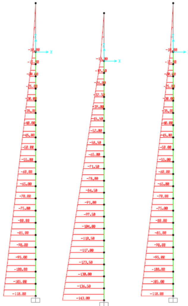
Figura 8: sezione tipo muro in testa alla paratia B – forze assiali per le combinazioni SLE, SLU-STR e SLV (da sx verso dx)
