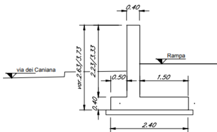
Figura 8: muro di sostegno su via dei Caniana – sezione tipo 1 muro a mensola
