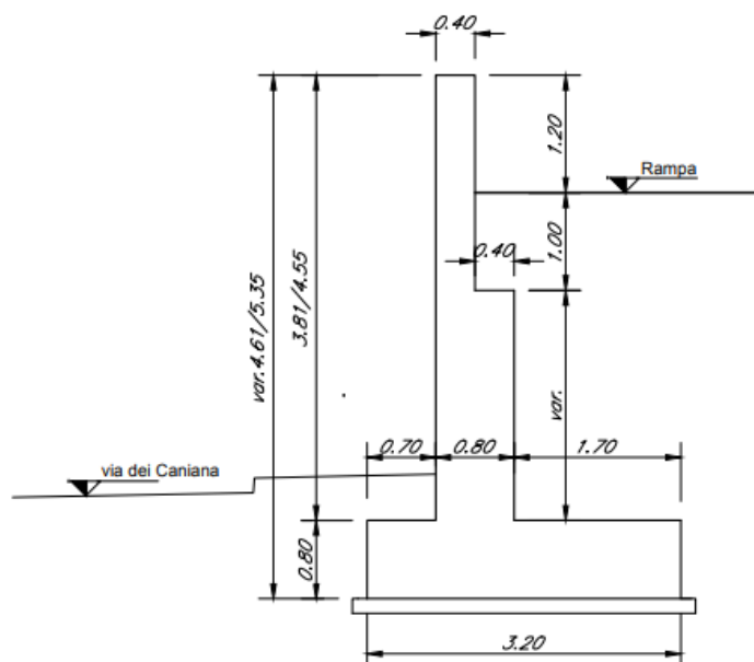
Figura 9: muro di sostegno su via dei Caniana – sezione tipo 2 muro a mensola
