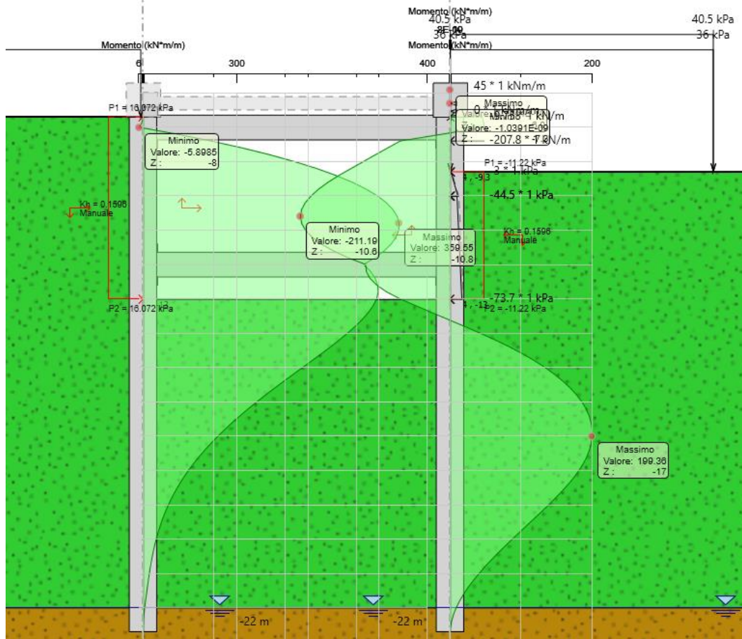
Figura 6: momento flettente allo SISMICA-STR
