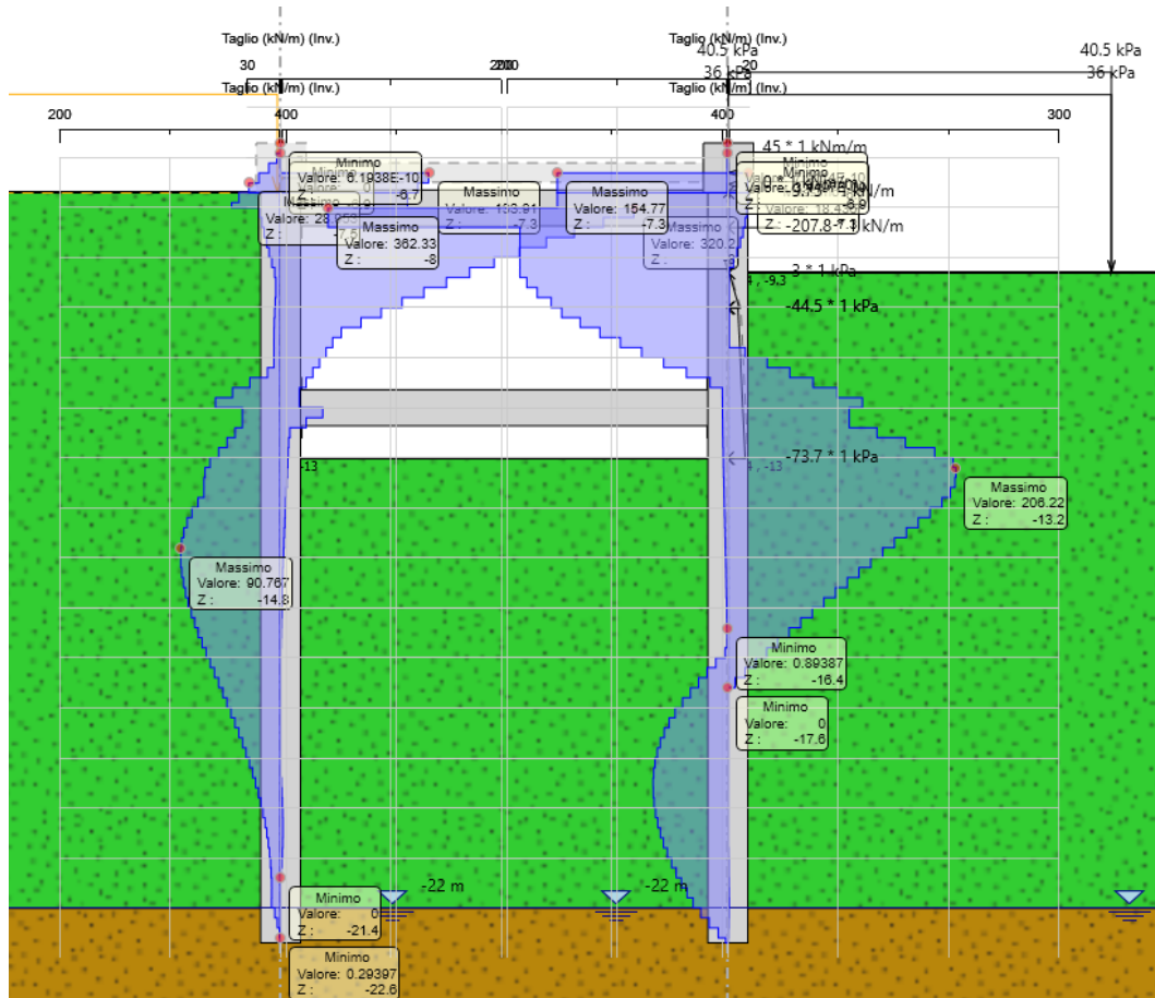
Figura 5: forza di taglio allo SLU-STR
