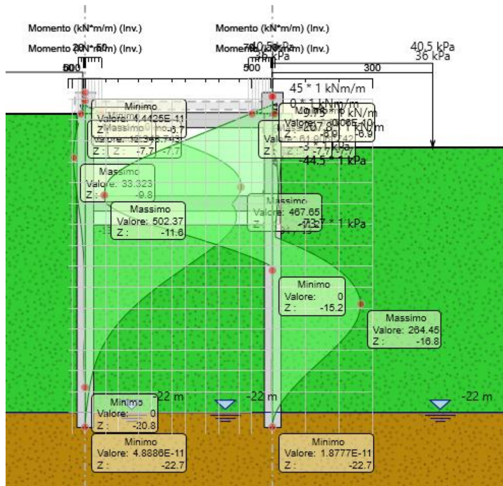
Figura 4: momento flettente allo SLU-STR
