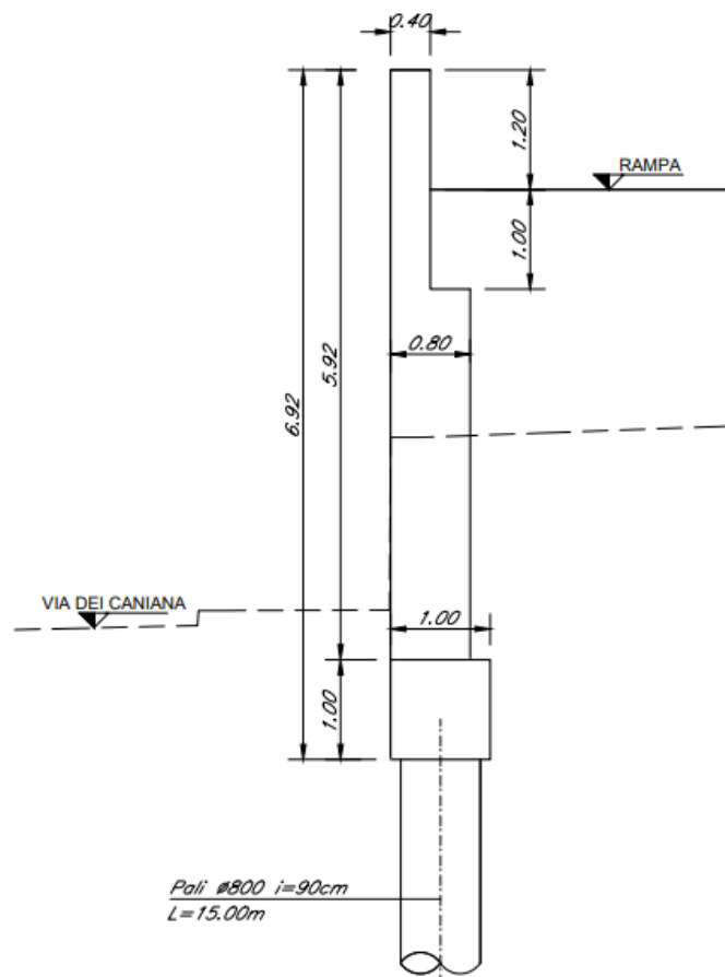
Figura 10: muro di sostegno su va dei Caniana – sezione tipo muro in testa alla paratia B
