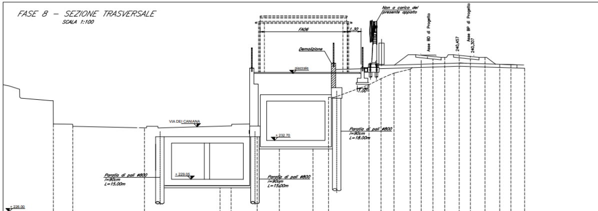
Figura 2 – Vasca di laminazione acque via dei Caniana pianta – Fase lungo termine - sezione
