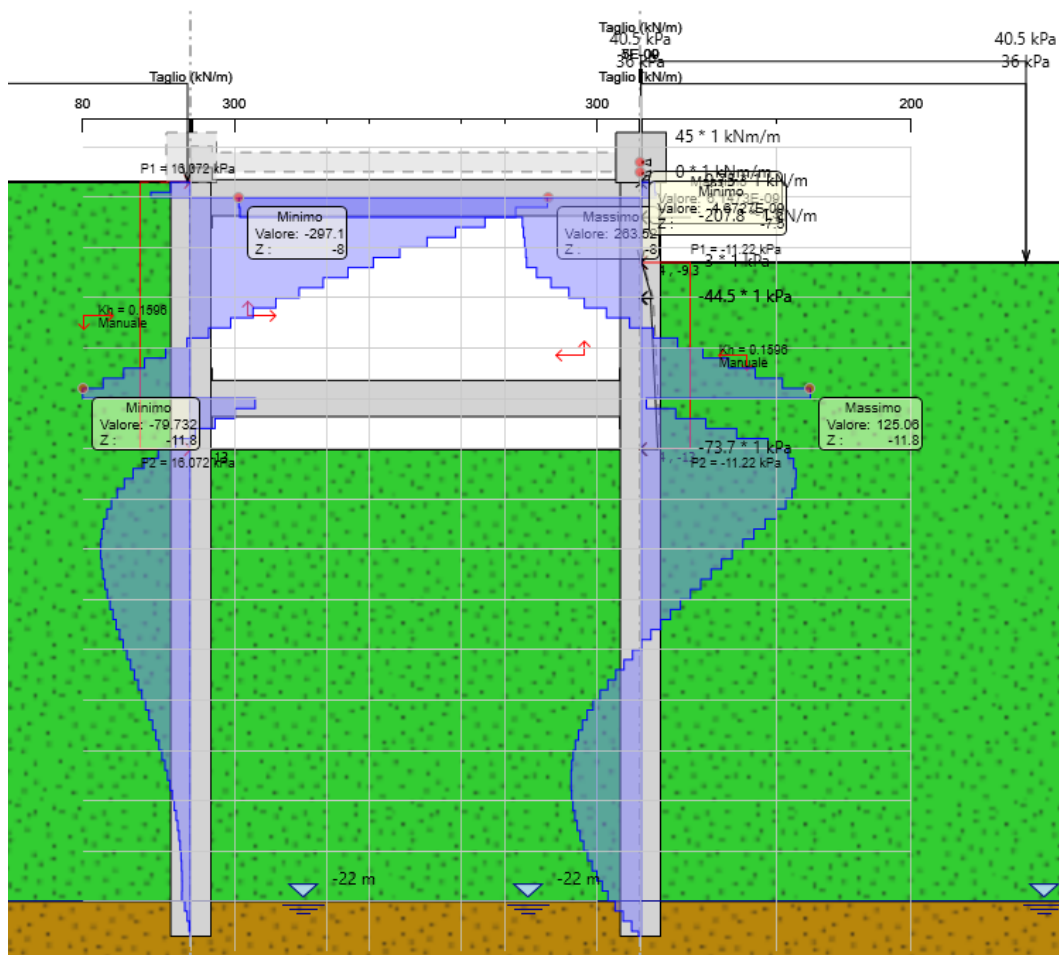
Figura 7: forza di taglio allo SSIMICA-STR
