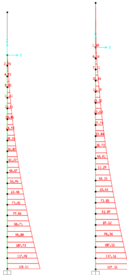
Figura 8: sezione tipo muro in testa alla paratia B – forze di taglio per le combinazioni SLU-STR e SLV (da sx verso dx)
