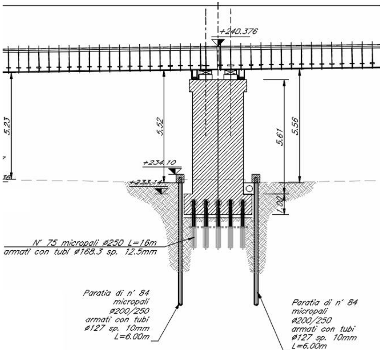
Figura 2 – Pila sezione trasversale
