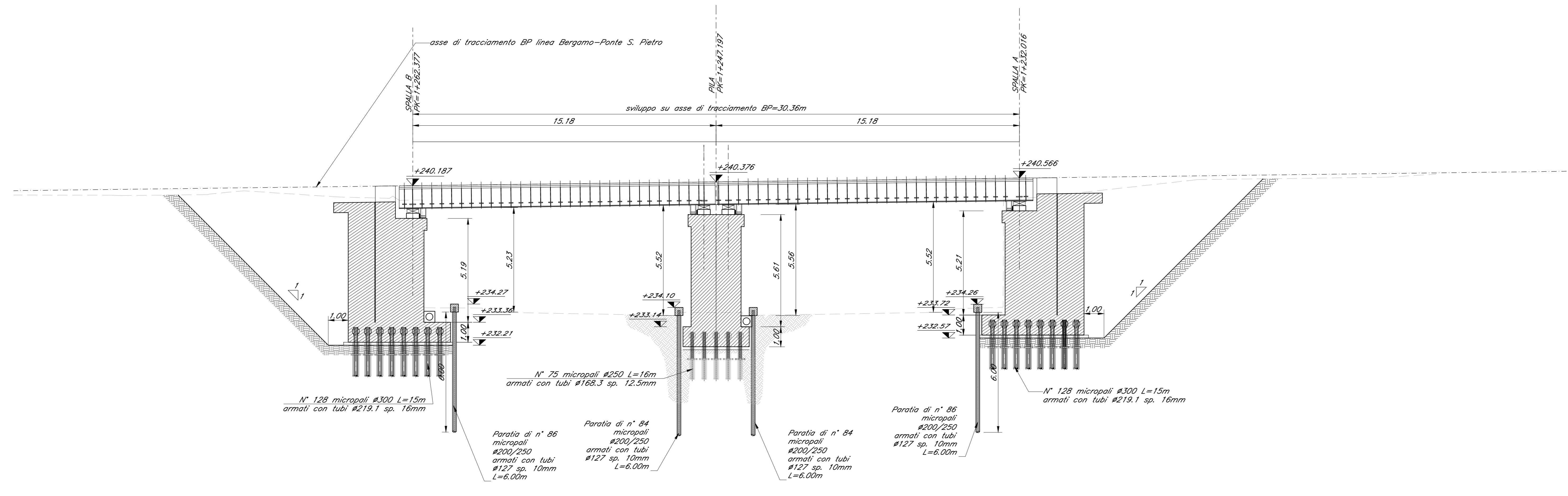
SEZIONE LONGITUDINALE ASSE DI TRACCIAMENTO BP LINEA Bergamo-Ponte S. Pietro Scale 1:100
