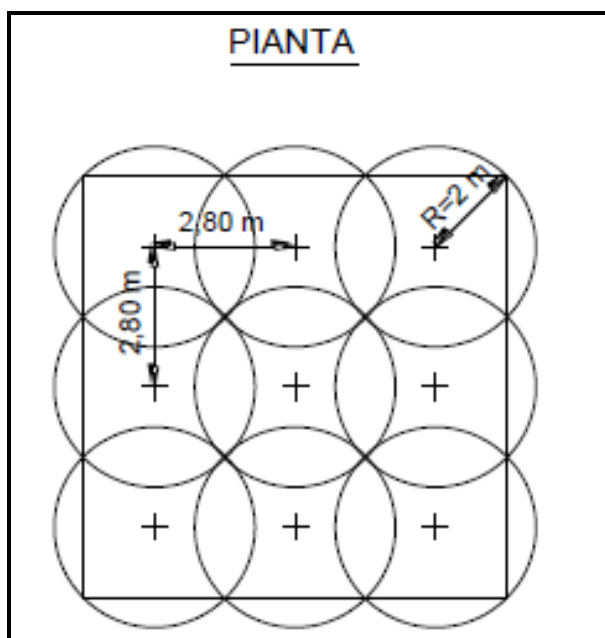
Figura 8-1 – Schema della bonifica profonda – in pianta
