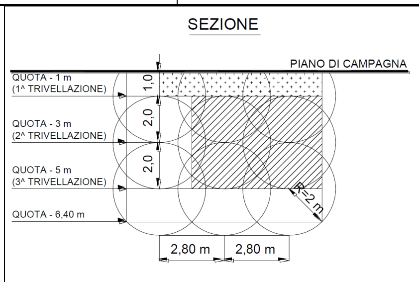
Figura 8-2 – Schema della bonifica profonda – in sezione
