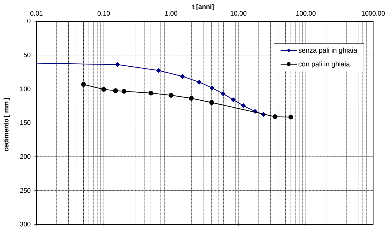
Curva Cedimenti nel tempo
