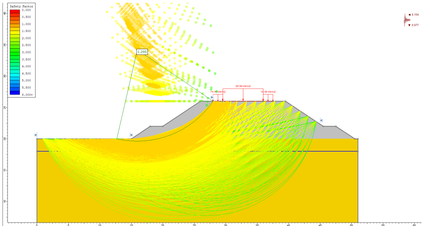
Figura 30 – Analisi di stabilità sismica doppio binario H=6m con banca (kv+)
