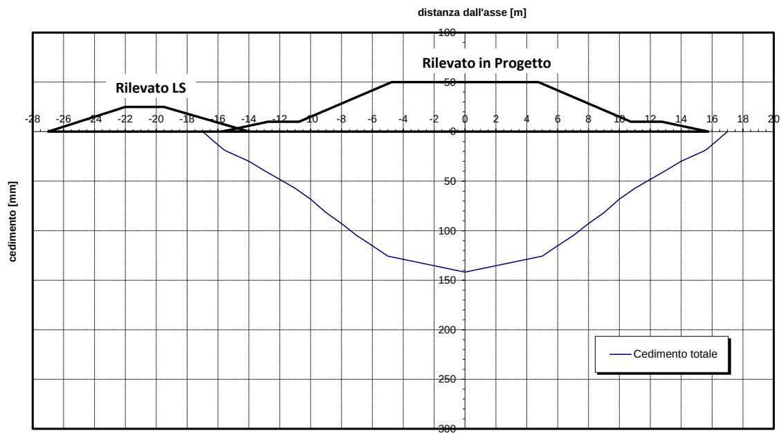
Figura 14 – Cedimento totale RI06 sezione 60 km 2+955
