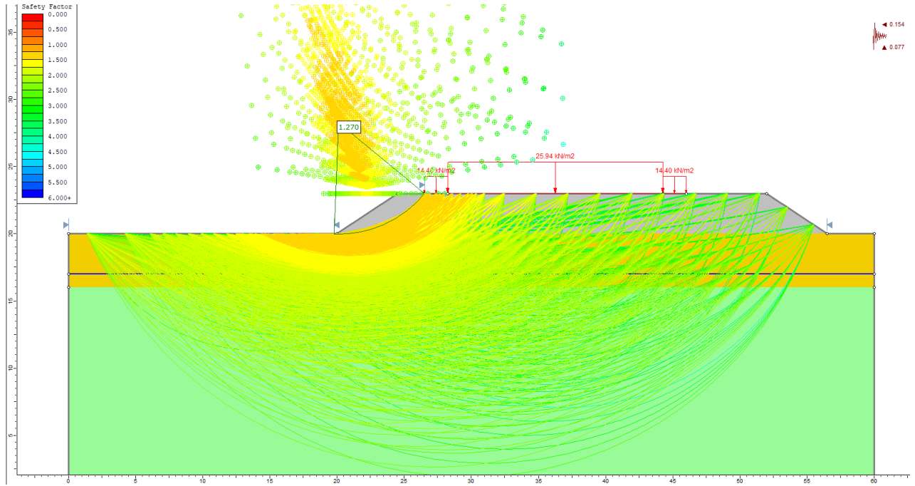
Figura 32 – Analisi di stabilità sismica sezione RI05 km 2+100 H=3m (kv-)
