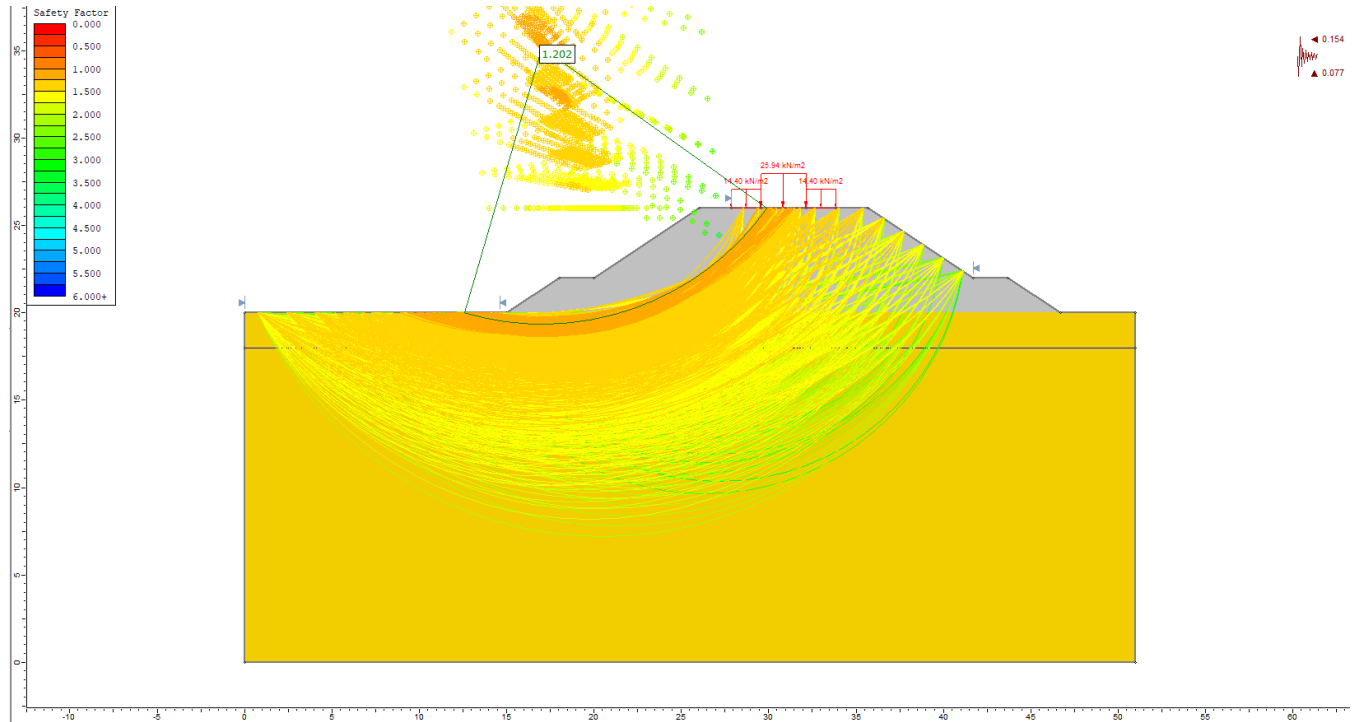
Figura 23 – Analisi di stabilità sismica singolo binario H=6m con banca (kv-)
