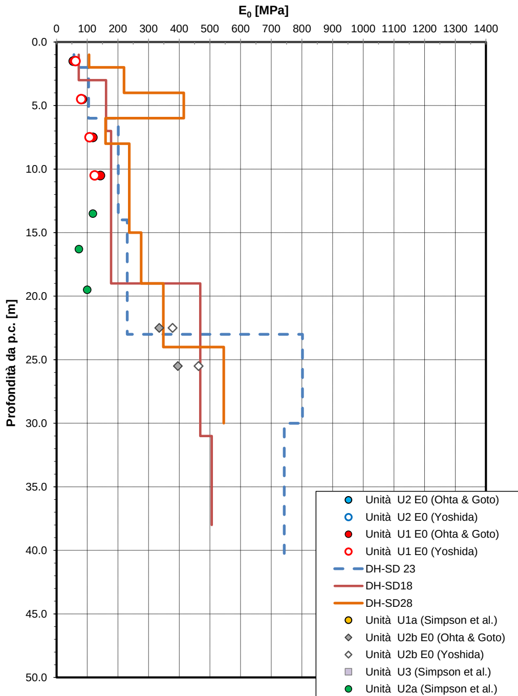
Figura 7 – Modulo di deformazione elastico a piccole deformazioni – RI05 sezione 29
