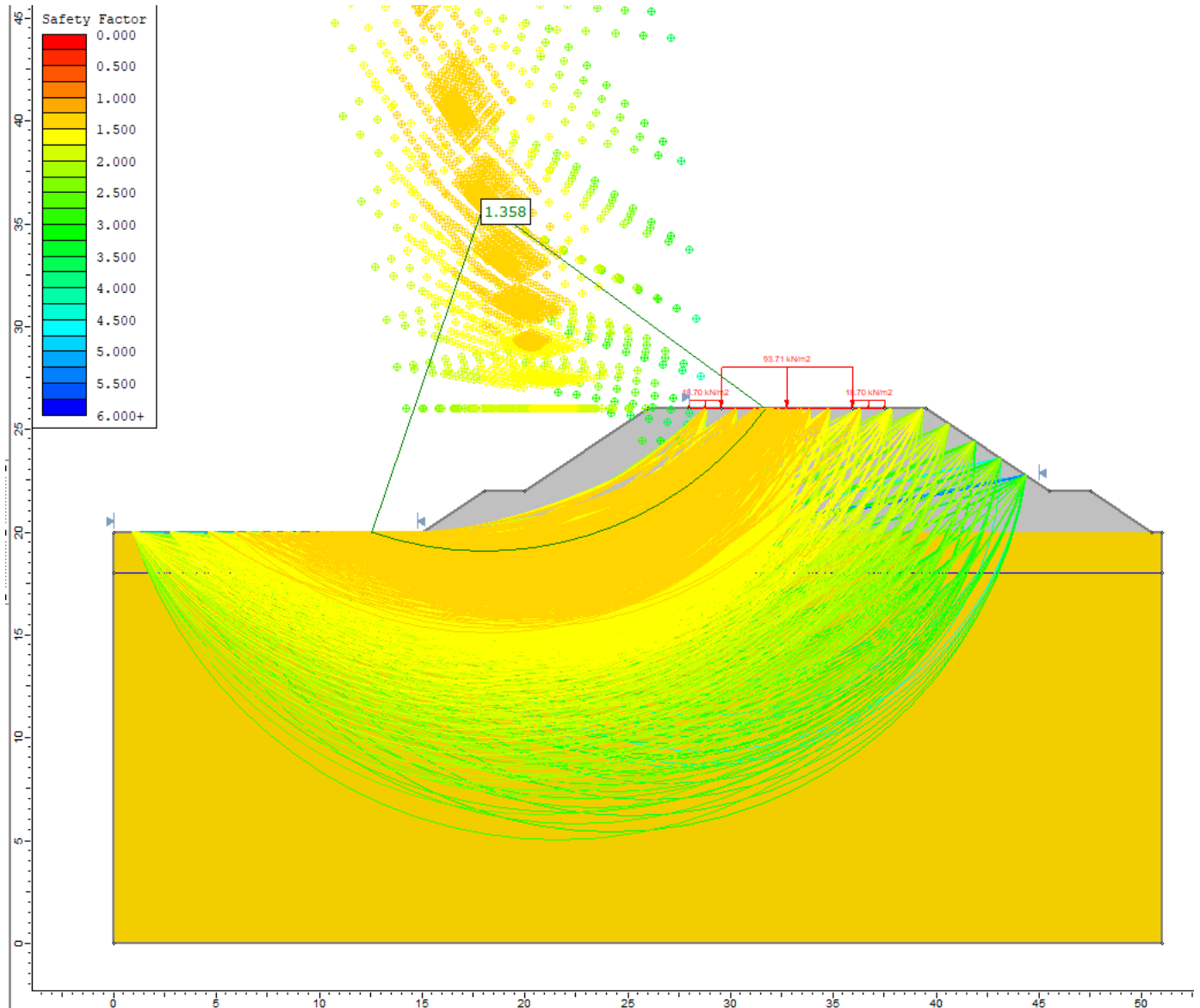
Figura 28 – Analisi di stabilità statica doppio binario H=6\text{m} con banca
