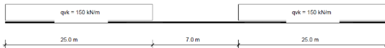
Figura 17 – Treno di carico SW2.
