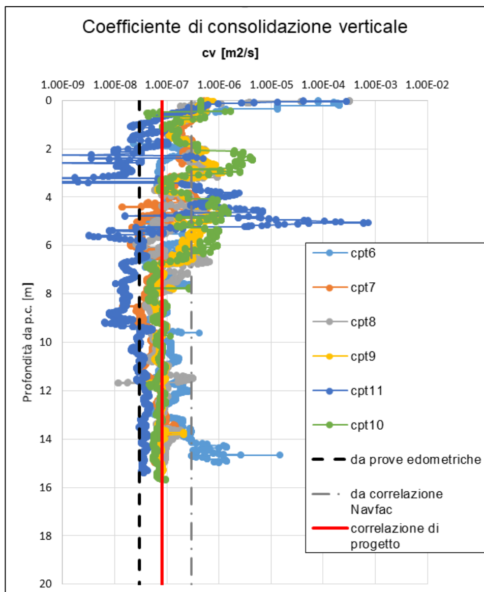
Figura 3 – Coefficiente di consolidazione verticale (da prove CPT, da edometriche di laboratorio e correlazione Navfac)
