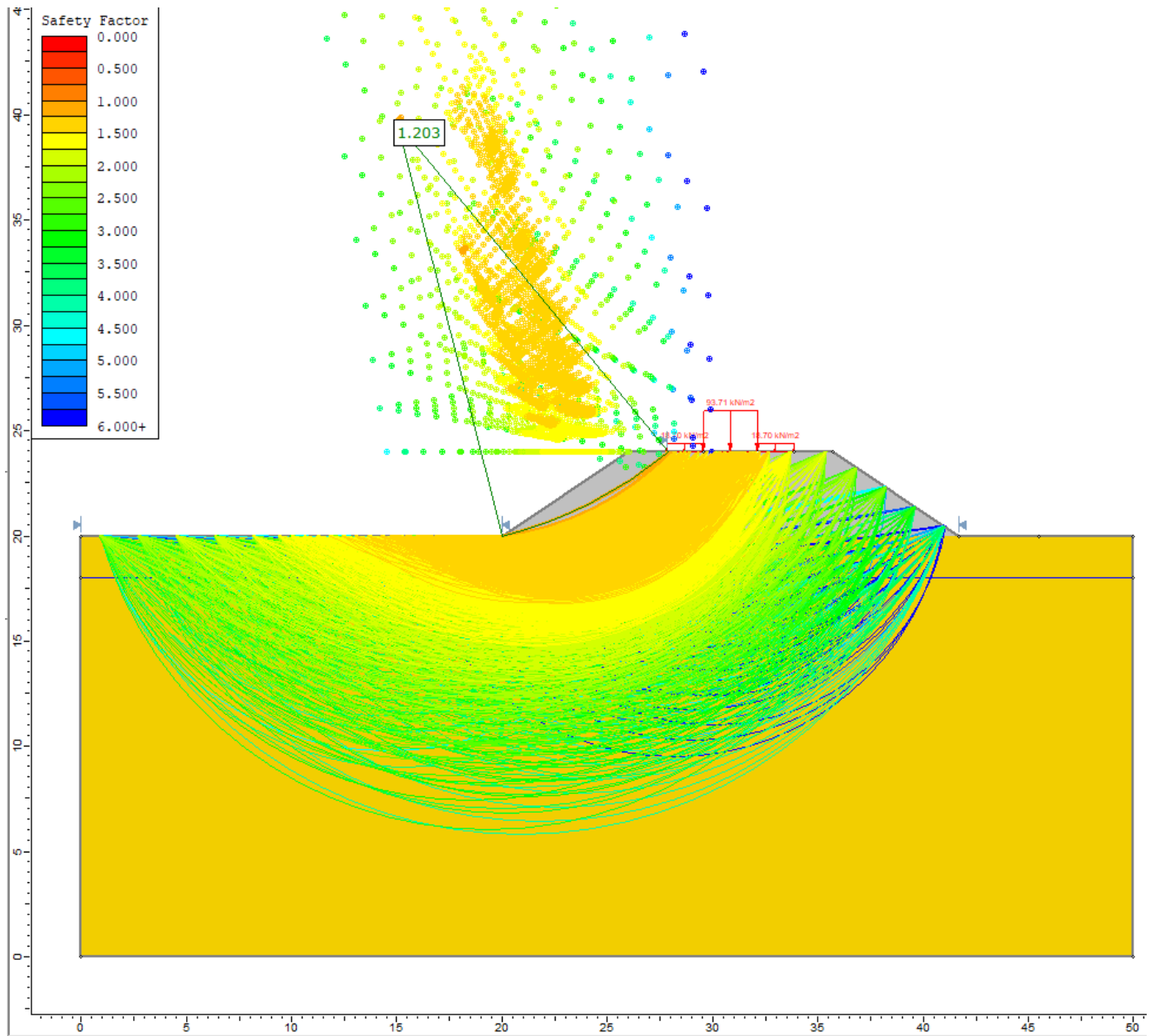
Figura 19 – Analisi di stabilità statica singolo binario H=4m
