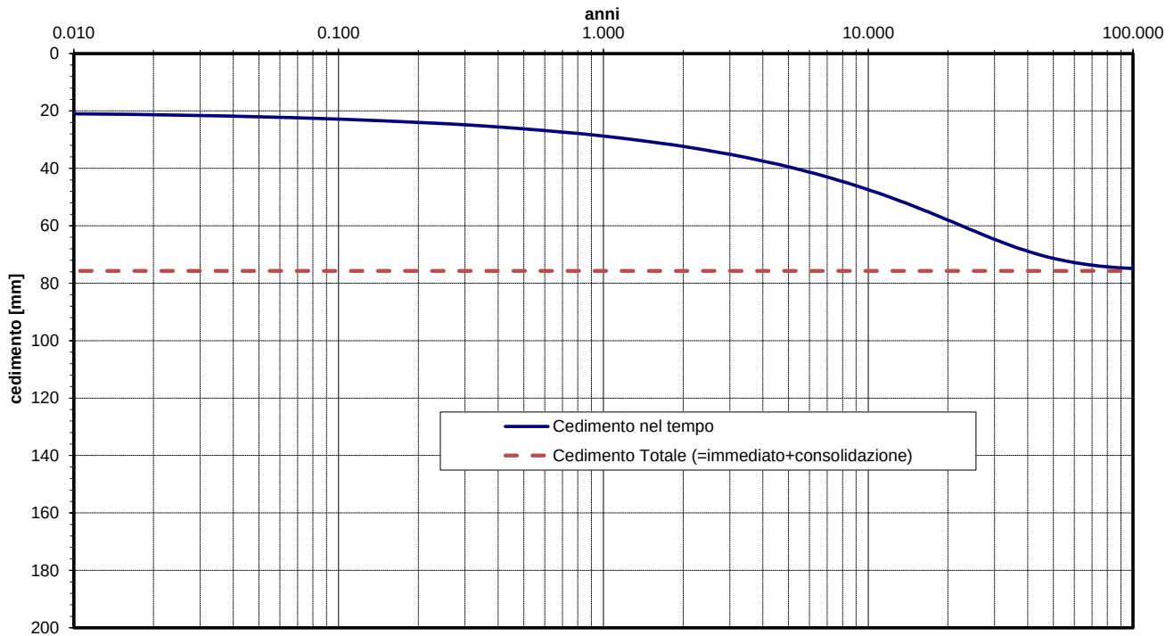
Figura 13 – Decorso dei cedimenti nel tempo – RI05 sez 42 km 2+100– H=3m
