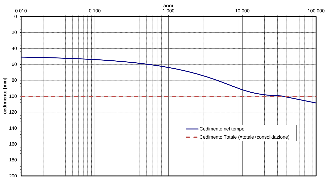
Figura 11 – Decorso dei cedimenti nel tempo – RI04 – H=6m
