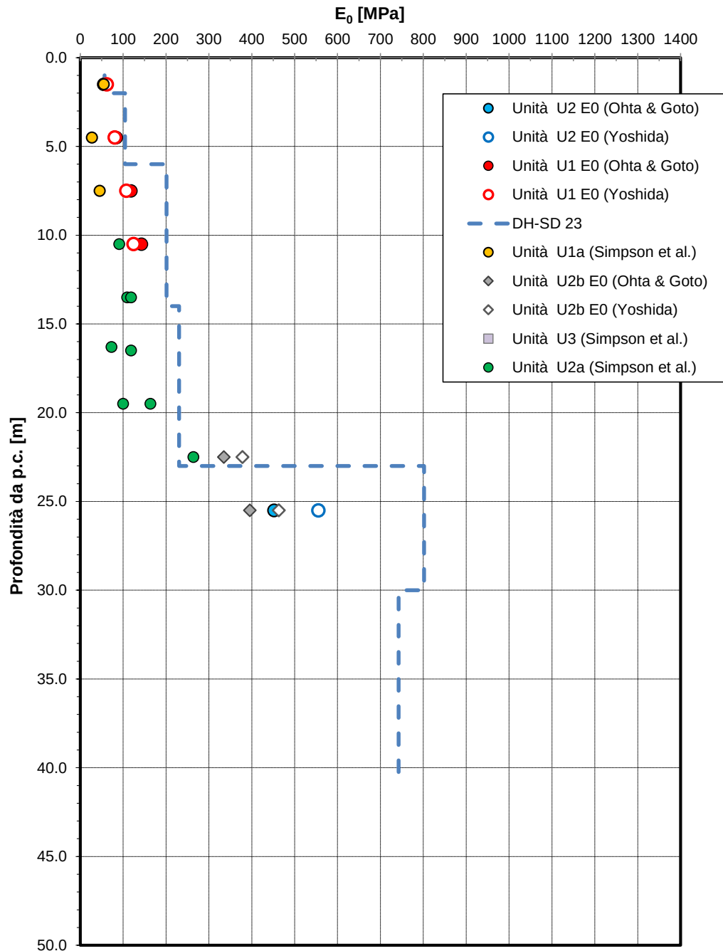
Figura 10 – Modulo di deformazione elastico a piccole deformazioni – RI08 sezione 13
