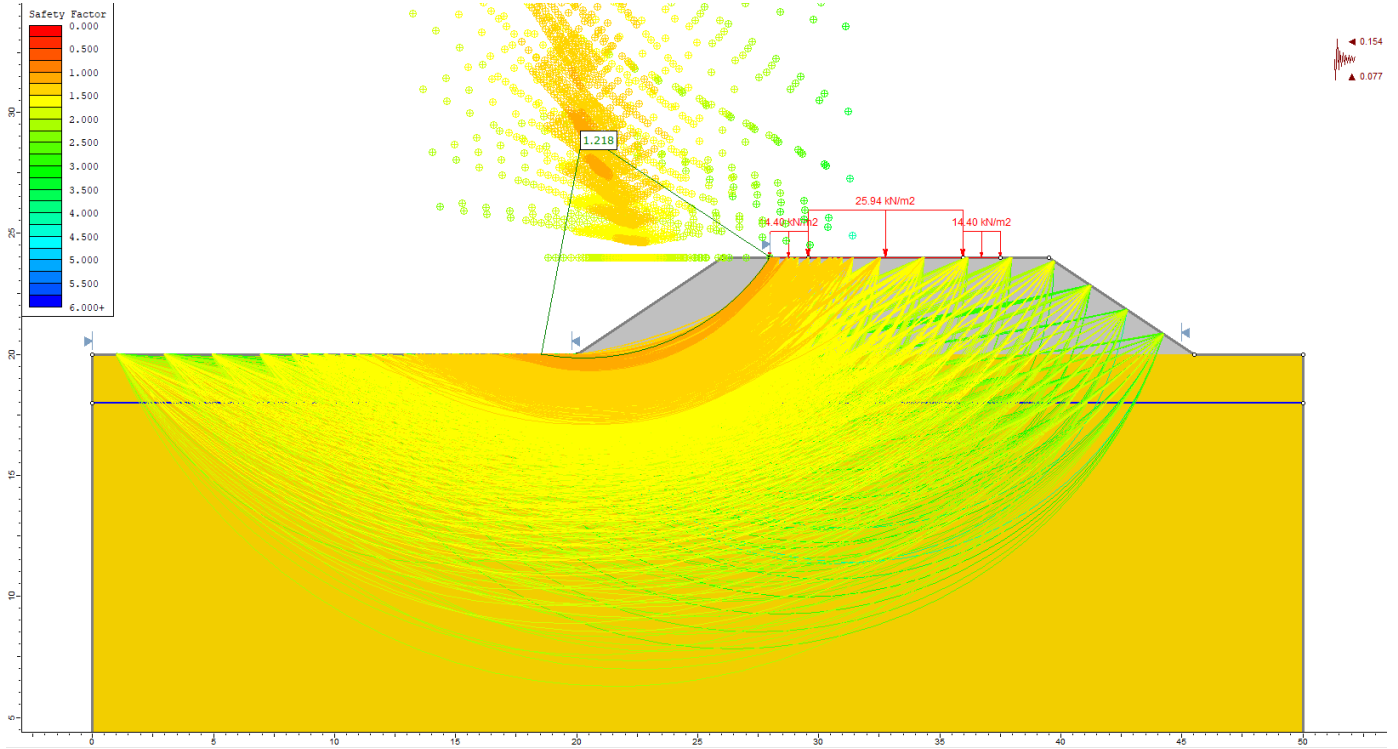
Figura 26 – Analisi di stabilità sismica doppio binario H=4m (kv-)
