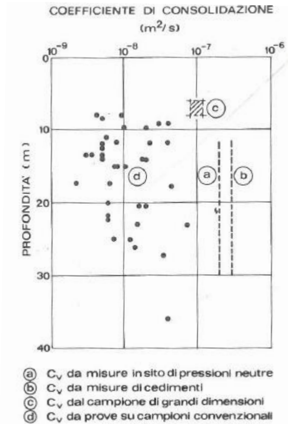
Figura 4 – Confronto fra valori del coefficiente di consolidazione ottenuto da diverse procedure (Bugnignoli e Calabresi, 1975)
