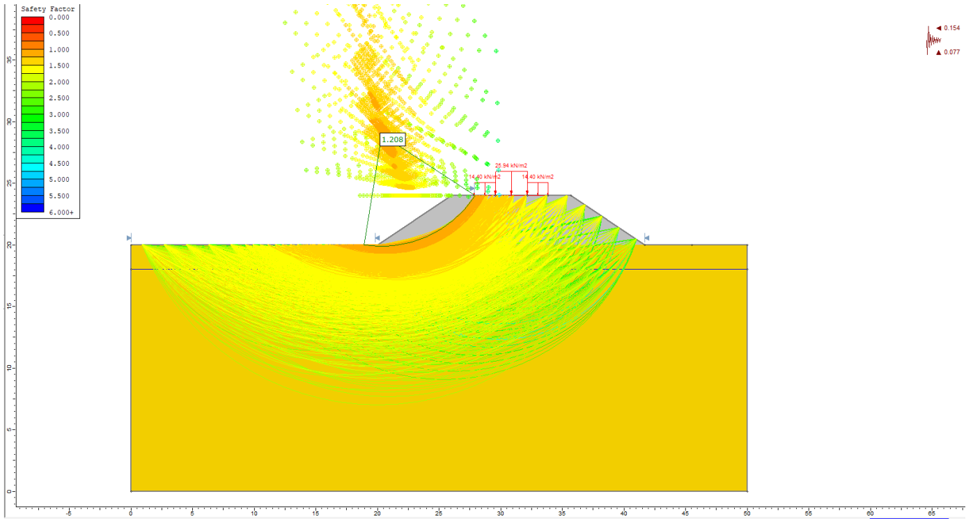
Figura 20 – Analisi di stabilità sismica singolo binario H=4m (kv-)
