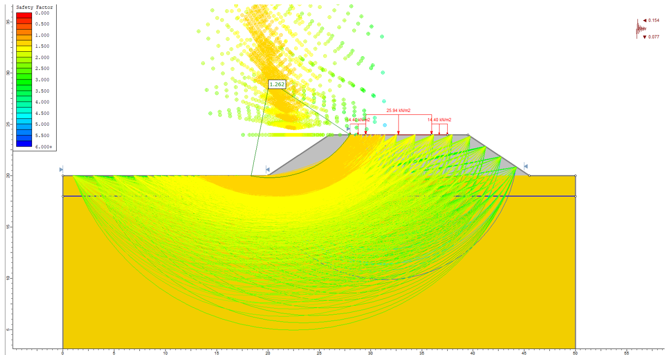
Figura 27 – Analisi di stabilità sismica doppio binario H=4m (kv+)
