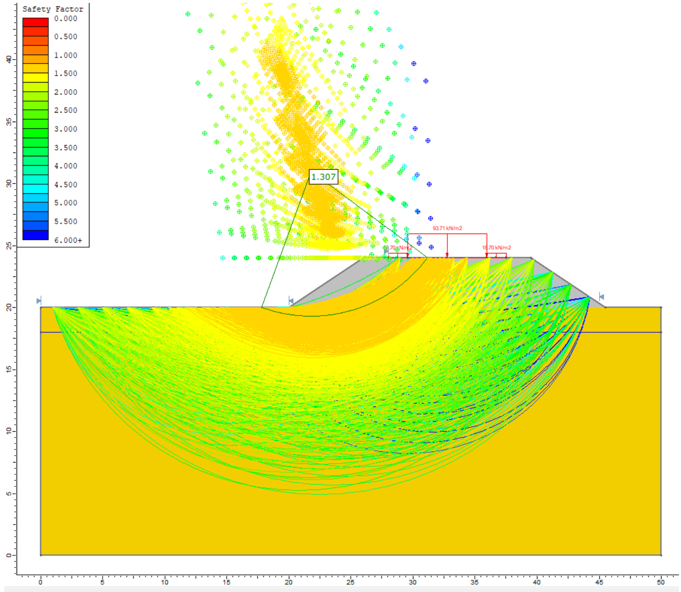
Figura 25 – Analisi di stabilità statica doppio binario H=4\text{m}
