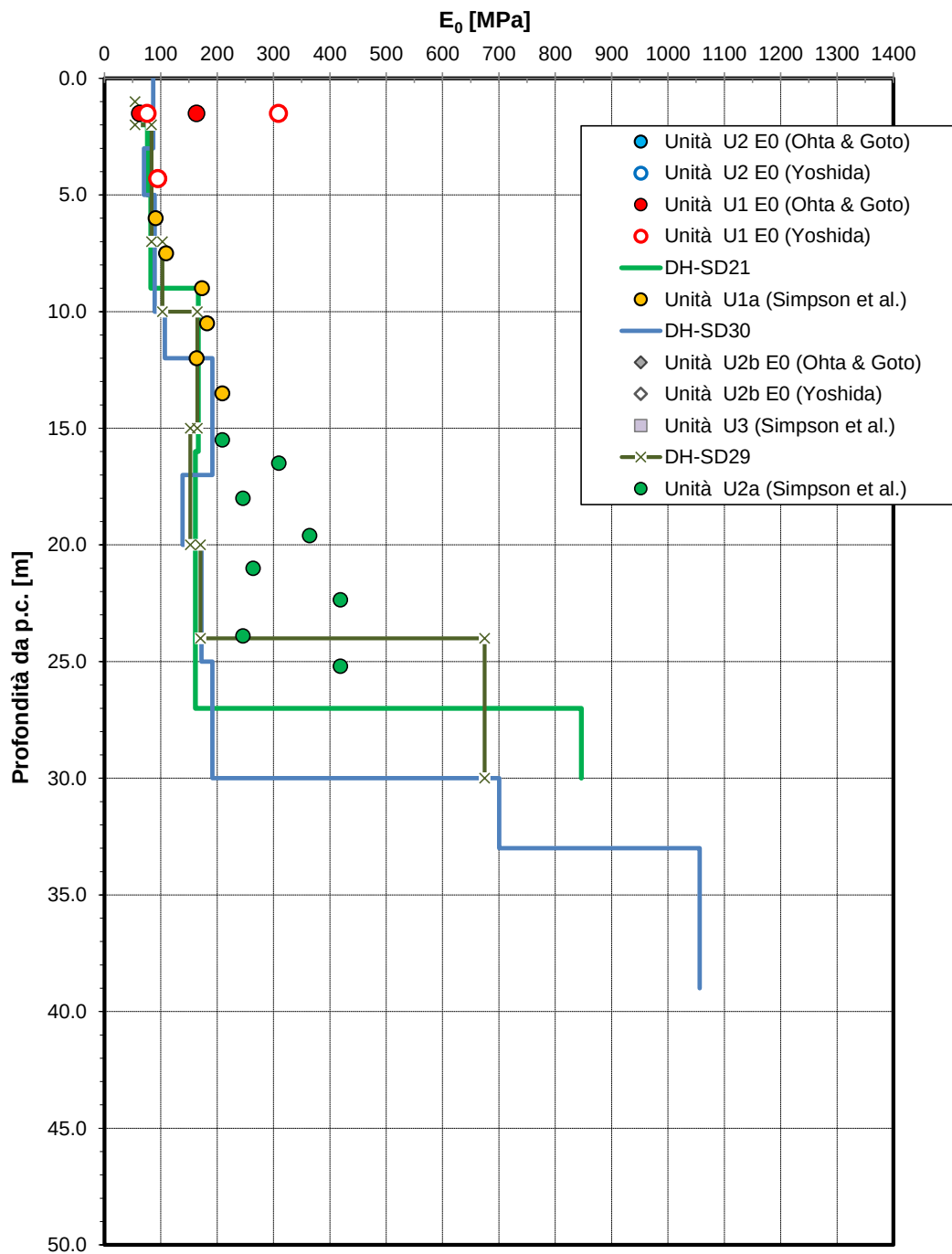
Figura 8 – Modulo di deformazione elastico a piccole deformazioni – RI05 sezione 42
