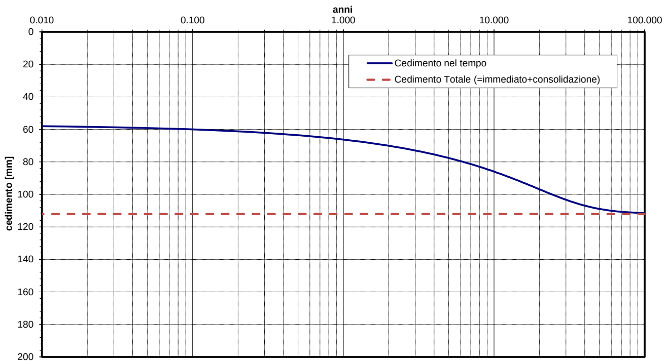
Figura 16 – Decorso dei cedimenti nel tempo – RI08 sez 13 km 0+600 – H=6m
