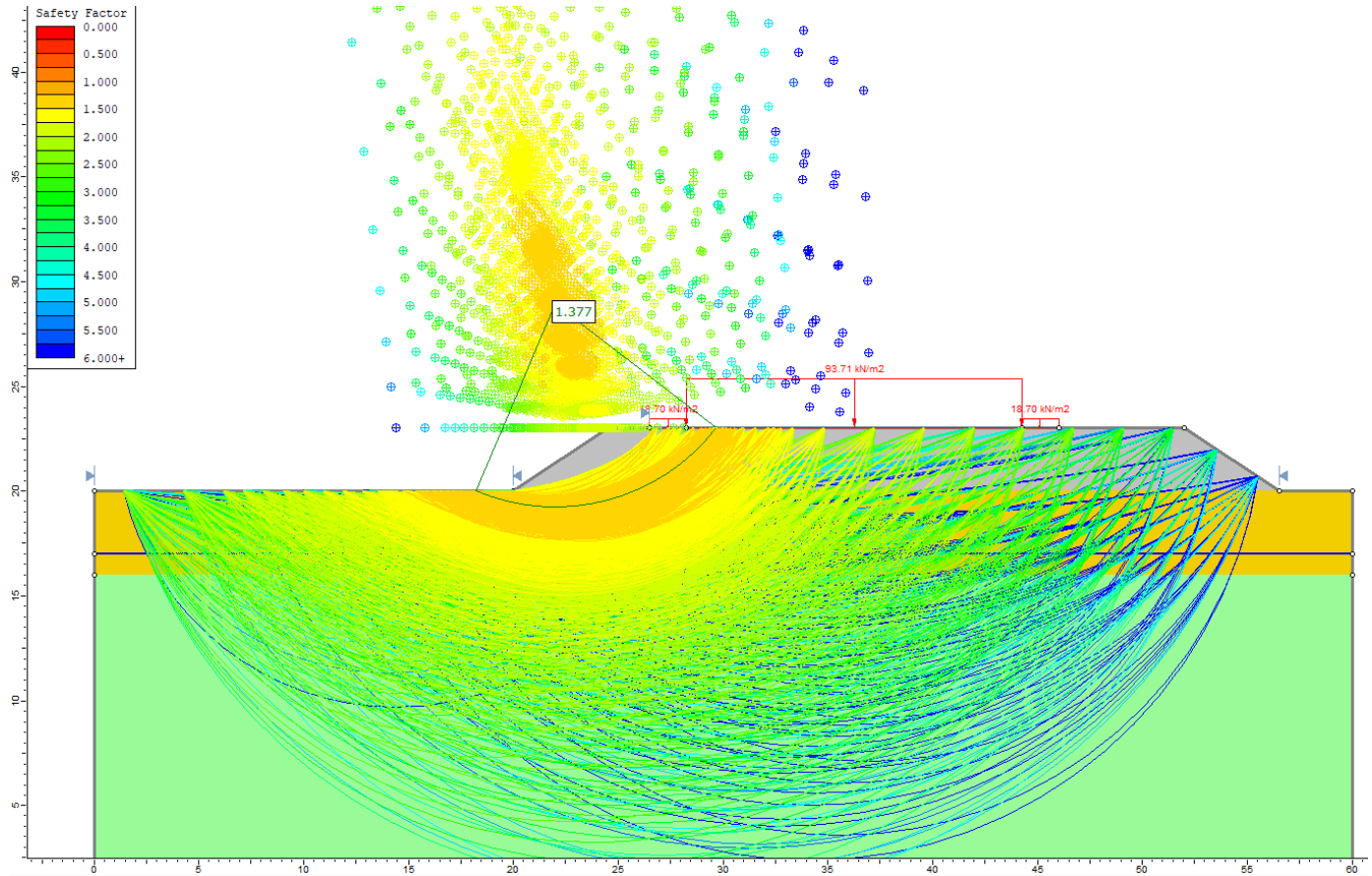
Figura 31 – Analisi di stabilità statica sezione RI05 km 2+100 H=3m
