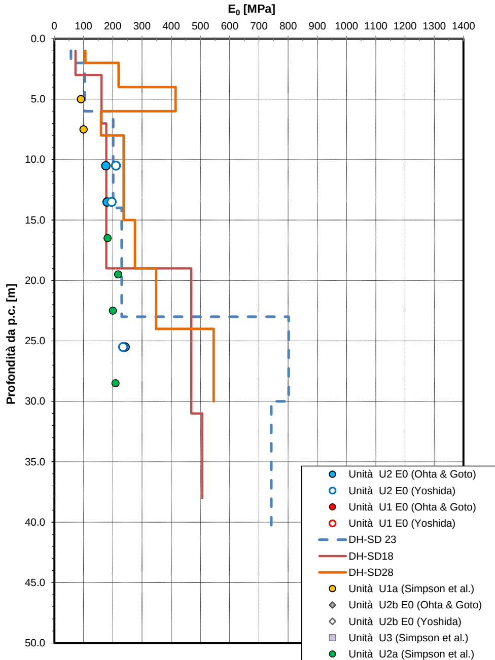
Figura 6 – Modulo di deformazione elastico a piccole deformazioni – RI04/VI01
