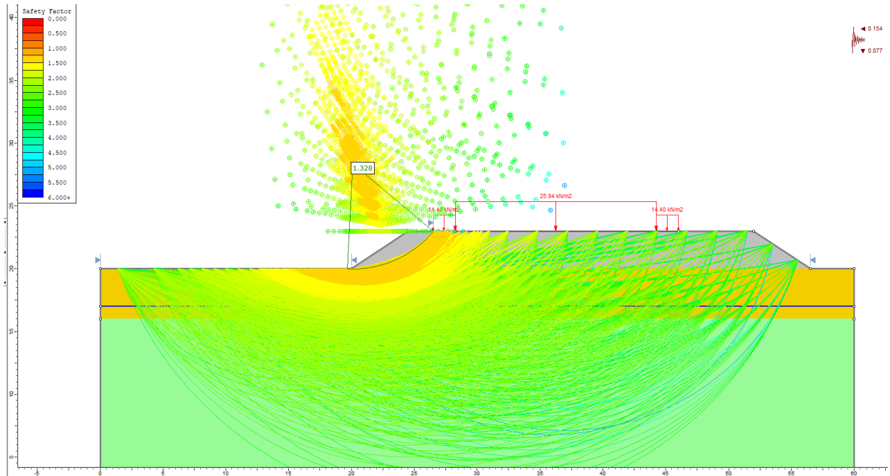
Figura 33 – Analisi di stabilità sismica sezione RI05 km 2+100 H=3m (kv+)
