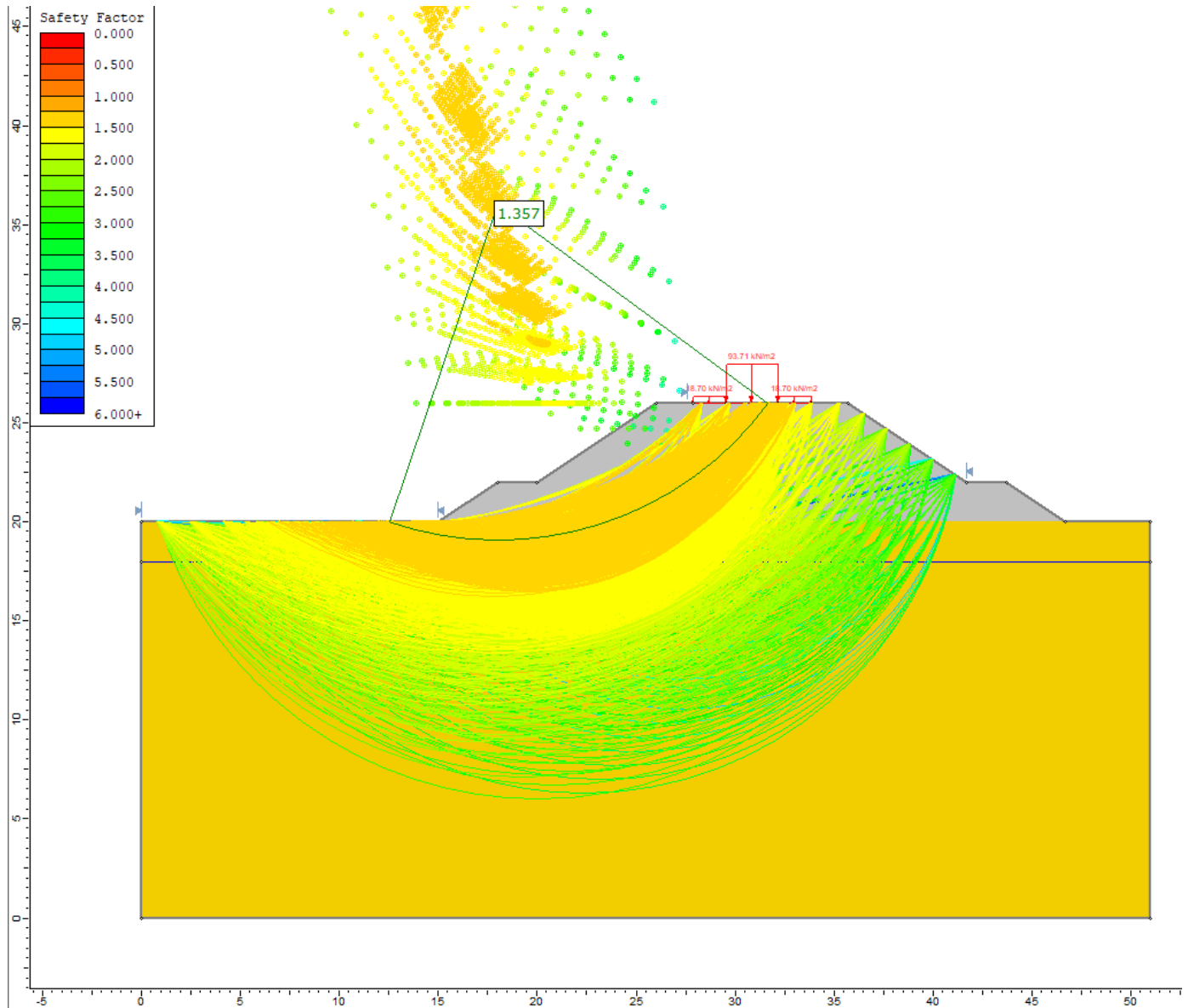
Figura 22 – Analisi di stabilità statica singolo binario H=6m con banca
