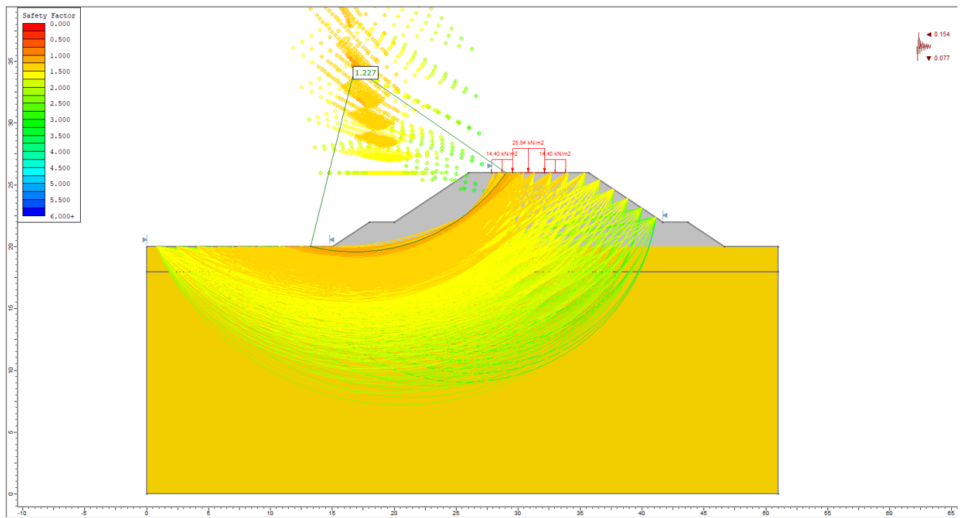
Figura 24 – Analisi di stabilità sismica singolo binario H=6m con banca (kv+)
