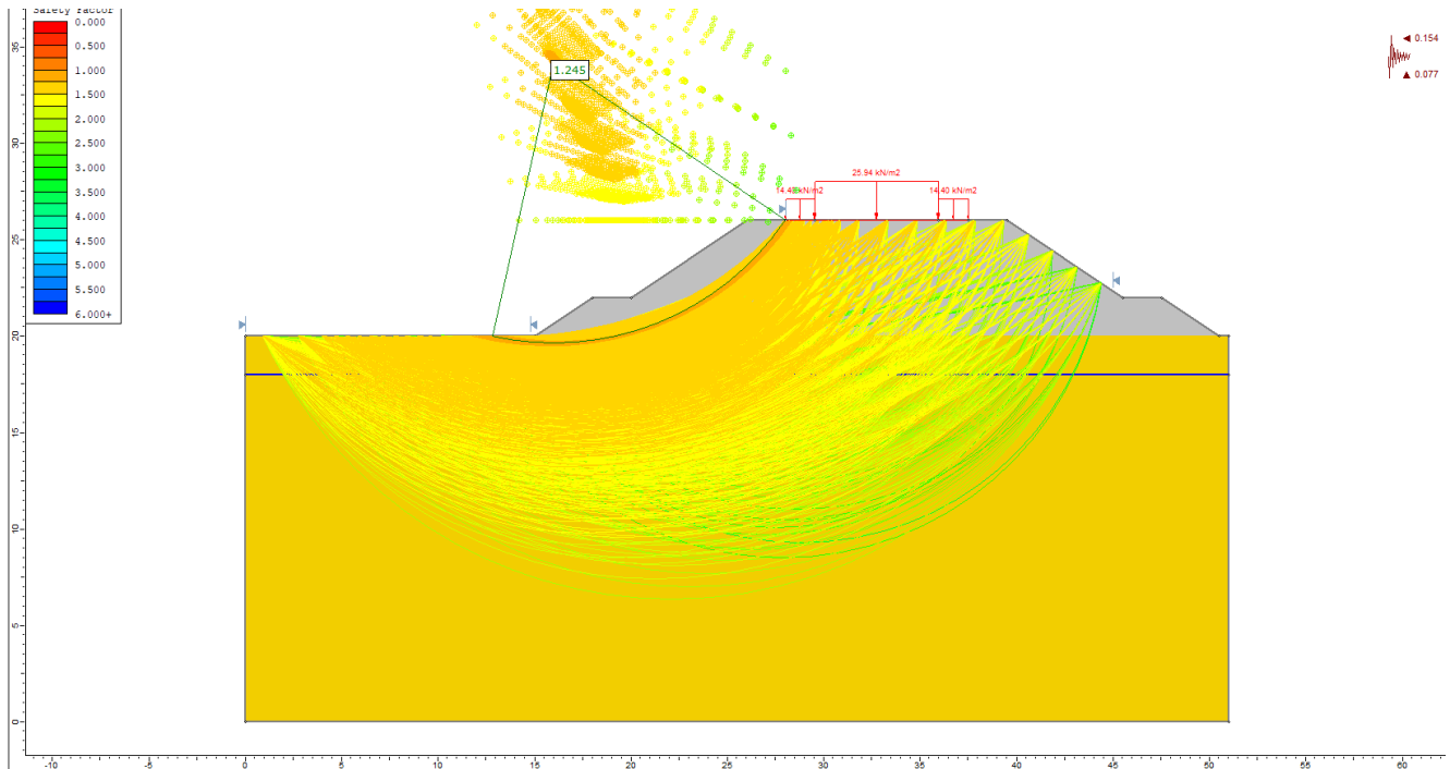
Figura 29 – Analisi di stabilità sismica doppio binario H=6m con banca (kv-)
