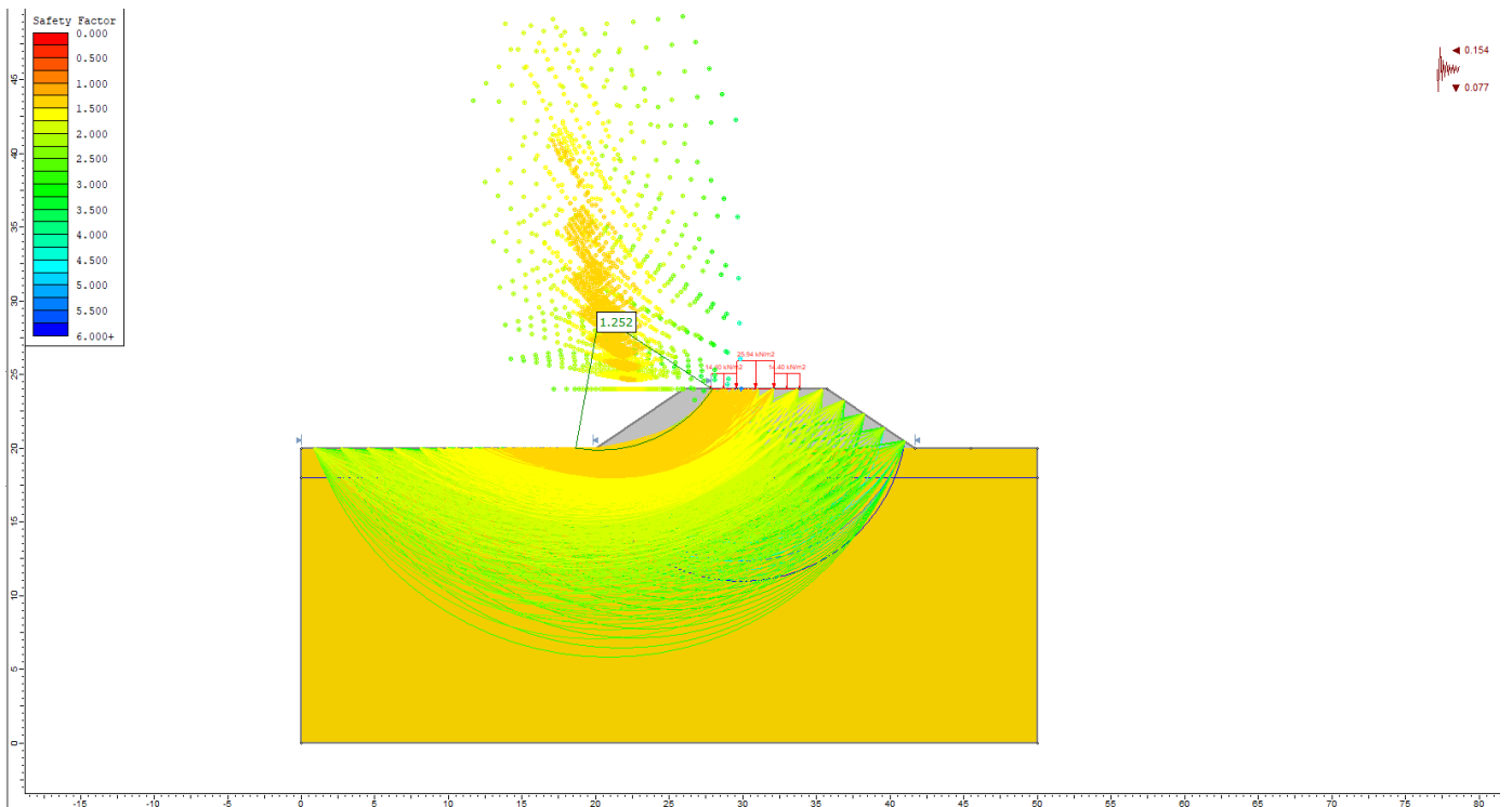
Figura 21 – Analisi di stabilità sismica singolo binario H=4m (kv+)
