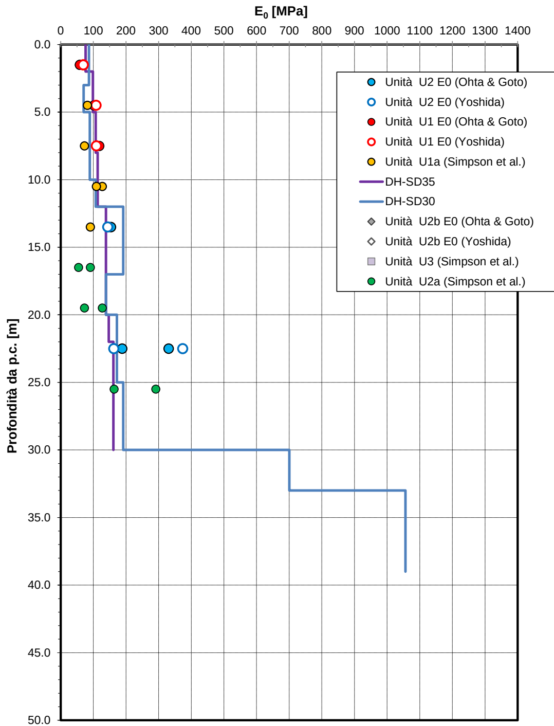
Figura 9 – Modulo di deformazione elastico a piccole deformazioni – RI06 sezione 60
