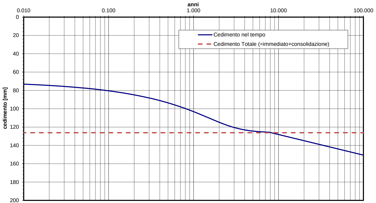
Figura 12 – Decorso dei cedimenti nel tempo – RI05 sez 29 km 1+450 – H=6m
