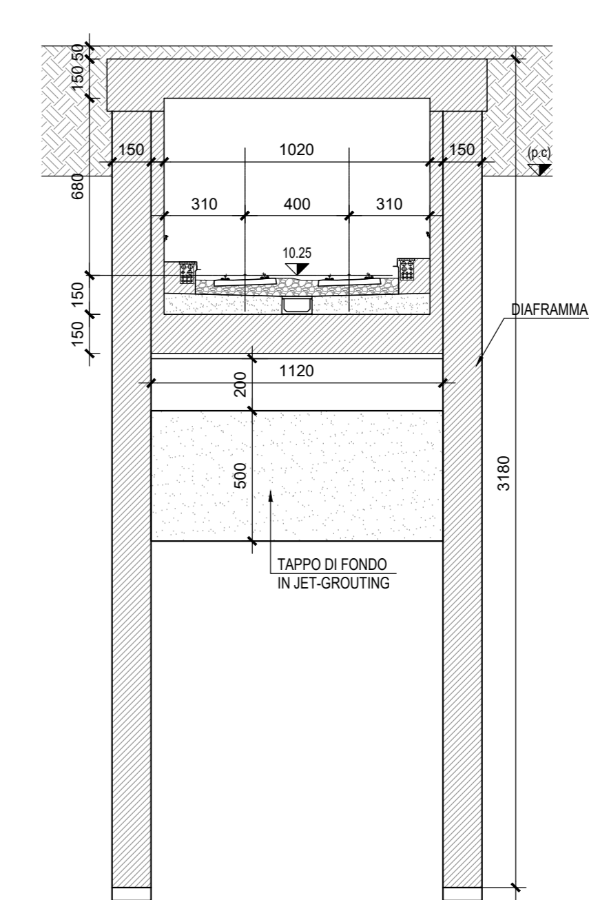
SEZIONE PK 1+000 - Scala 1:200
