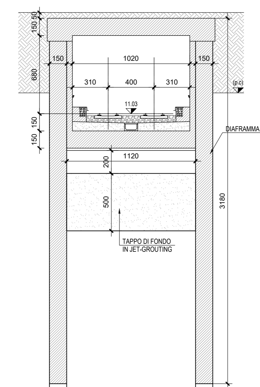
SEZIONE PK 0+922 - Scala 1:200
