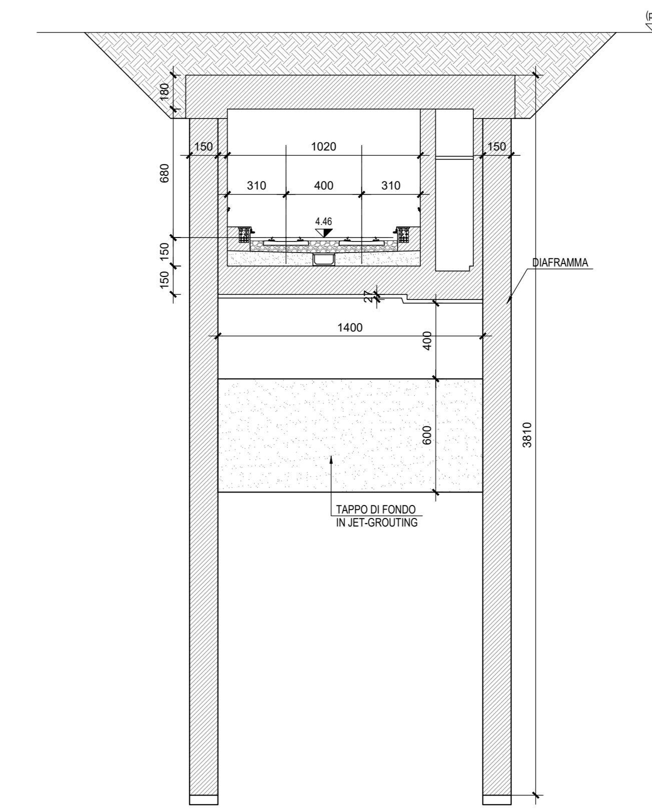
SEZIONE PK 1+600 - Scala 1:200
