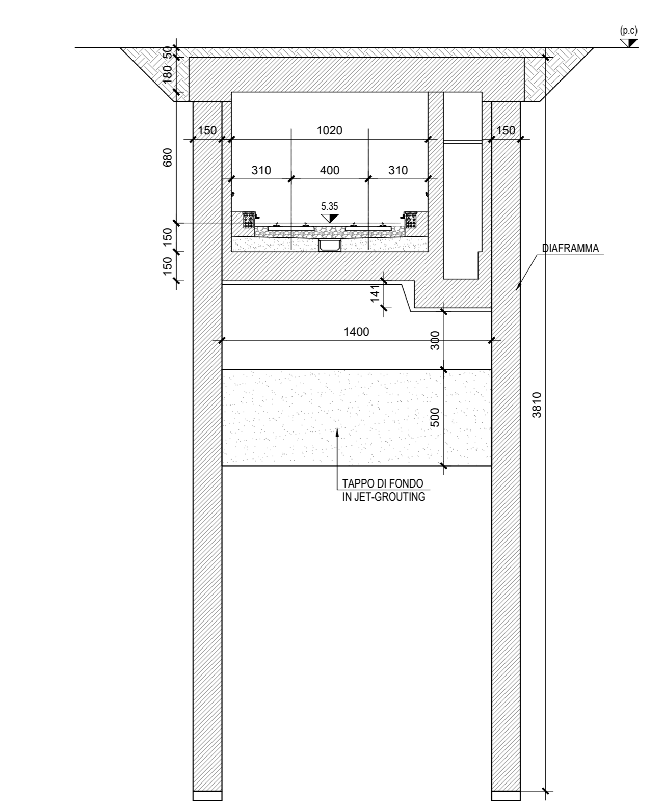
SEZIONE PK 1+700 - Scala 1:200
