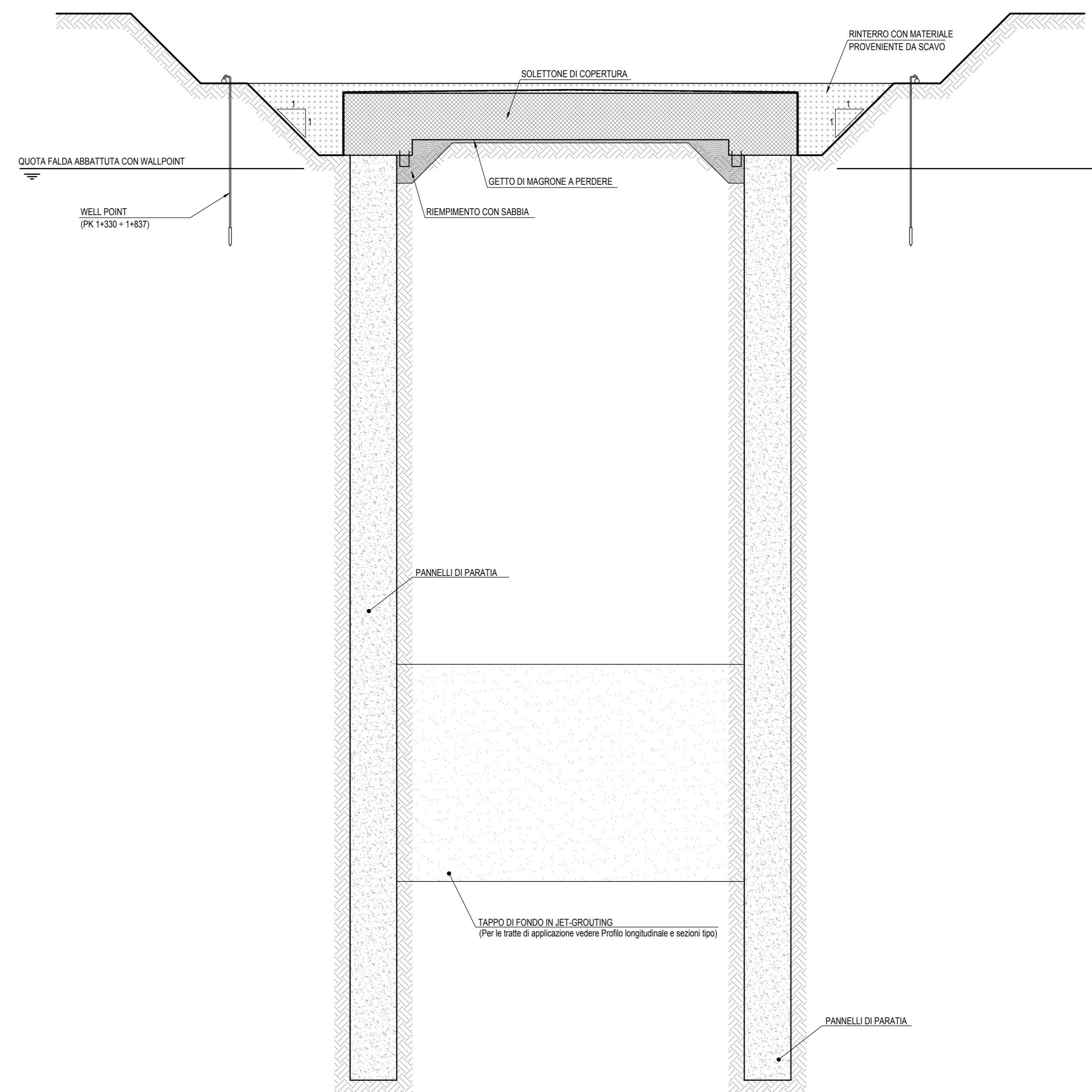
SEZIONE TIPO A e B - Fase 4 - scala 1:100
