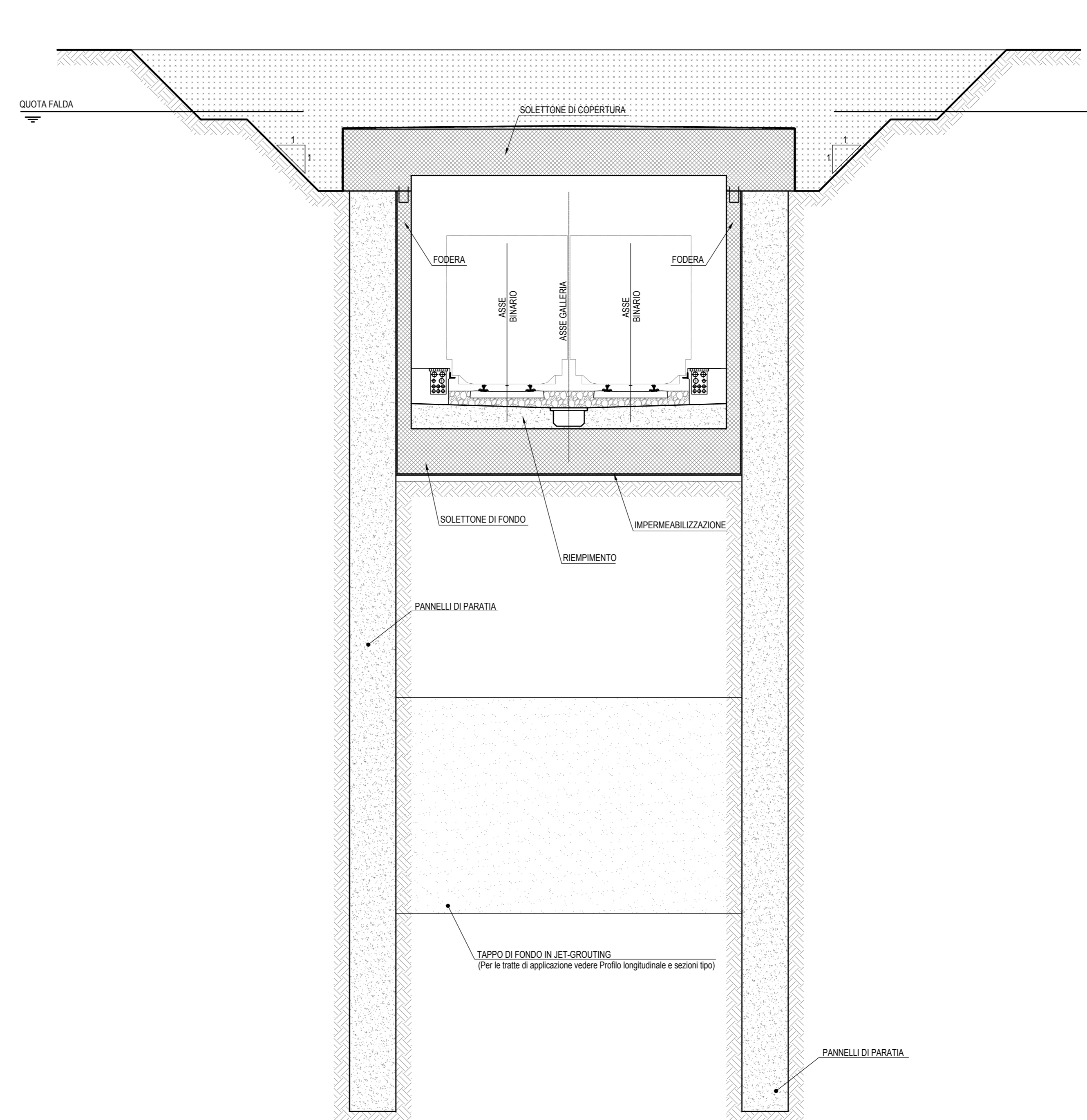
SEZIONE TIPO A e B - Fase 4 - scala 1:100
