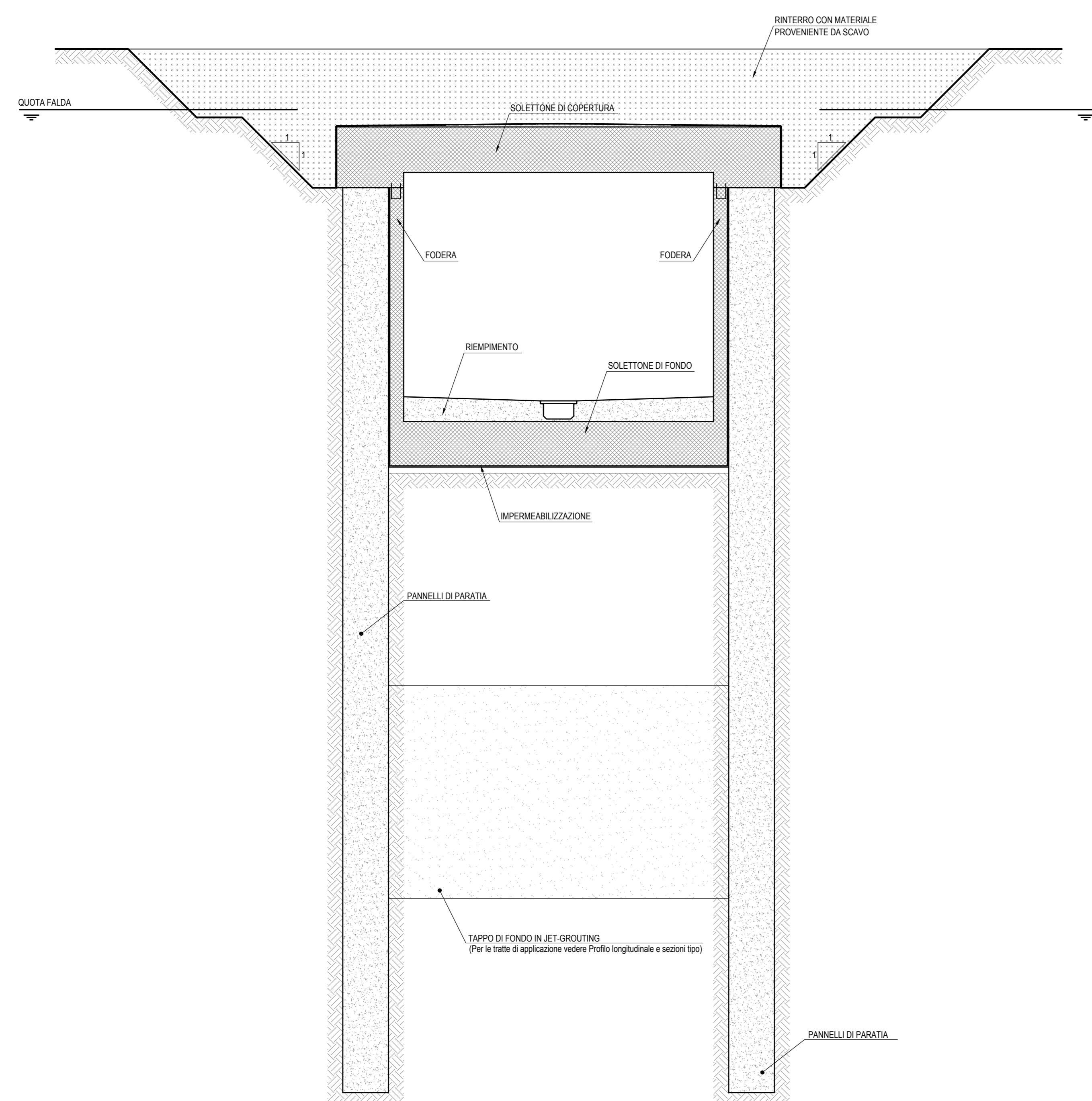
SEZIONE TIPO A e B - Fase 3 - scala 1:100
