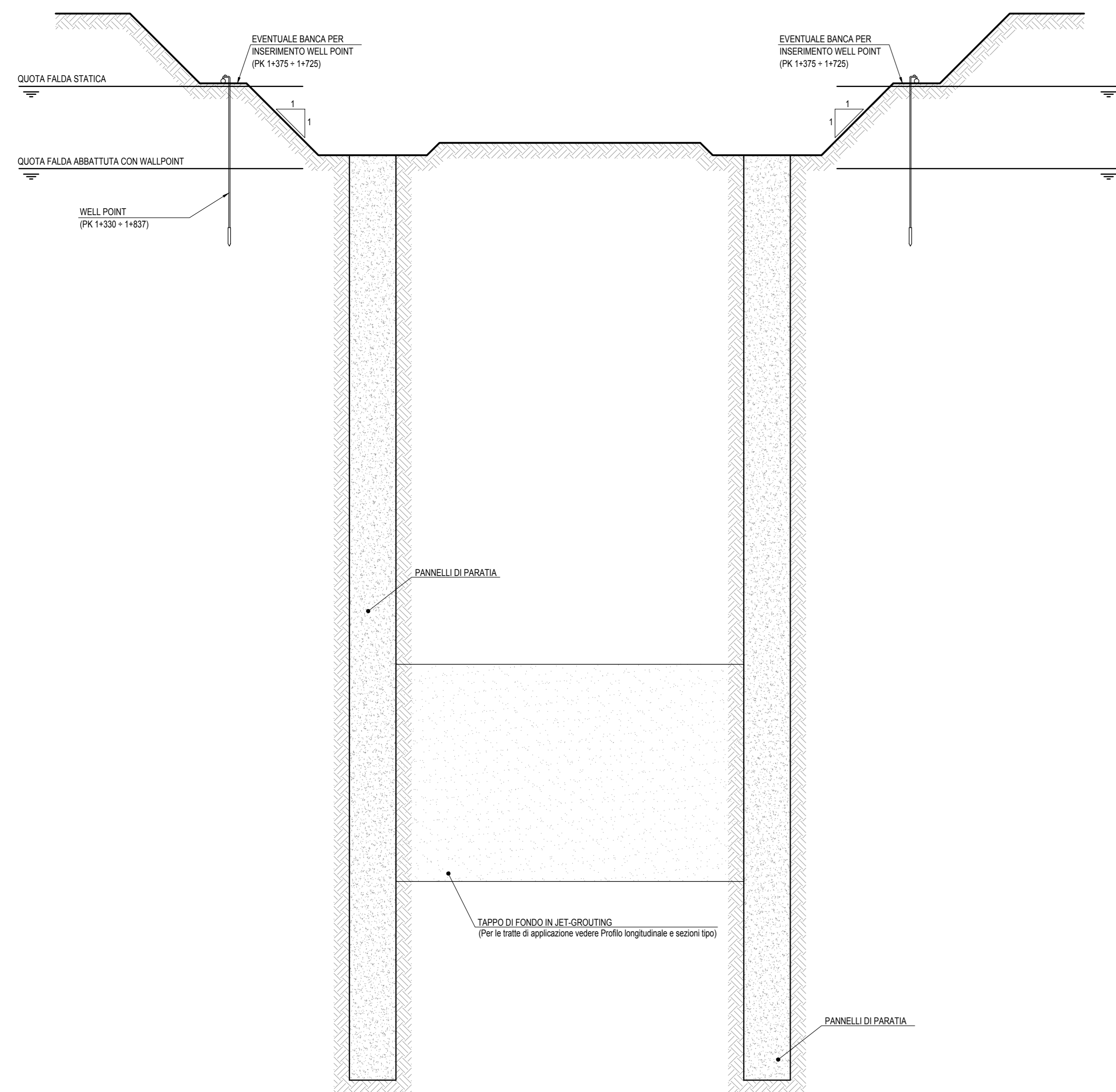
SEZIONE TIPO A e B - Fase 3 - scala 1:100
