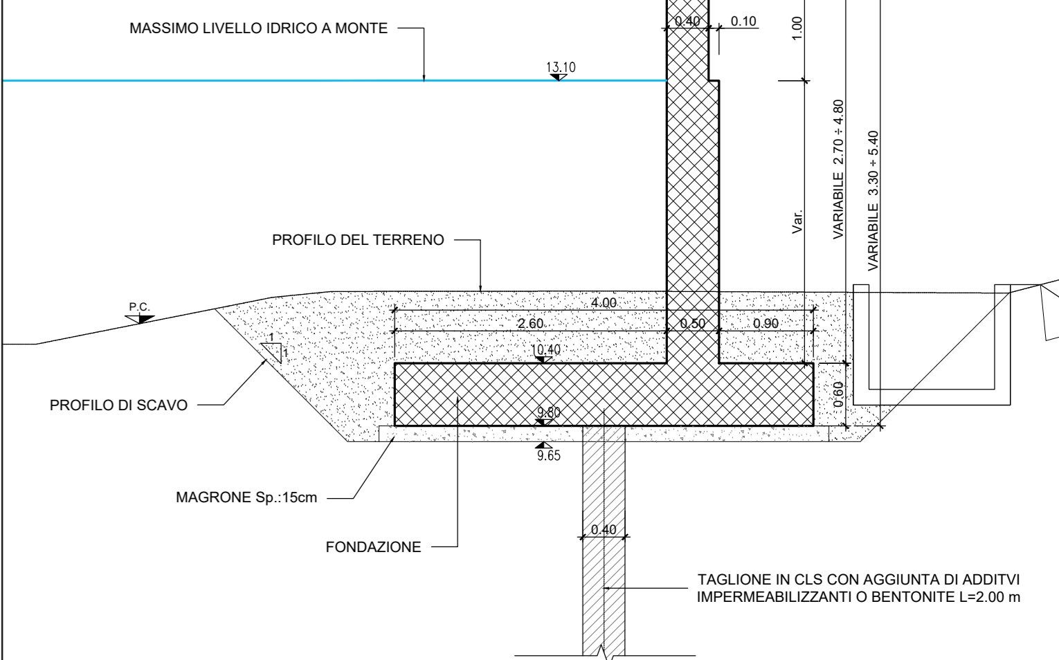
MURO TIPO 2 SEZIONE TRASVERSALE Muro di Protezione con Argine (Passaggio) da Km 2+504.45 a Km 2+701.60 Scala 1:50
