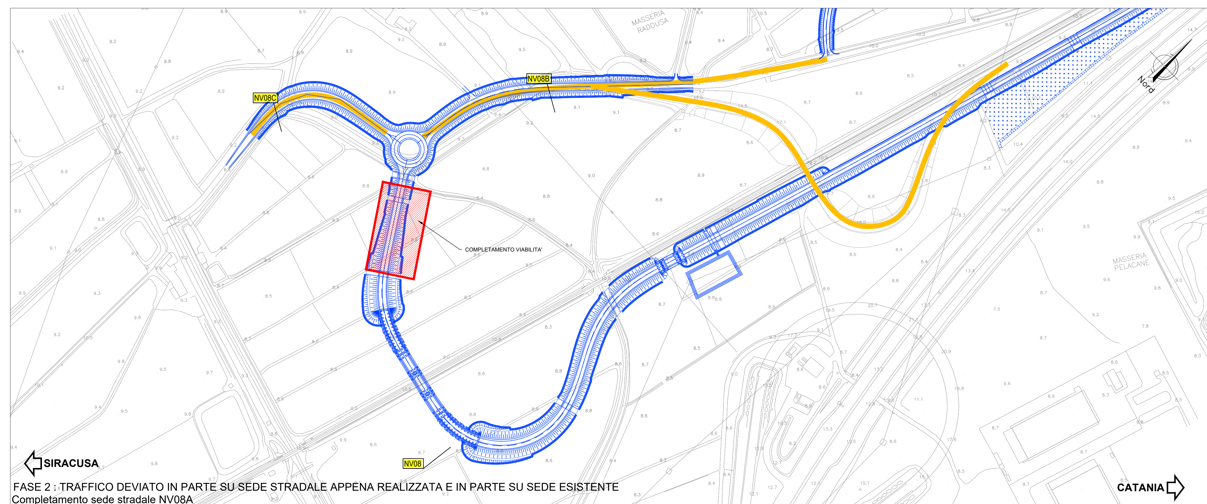
FASE 1 : TRAFFICO VEICOLARE SU SEDE ATTUALE Si realizza la nuova viabilità NV08 parzializzando il traffico dove interseca con la viabilità esistente
