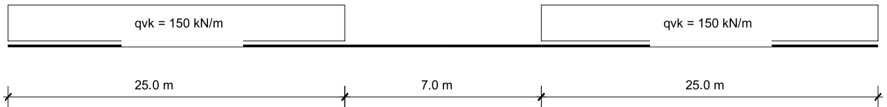
Figura 8. Treno SW/2
