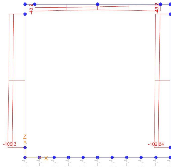
Sforzo normale
