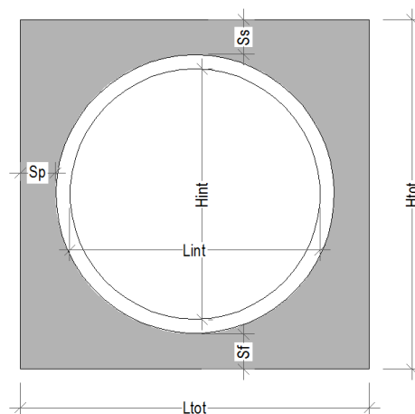
Figura 2. Sezione trasversale dello scatolare
