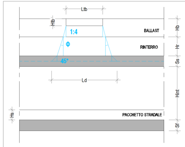
Figura 9. Schema modalità di diffusione dei carichi ferroviari
