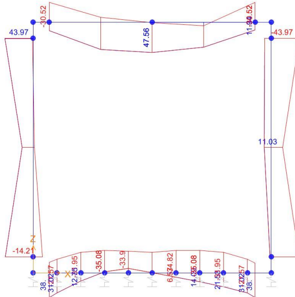
Momento Flettente
