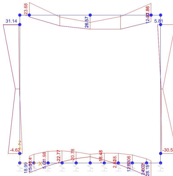
Momento Flettente
