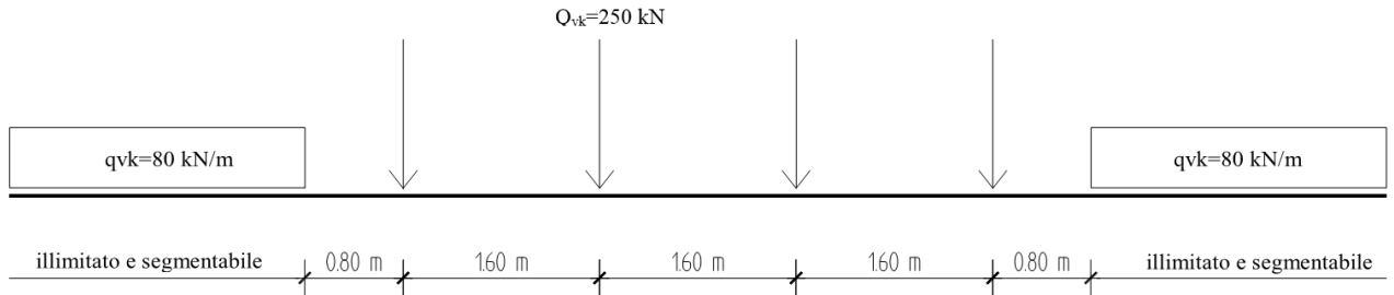
Figura 7. Treno LM71
